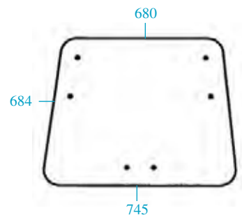
23/4072-73 (D9042, 5136410) Trasero (superior) 6 agujeros Upper rear - 6 holes
