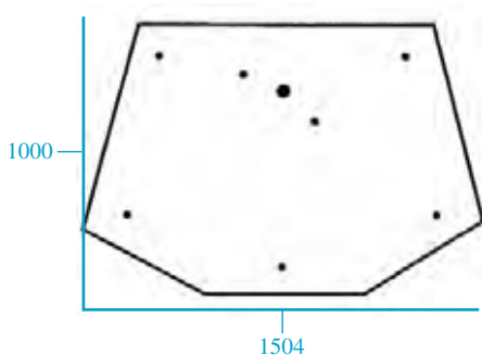
23/4071-28 (D6827, 86002901) Trasero - 8 agujeros Rear - 8 holes
