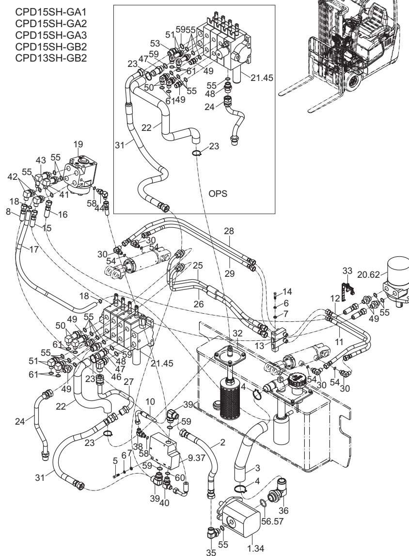
液壓管路系統(公制)/HYDRAULIC SYSTEM (METRIC)
