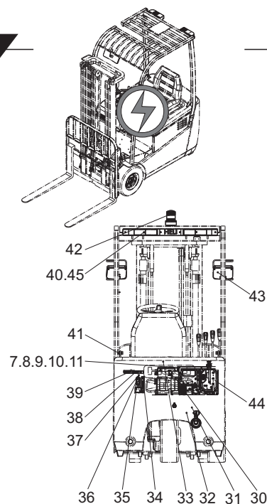
电气系统/ELECTRIC SYSTEM
