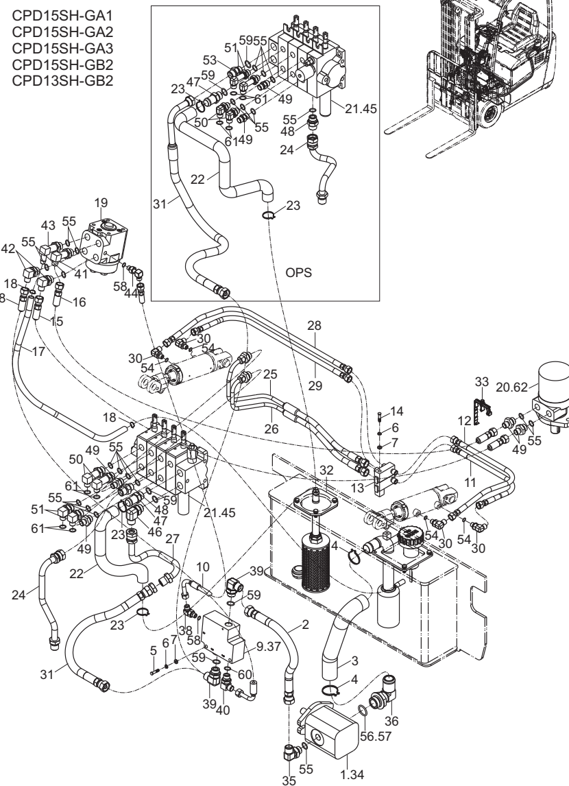
液压管路系统(公制)/HYDRAULIC SYSTEM(METRIC)
