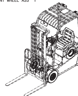
前轮总成 FRONT WHEEL ASS'Y
