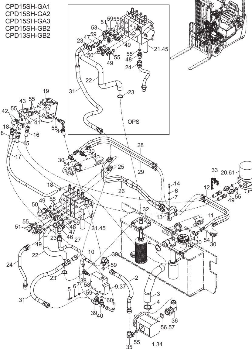
液压管路系统(美制)/HYDRAULIC SYSTEM(SAE)
