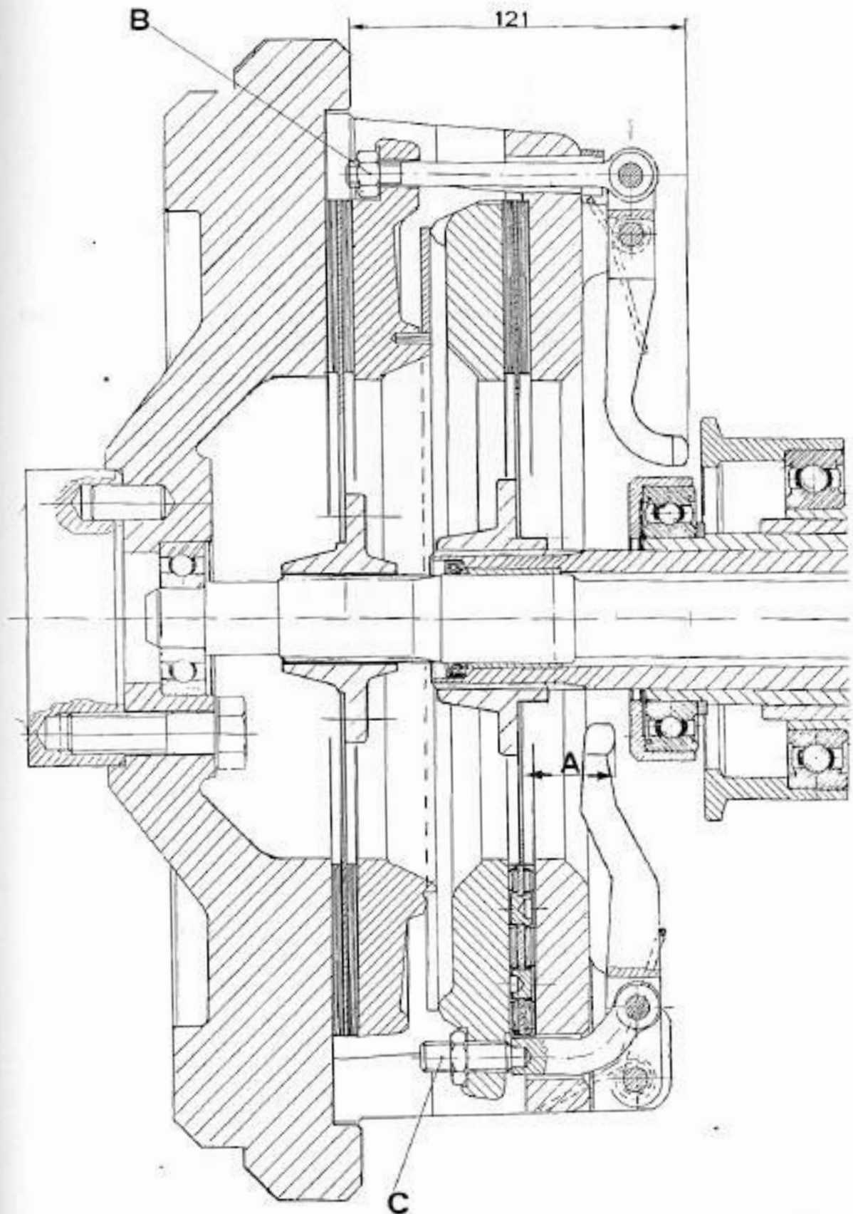
FIG. 55/B - Embrayage Luk pour tracteurs R 704 - R 804
