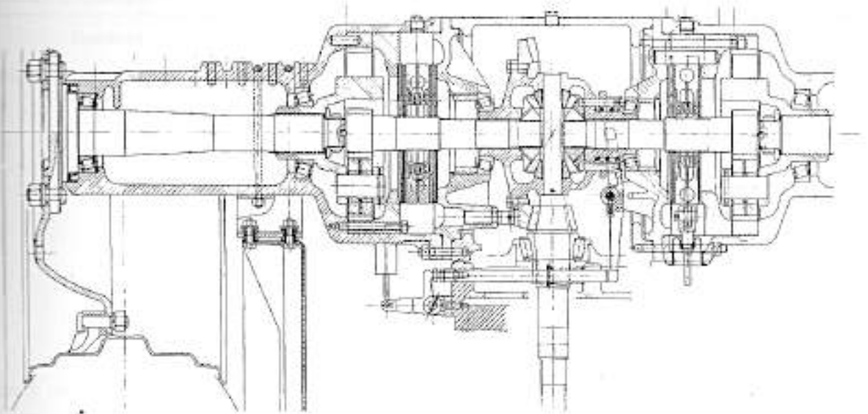
FIG. 58 - Coupe transversale arrière des tracteurs R 704 - R 804
