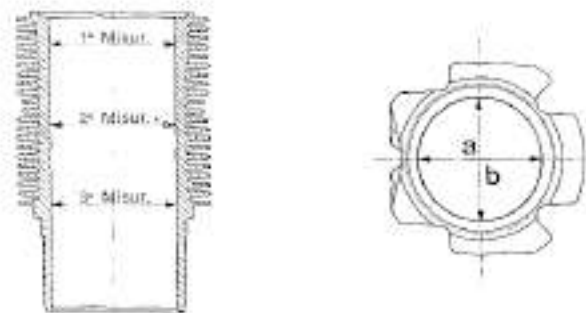
FIG. 10 - Schéma pour le contrôle des cylindres
