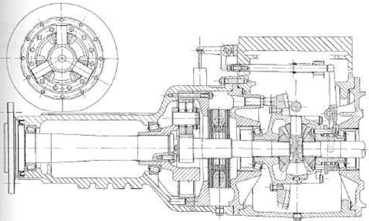
FIG. 58 - Coupe transversale arrière des tracteurs * R 904
