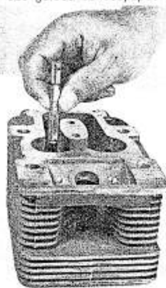
FIG. 24 - Contrôle des sièges sur la culasse
