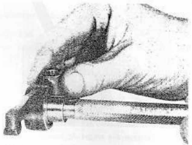
FIG. 28 - Contrôle du diamètre intérieur des culbuteurs
