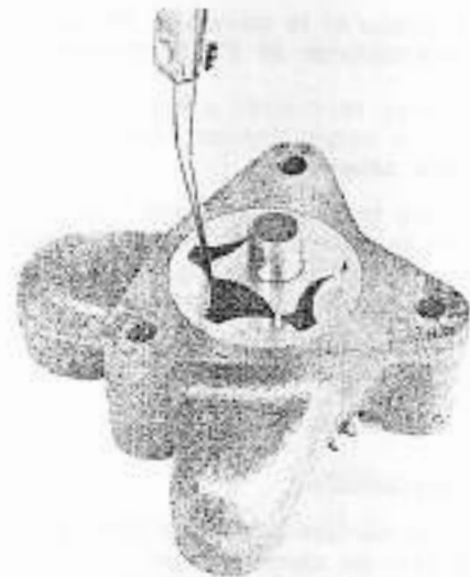
FIG. 29 - Contrôle du jeu entre les rotors de la pompe à huile
