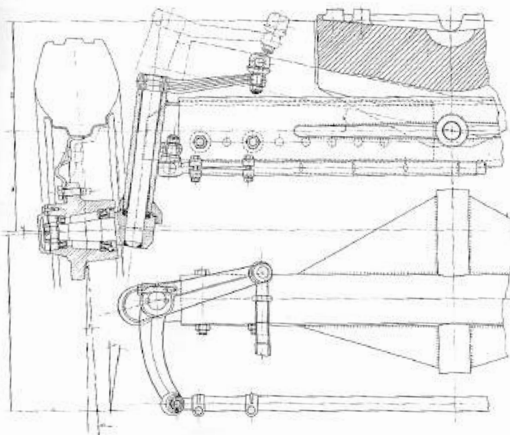
FIG. 61 - Essieu avant
