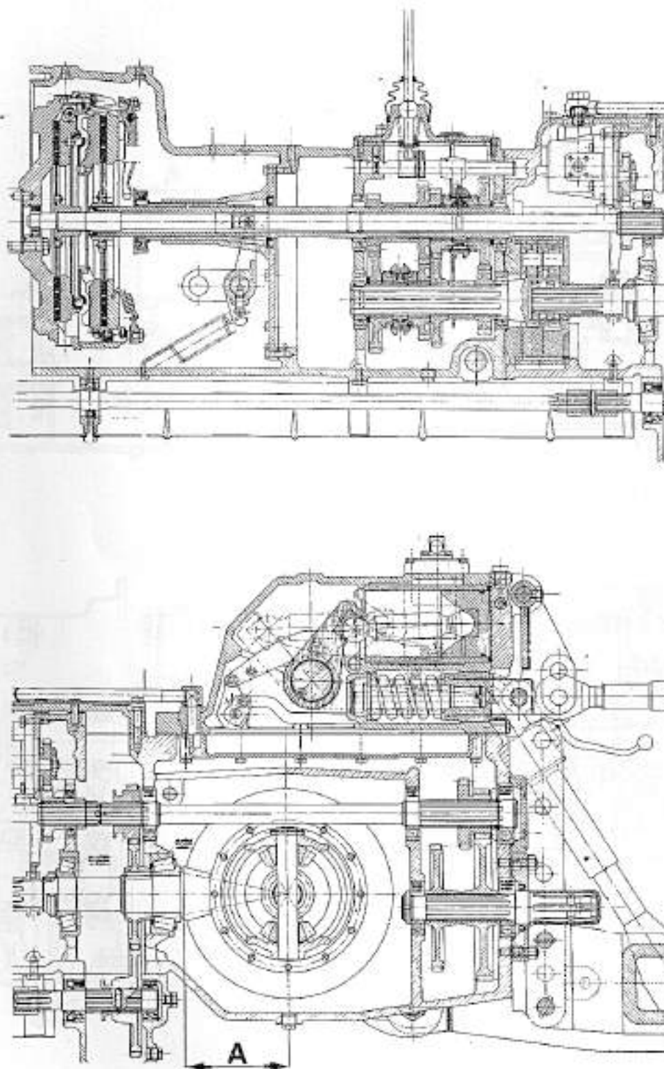
FIG. 57 - Coupe longitudinale avant et arrière de la boîte de vitesses des tracteurs R 704 R 804 - R 904
