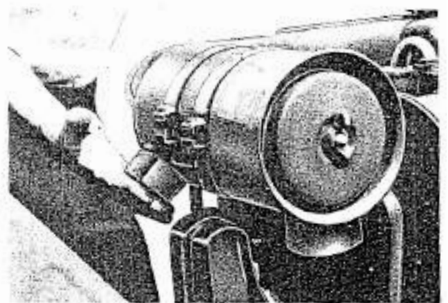
FIG. 38 - Fermeture du tuyau d'aspiration
