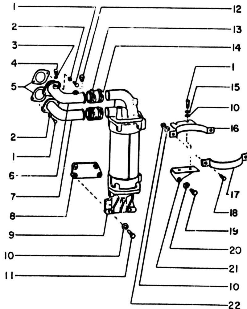
TRANSMISSION HEAT EXCHANGER COOLANT PIPING - TUBULAÇÃO DO INTERCAMBIADOR DA TRANSMISSÃO
