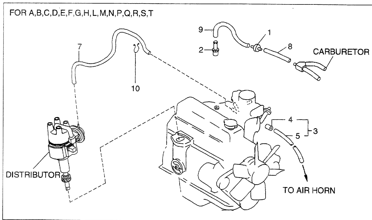
FIG. 49 VACUUM CONTROL SYSTEM バキュームコントロールシステム
