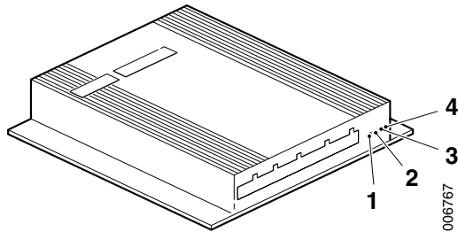
Lámparas testigo de unidad de mando de la cabina
