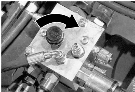
Cierre la válvula de carga de acumuladores
