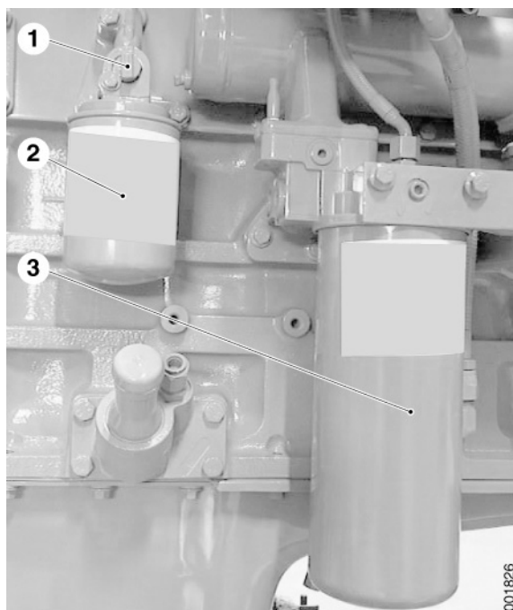
Filtro en lado izquierdo, opción de motor Cummins
