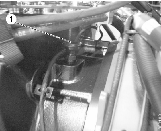
1. Filtro de respiración, en parte superior del convertidor de par.
