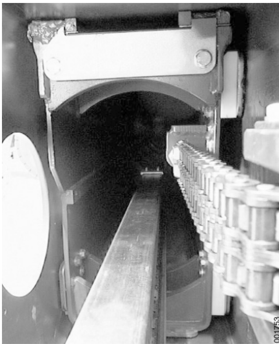
La figura muestra las placas deslizantes interiores en la viga principal del implemento.
