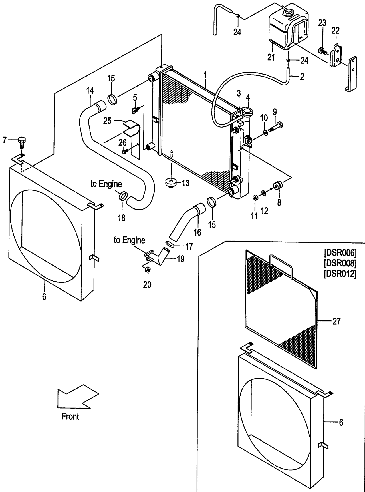
FIG.6 COOLING UNIT (F6042120) クーリングユニット
