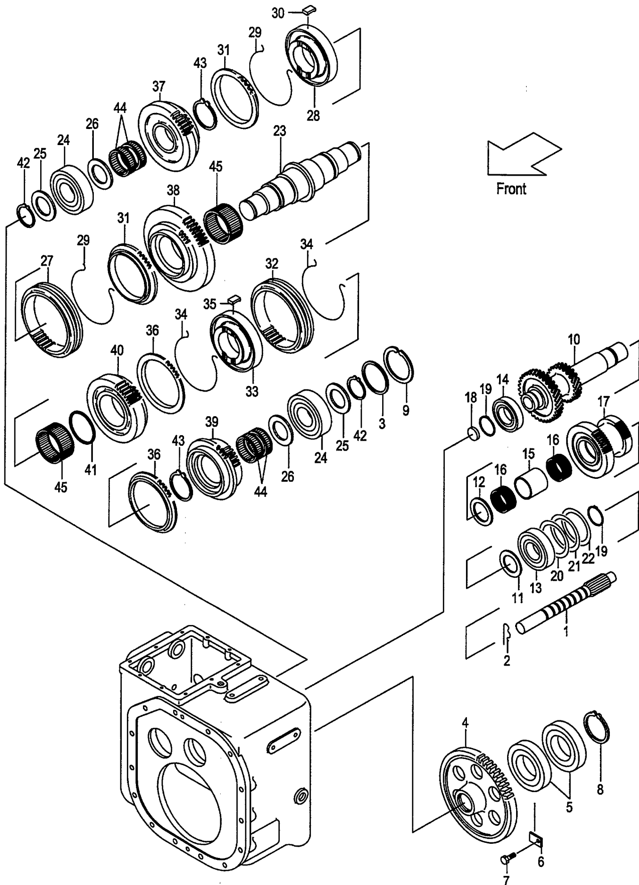
FIG.25 DRIVE UNIT (3/3)(CLUTCH) (F6042550) ドライブユニット
