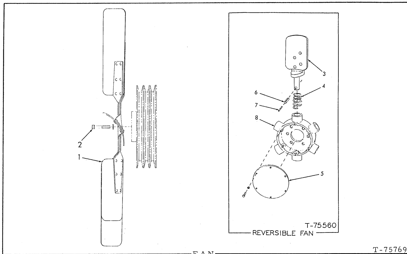
FAN
