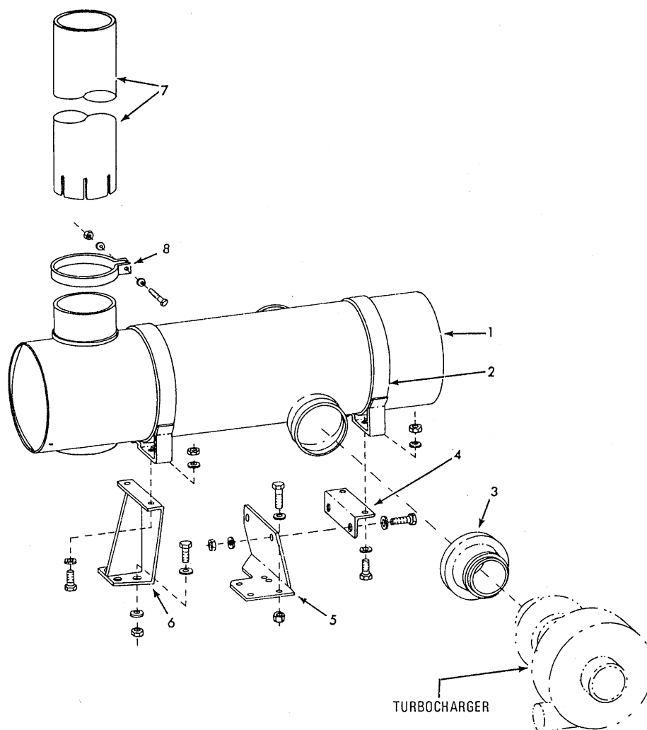
MUFFLER
