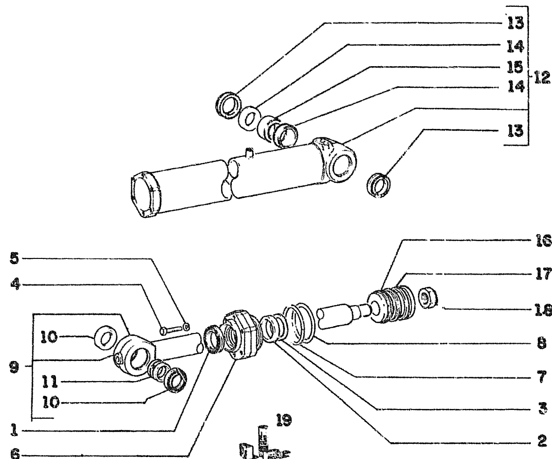
RIPPER CYLINDER - CILINDRO DO RIPER
