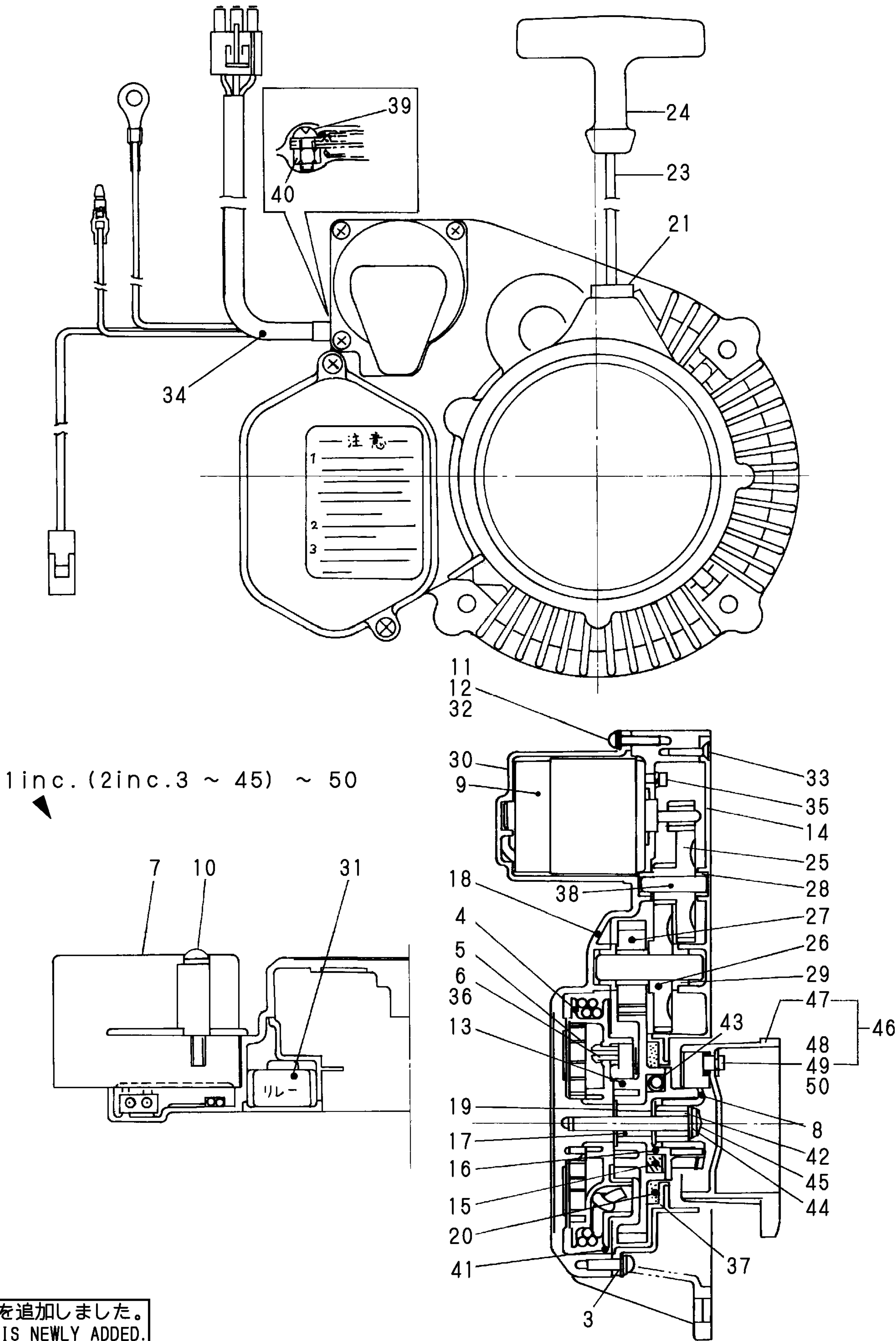
Fig. 9 セルリコスタータインナーパーツ SEL - REC STARTER COMPONENT PART
