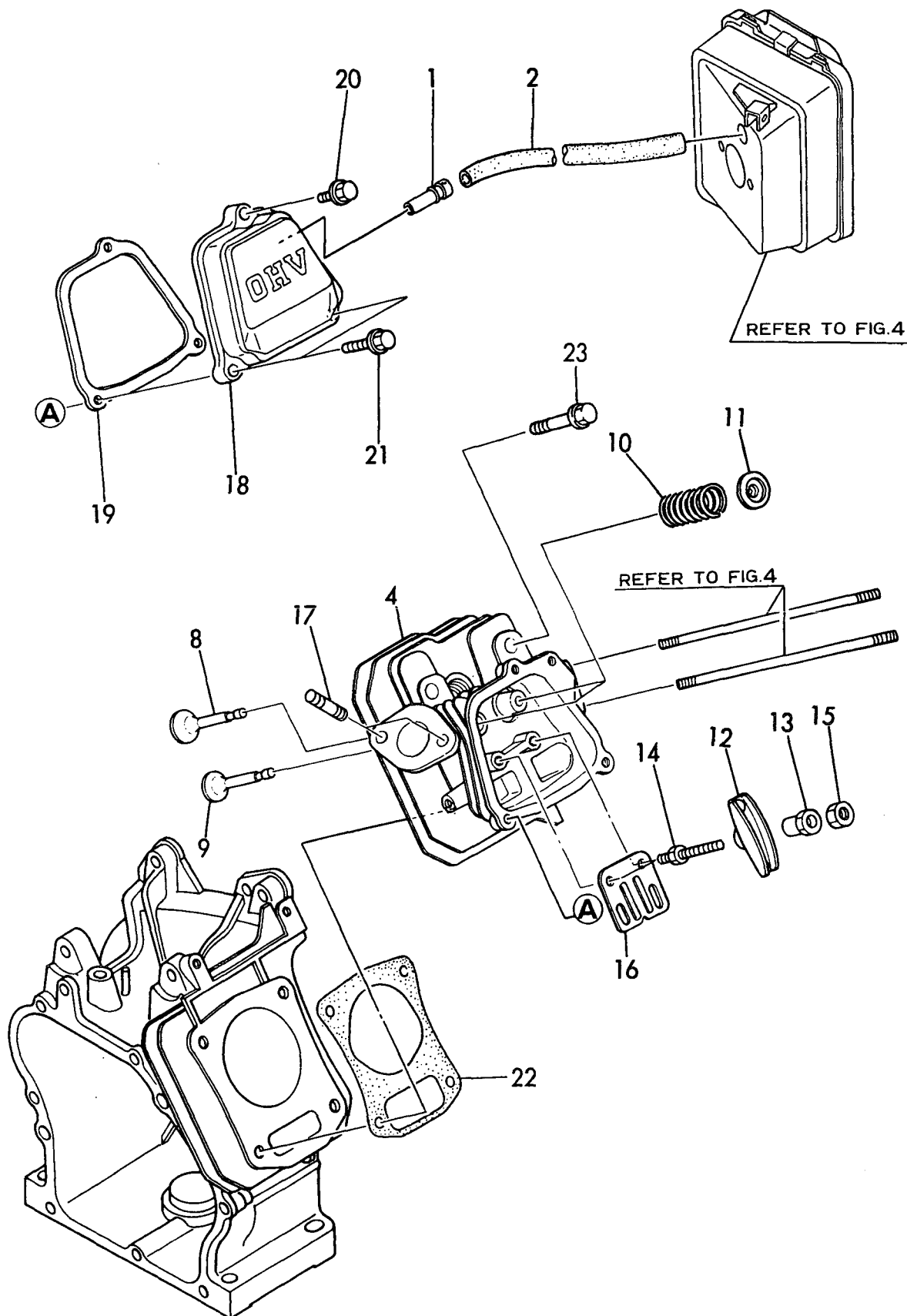
Fig. 2 シリンダヘッド&ボンネット CYLINDER HEAD & BONNET
