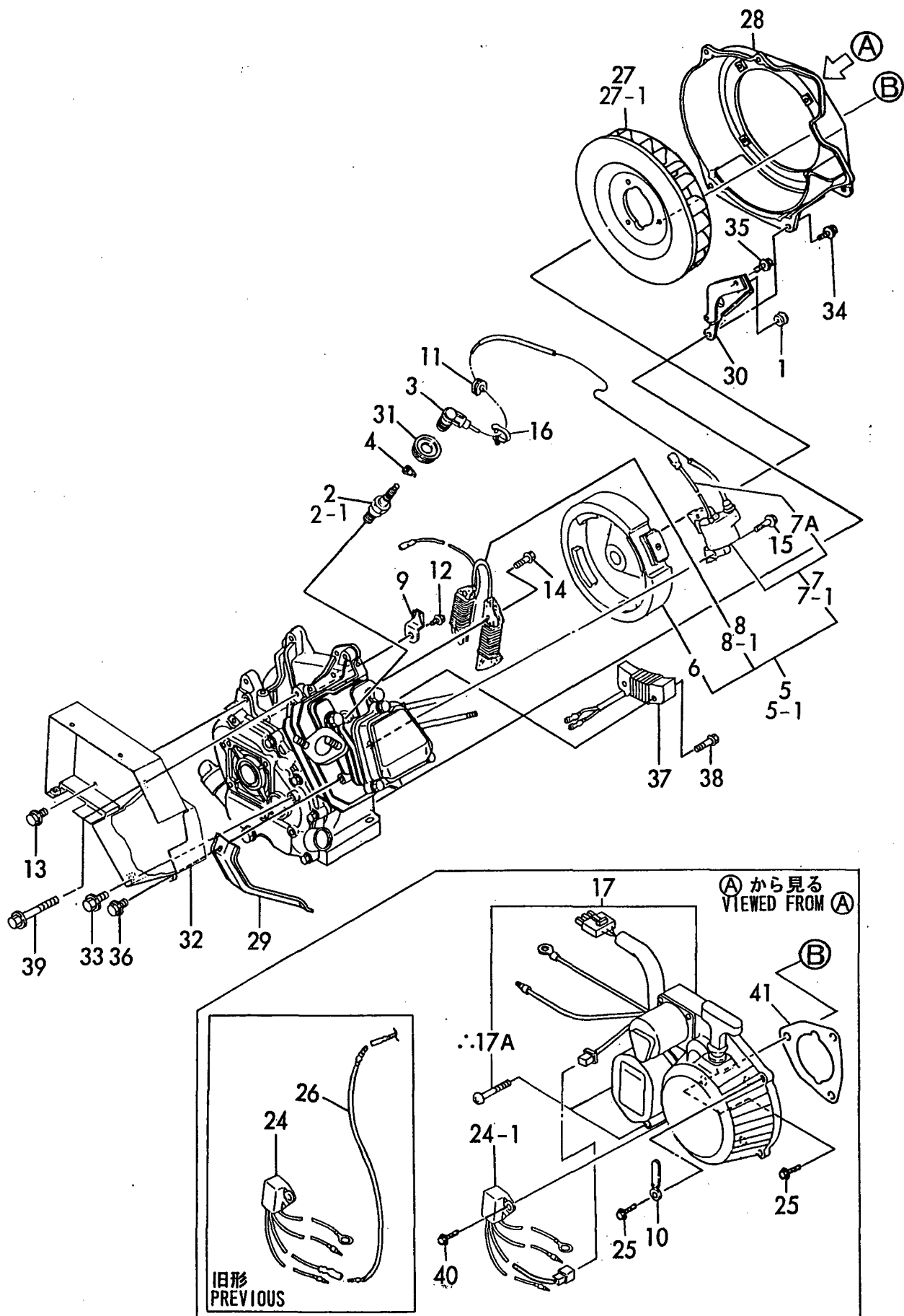
Fig. 8 フライホイールマグネット&始動装置 FLY. MAGNETO & STARTING DEVICE
