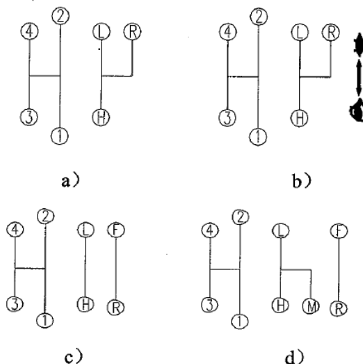
Figuur 2-24 versnelling combinaties voor de TB series
