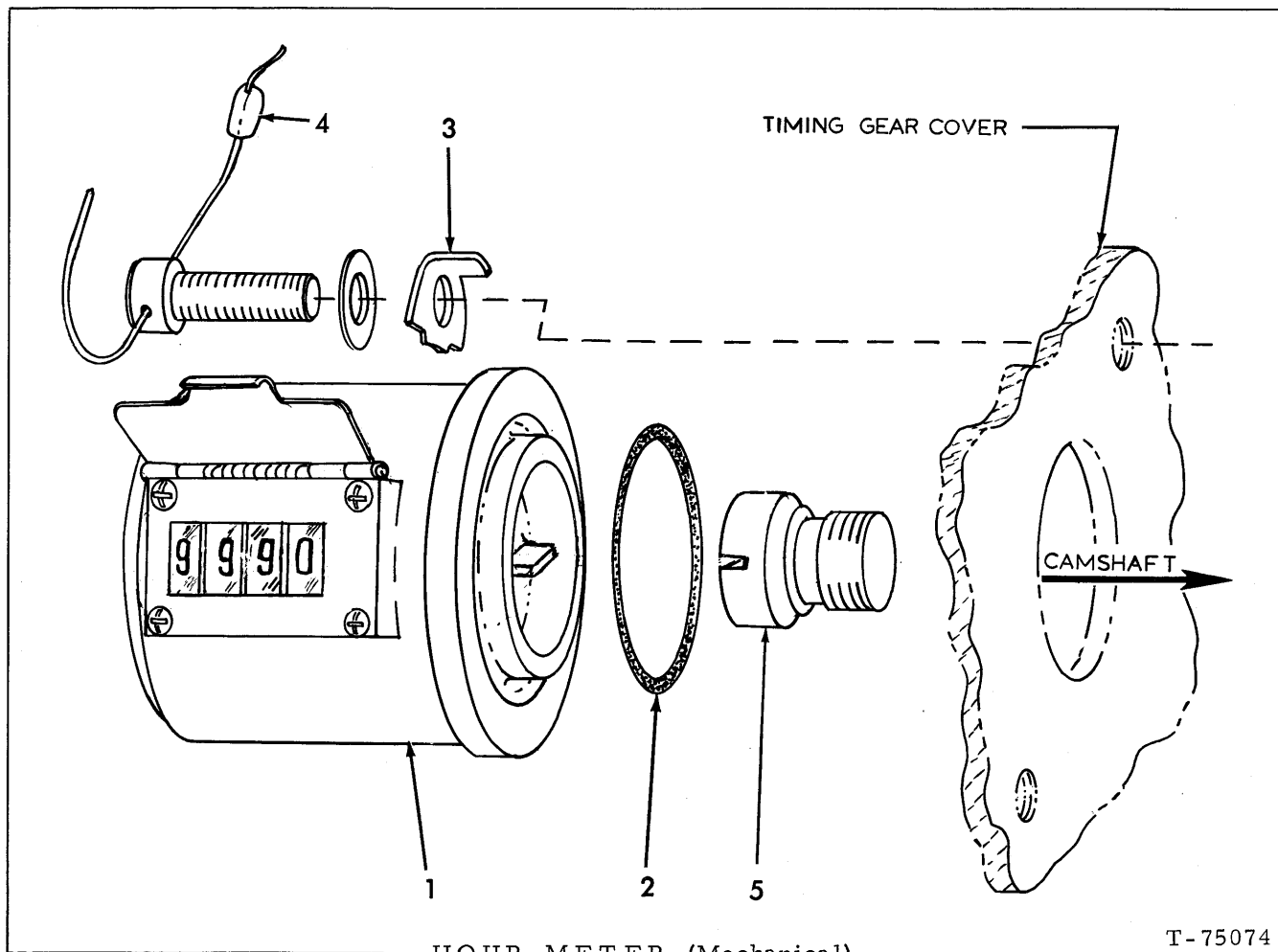
HOUR METER (Mechanical)
