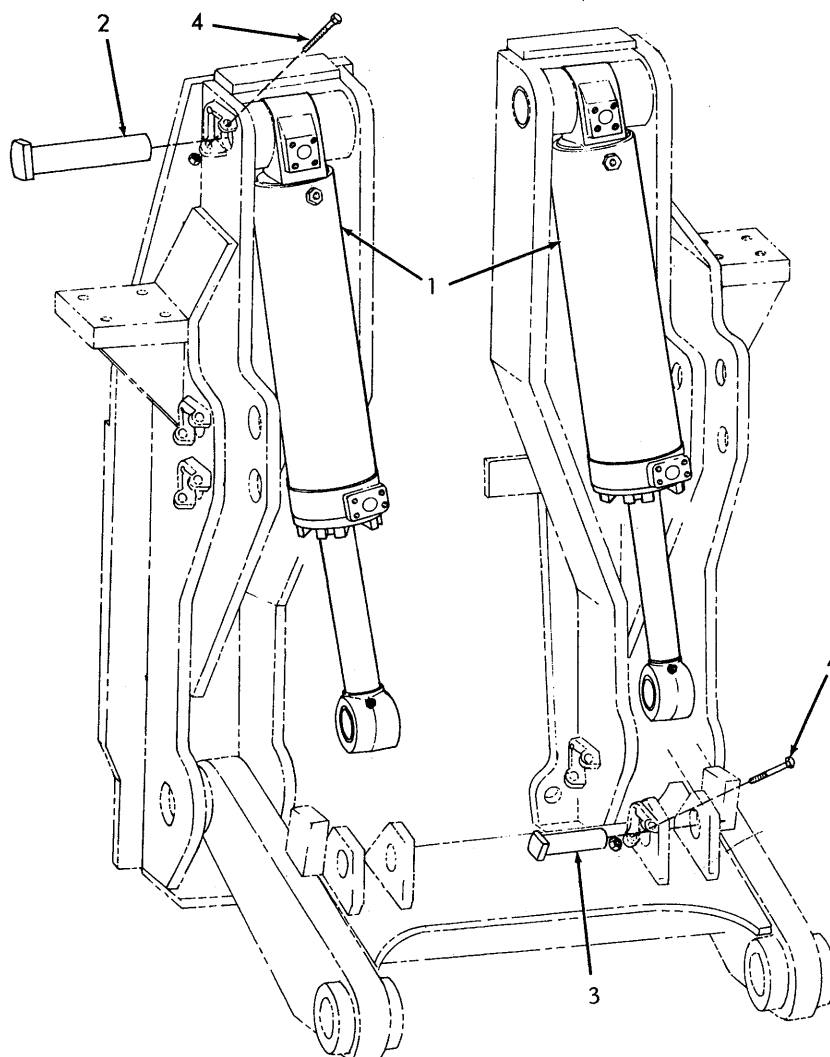
R I P P E R C Y L I N D E R M O U N T I N G
