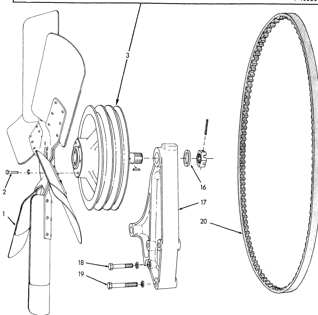
FAN PULLEY
