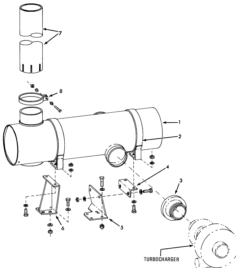
MUFFLER
