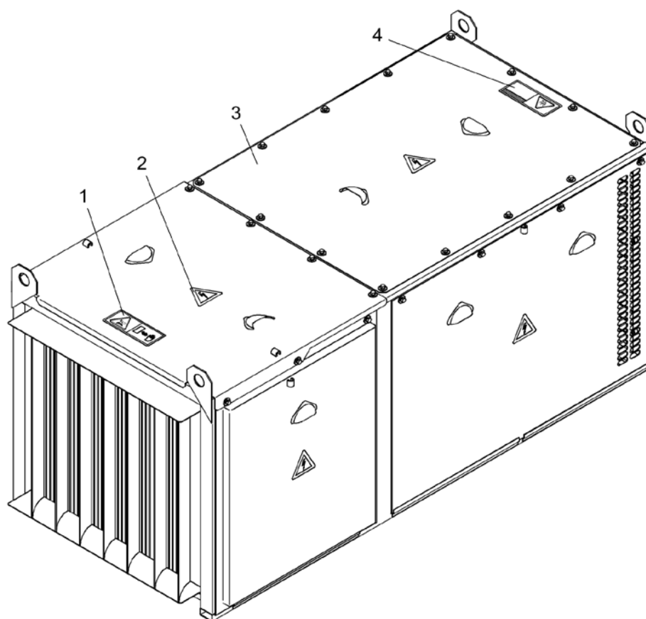
Рисунок 2.5.7 – Вентилируемая тормозная установка в сборе (75139-2126002, 75139-2126002-01) Figure 2.5.7 – Vented brake unit
