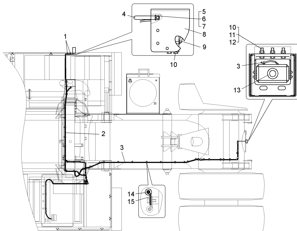
Рисунок 2.17.1 – Установка системы видеонаблюдения по шасси (75131-7912002, 75131-7912002-01, 75131-7912002-02)
