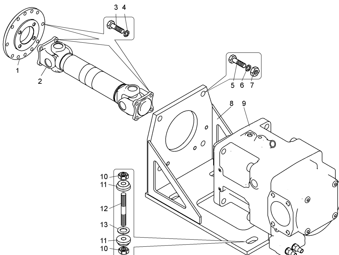
Рисунок 2.19.14 – Установка насоса и карданного вала (75131-8600032-20)
