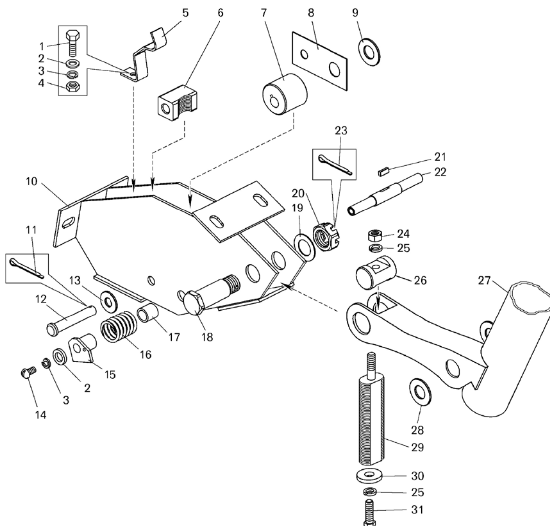
Рисунок 2.10.4 – Колонка рулевая с кронштейном (75474-3444009) Figure 2.10.4 – Steering column with bracket
