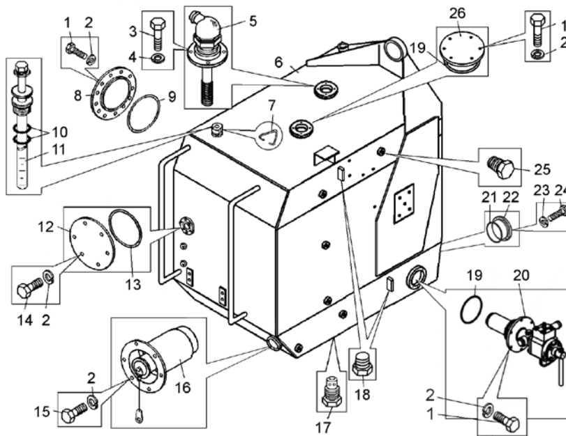
Рисунок 2.2.3 – Бак топливный (с системой заправки «Wiggins»), (75131-1101010-41) Figure 2.2.3 – Fuel tank (with refilling system of “Wiggins”)
