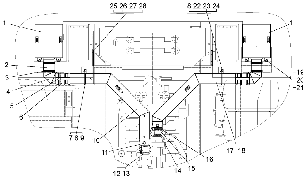
Рисунок 2.2.6 – Установка воздушных фильтров" (75131-1100005) Figure 2.2.6 – Mounting of air filters
