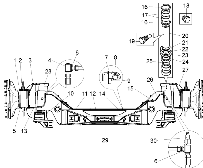
Рисунок 2.9.1 – Ось передняя с тормозами (75131-3000012) Figure 2.9.1 – Front axle with brakes
