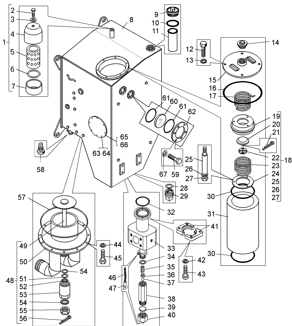
Рисунок 2.19.18 – Бак масляный (75131-8608008-20)
