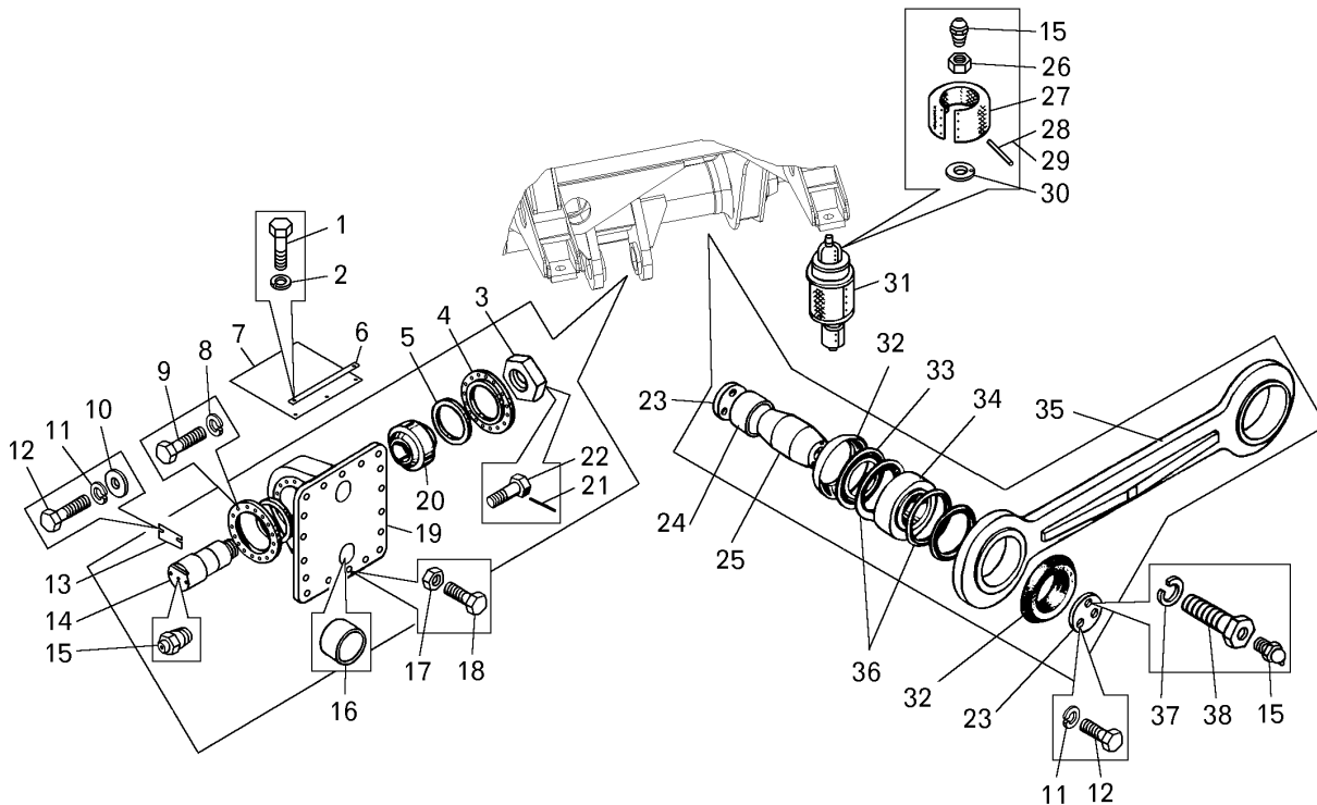
Рисунок 2.8.2 – Установка задней подвески (75131-2900002-40)
