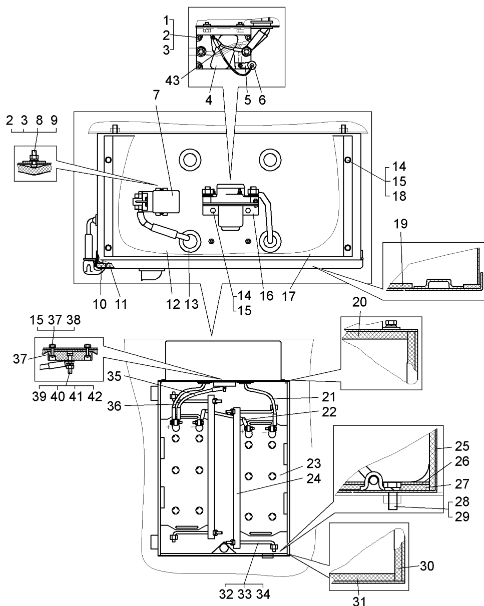
Рисунок 2.13.6 – Установка аккумуляторных батарей и монтаж проводов (75131-3700008-31) Figure 2.13.6 – Installation of storage batteries and cables montage
