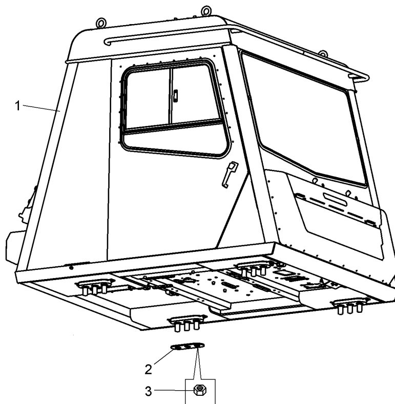
Рисунок 2.16.1 – Установка кабины на шасси (75306-5000002-30)
