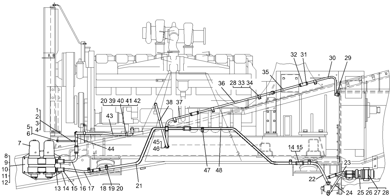
Рисунок 2.2.11 – Топливные трубопроводы с фильтрами "Flitguard" (75131-1100006-30)
