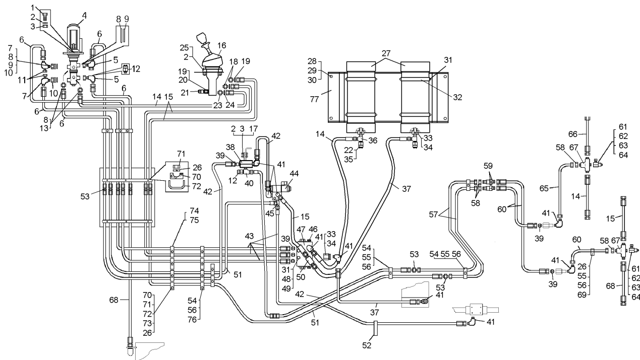
Рисунок 2.11.1 – Монтаж гидравлического привода тормозов (75131-3500003-40) Figure 2.11.1 – Mounting of hydraulic brake drive
