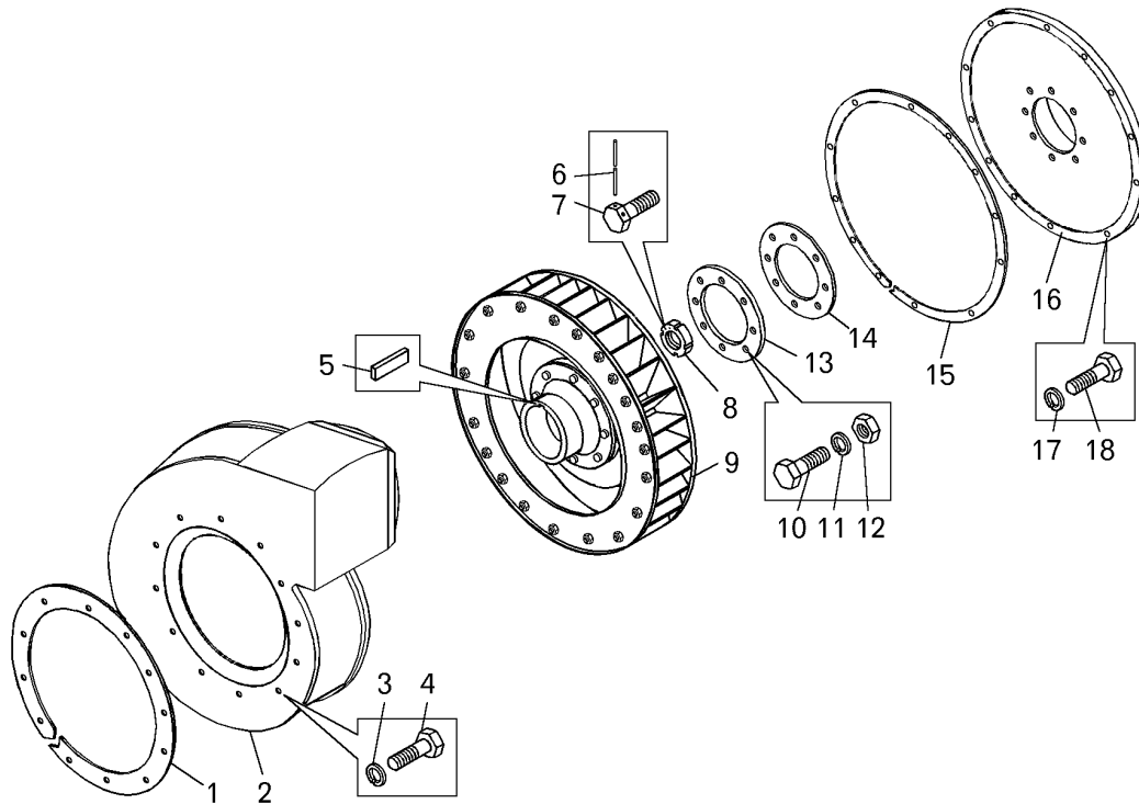
Рисунок 2.5.11 – Установка вентилятора охлаждения тяговых электромашин (75131-2100040) Figure 2.5.11 – Mounting of fan of haul electrical units cooling
