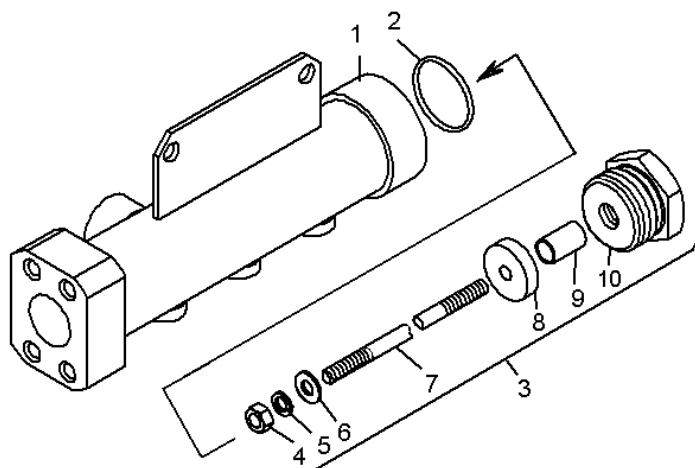
Рисунок 2.19.10 – Коллектор сливной (75306-8609320) Figure 2.19.10 – Drain collector
