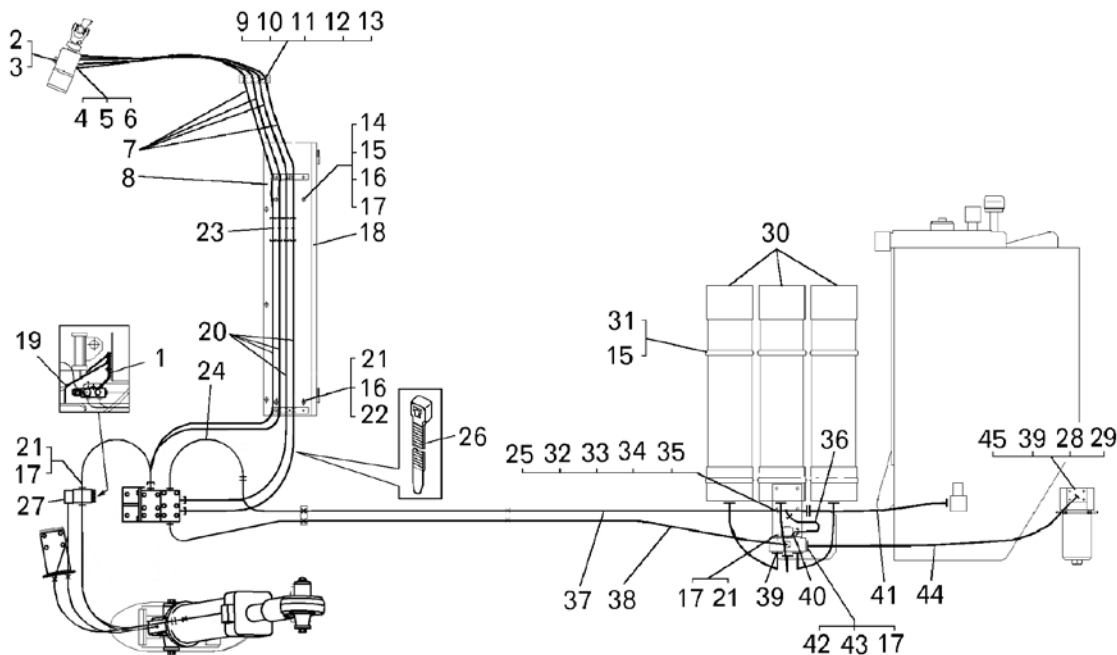
Рисунок 2.10.13 – Трубопроводы рулевого управления (вид I), (75137-3400001-31) Figure 2.10.13 – Steering pipelines (view I)
