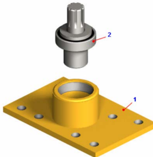
Рисунок 2.10.2 – Фланец с подшипником (75474-3401259) Figure 2.10.2 – Flange with bearing
