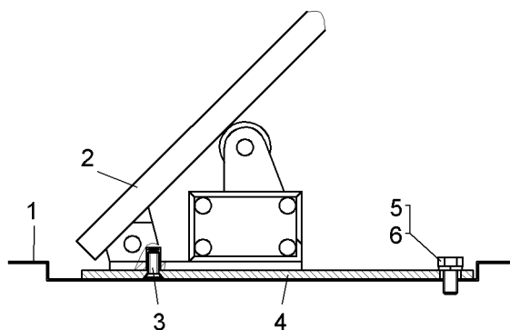
Рисунок 2.5.14 – Установка тормозной педали (75307-2100080-10)
