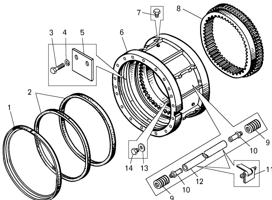
Рисунок 2.6.8 – Ступица электромотор-колеса (75132-3104006-10) Figure 2.6.8 – Electromotor-wheel hub
