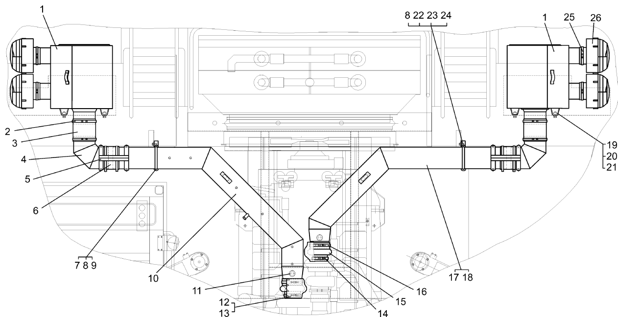
Рисунок 2.2.7 – Установка воздушных фильтров с системой очистки "Flitguard" (7513-1100005-10) Figure 2.2.7 – Mounting of air filters with cleaning system "Flitguard"
