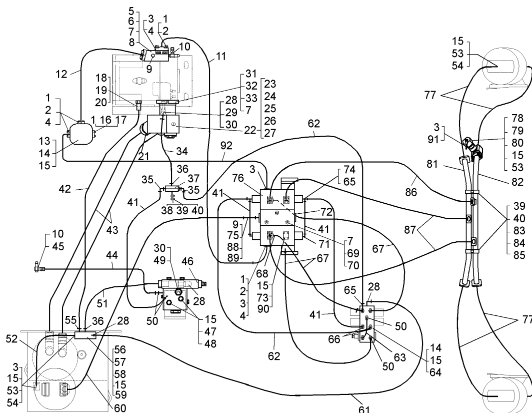
Рисунок 2.19.3 – Трубопроводы опрокидывающего механизма (75131-8600005-40) Figure 2.19.3 – Dumping mechanism pipelines
