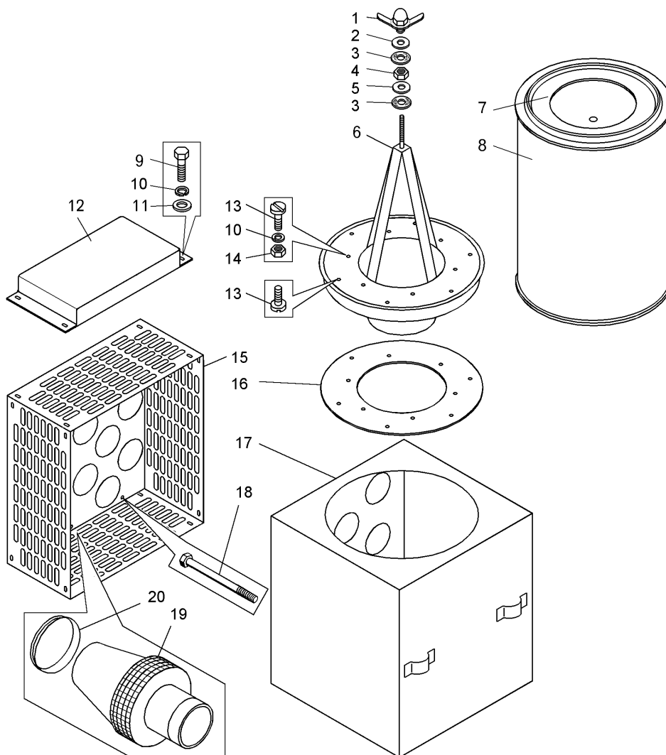
Рисунок 2.2.8 – Фильтр воздушный (75131-1109010) Figure 2.2.8 – Air filter
