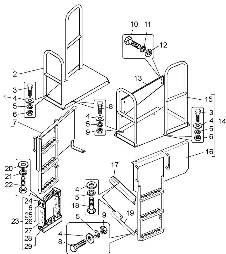
Рисунок 2.16.14 – Установка площадок моторного отсека (75131-8012003) Figure 2.16.14 – Mounting of sites of the engine compartment
