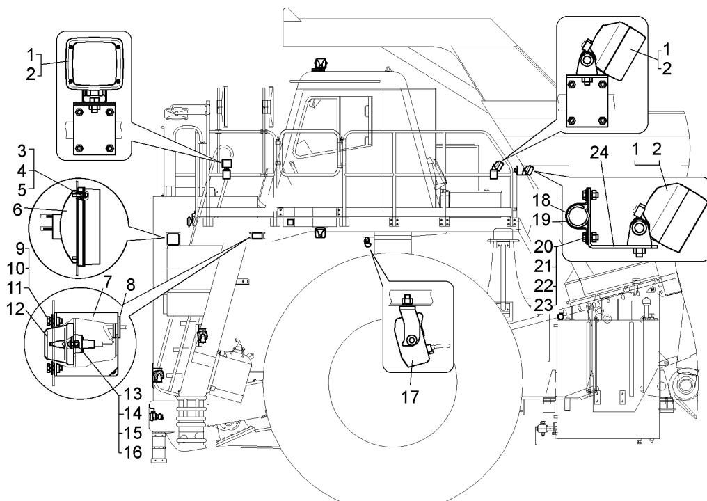
Рисунок 2.13.3 – Установка фар и подфарников (75131-3700006-30) (Рисунок1) Figure 2.13.3 – Mounting of headlights
