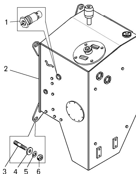
Рисунок 2.19.17 – Установка масляного бака(75131-8600034-20) Figure 2.19.17 – Mounting of oil tank
