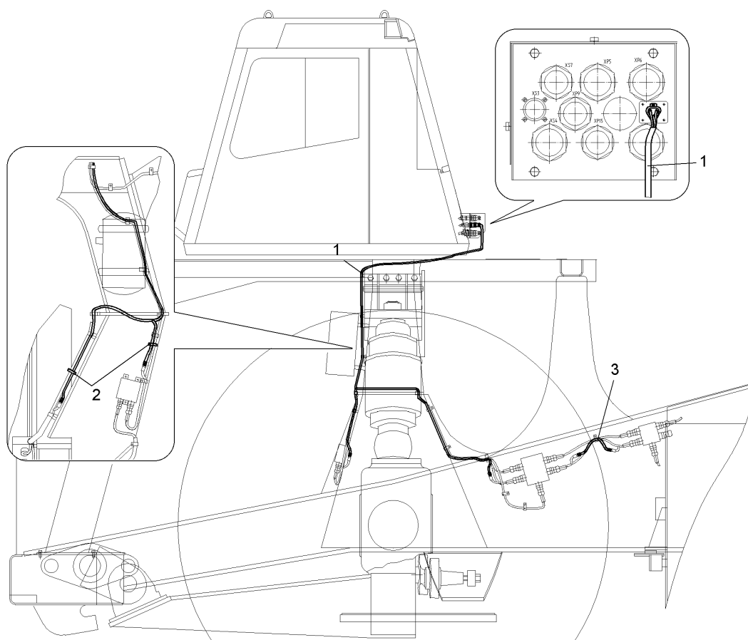
Рисунок 2.17.6– Монтаж информационной шины по шасси (75131-8077012-10) Figure 2.17.6 – Mounting of info bus over chassis
