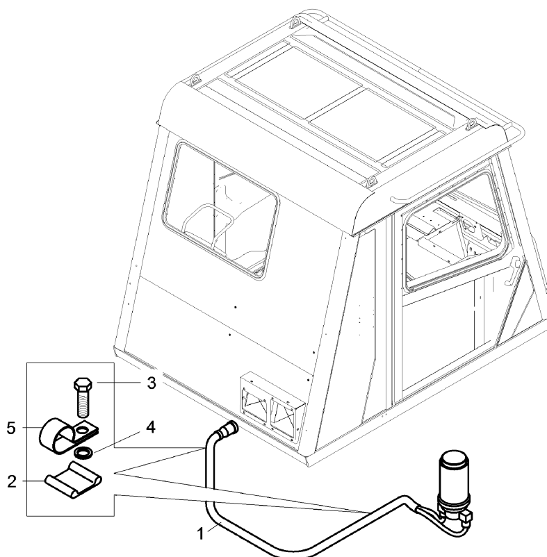
Рисунок 2.13.9 – Монтаж проводов системы смазки “Lincoln” по шасси (75172-3700055) Figure 2.13.9 – Arrangement of wiring of “Lincoln” lubrication system on chassis
