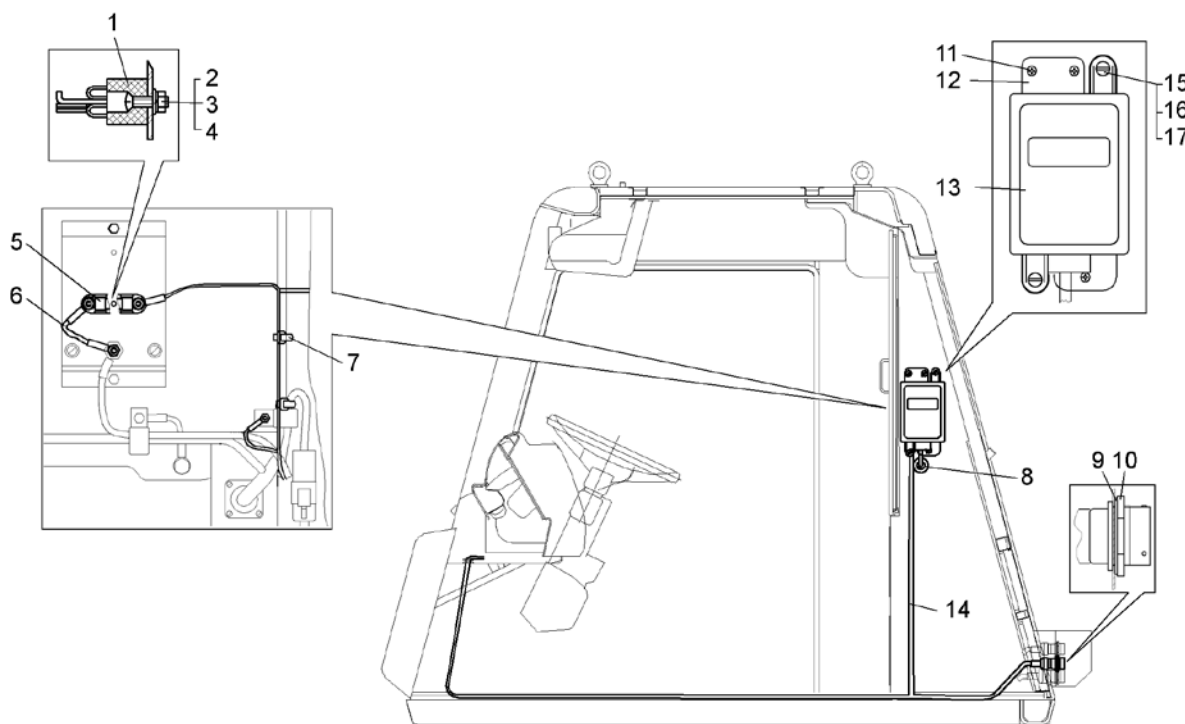
Рисунок 2.13.8 – Монтаж проводов системы смазки “Graco” в кабине (7513-3700051) Figure 2.13.8 – Arrangement of wiring of “Graco” lubrication system in the cabin
