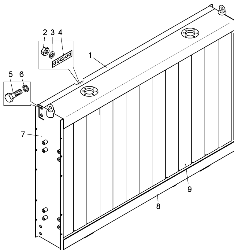
Рисунок 2.4.2– Радиатор (75131-1300008-10)
