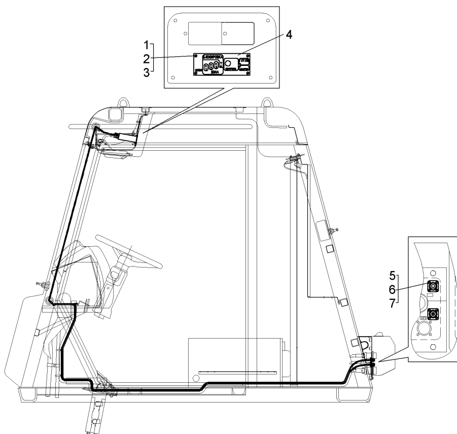
Рисунок 2.13.15 – Установка сигнализатора высоковольтной линии (75131-3733001-20) Figure 2.13.15 – Mounting signal device of approaching overhead power line
