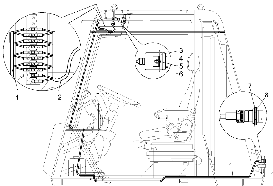
Рисунок 2.13.17 – Монтаж электрооборудования системы пожаротушения в кабине (75137-3767007-30)
