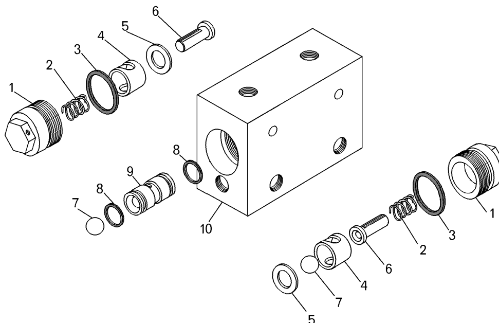
Рисунок 2.11.5 – Двойной защитный клапан (75125-3515110) Figure 2.11.5 – Dual safety valve
