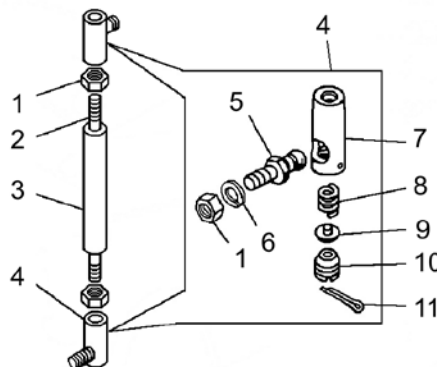
Рисунок 2.2.16 – Механизм толкающий (75483-1108450) Figure 2.2.16 – Pushing unit
