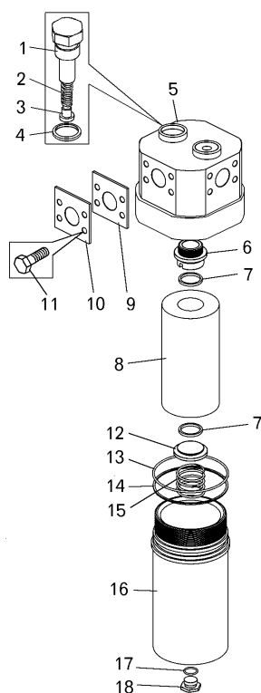
Рисунок 2.19.9 – Фильтр (75137-3442010) Figure 2.19.9 – Filter
