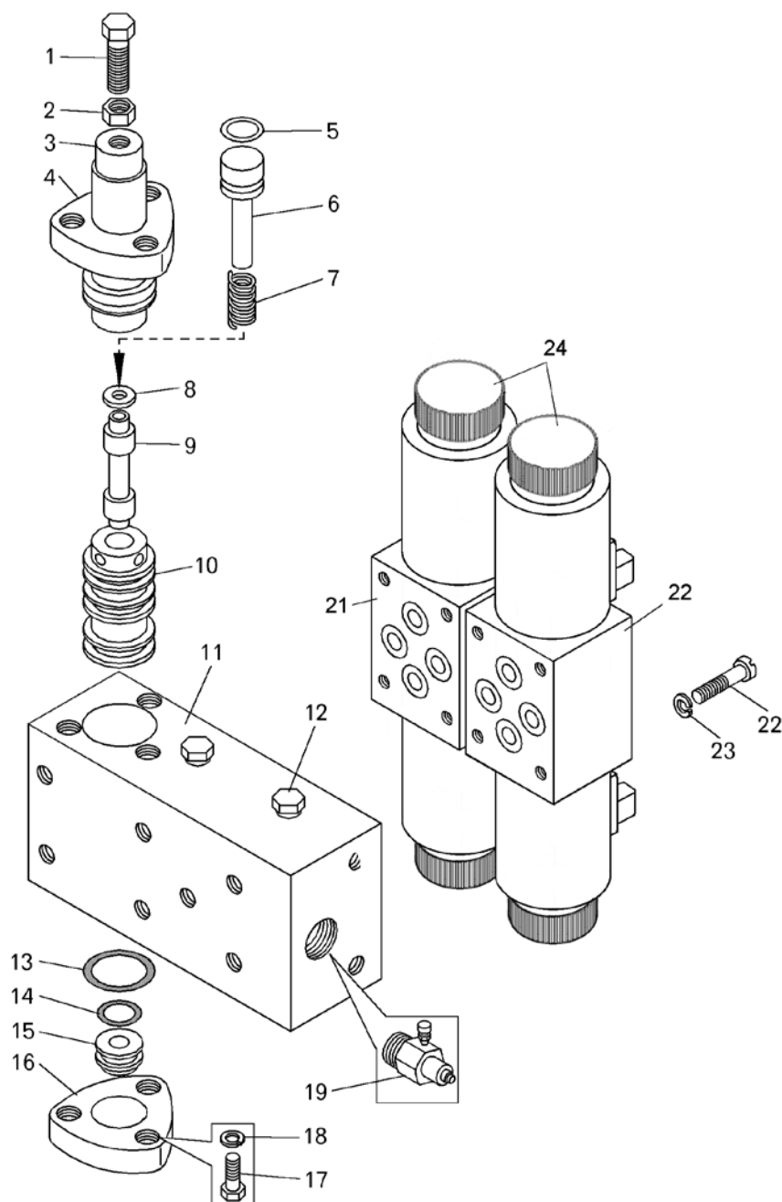
Рисунок 2.19.4 – Блок управления (75132 -8606410) Figure 2.19.4 – Control unit
