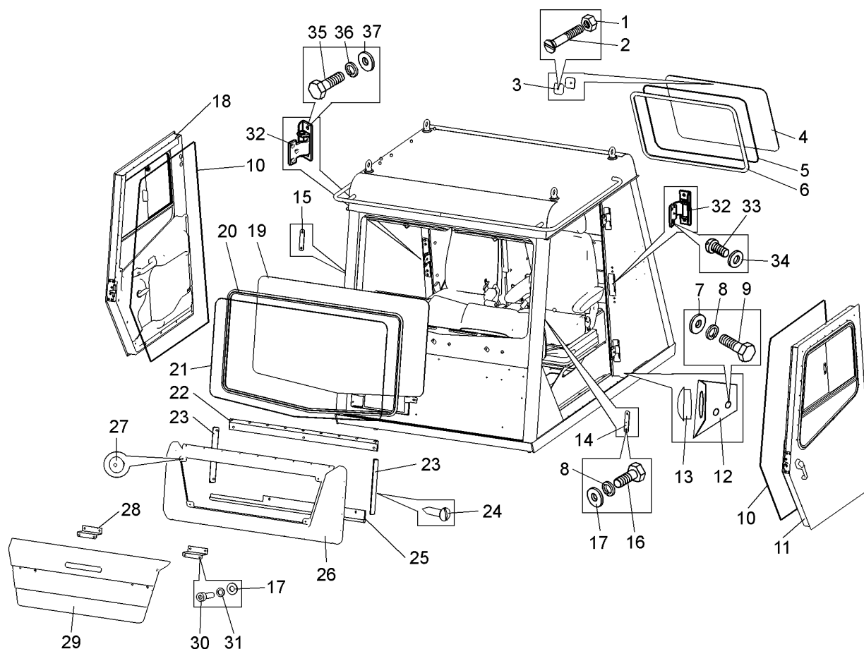
Рисунок 2.16.3 – Кабина (75306-5000012-40). Установка дверей, окон и кожуха защитного Figure 2.16.3 – Cabin. Mounting of doors, windows and protective shroud
