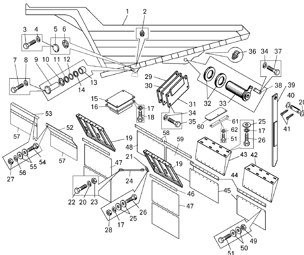
Рисунок 2.18.1 – Установка платформы, камневых толкателей и брызговиков (75136-8500001-10, 75131-3111001, 7513-8511002)
