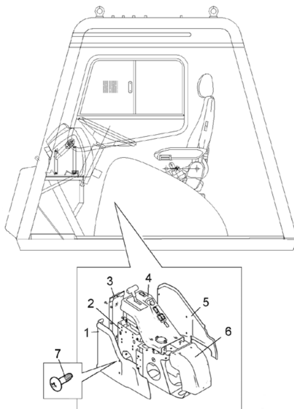
Рисунок 2.16.12 – Установка консоли в кабине (75603-5405002) Figure 2.16.12 – Mounting of console in the cabin
