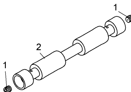
Рисунок 2.10.19 – Золотник распределителя (7822-3416550-01) Figure 2.10.19 – Distributor spool-valve
