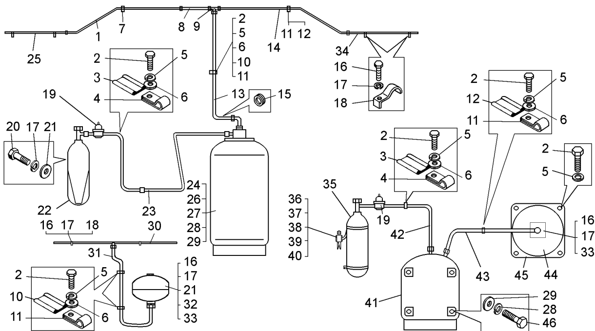
Рисунок 2.15.1 – Установка системы пожаротушения (75131-3910007-10) Figure 2.15.1 – Mounting of fire fighting system
