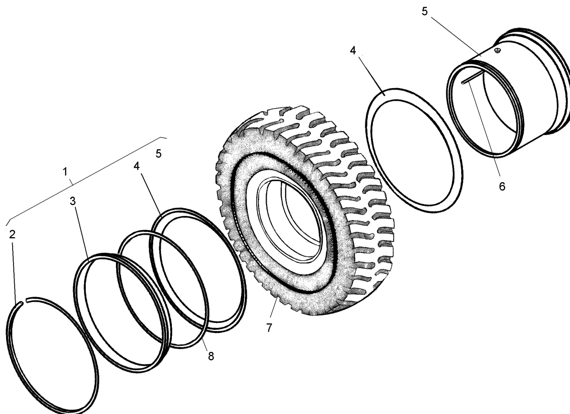
Рисунок 2.9.5 – Детали колес (75131-3101011) Figure 2.9.5 – Wheels parts
