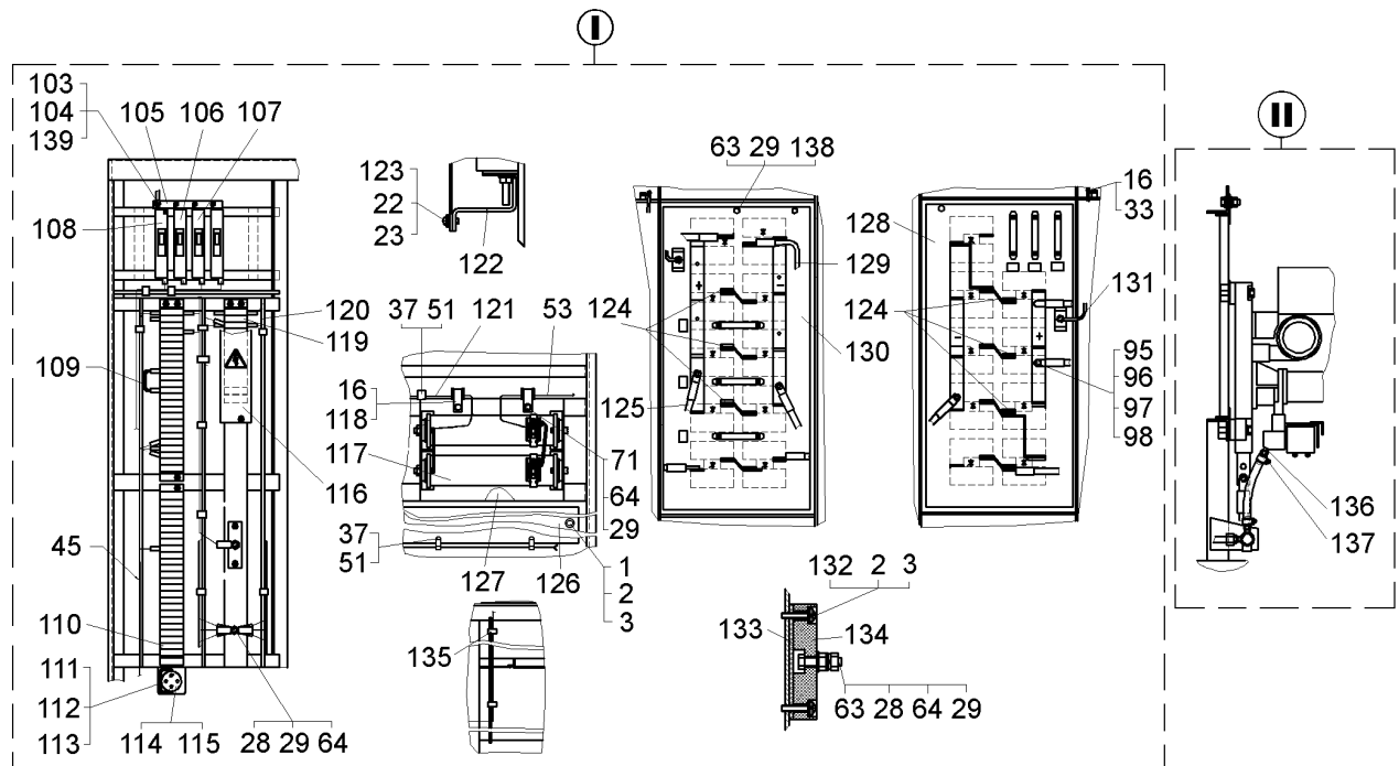
Рисунок 2.5.4 – Шкаф с пускорегулирующей аппаратурой (продолжение рис. 2.5.3) (75131-2112010-21) Figure 2.5.3 – Cabinet with start-up control equipment
