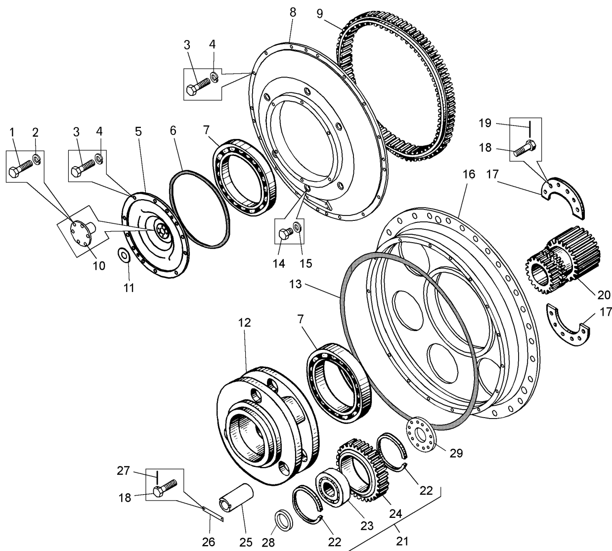
Рисунок 2.6.7 – Ряд первый редуктора электромотор-колеса (75132-2405250-03) Figure 2.6.7 – First row of electromotor-wheel reducer
