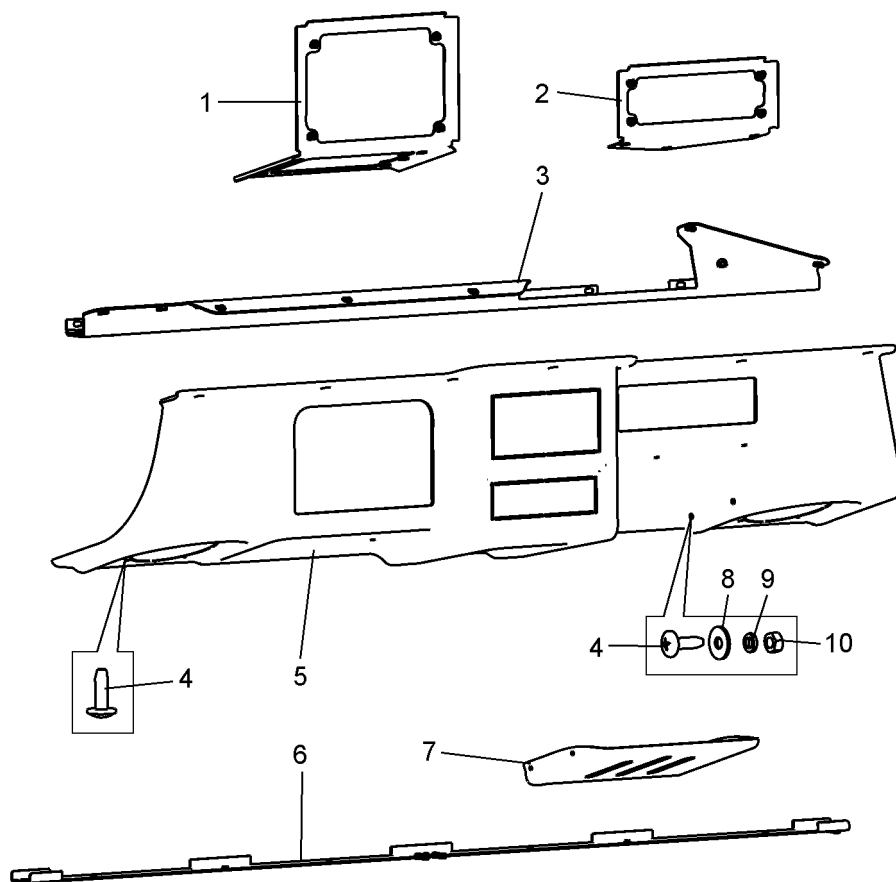
Рисунок 2.16.9 – Панель приборов верхняя (7555В-5325250-10)
