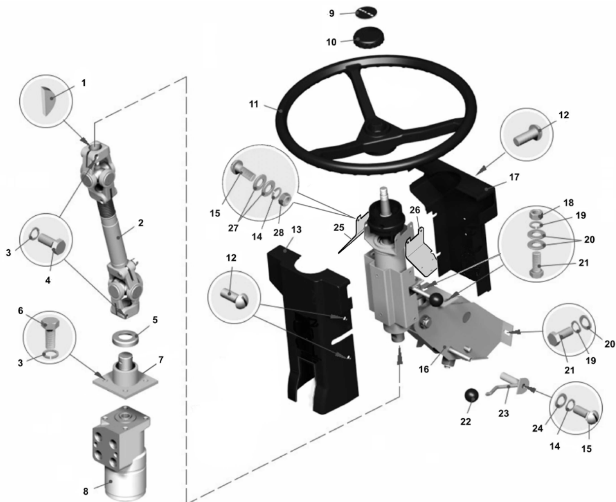
Рисунок 2.10.1 – Установка рулевого управления (75131-3400001-30)
