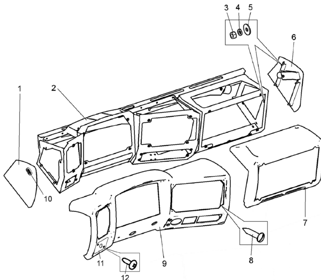
Рисунок 2.16.8– Панель приборов (7555В-5325440-10)
