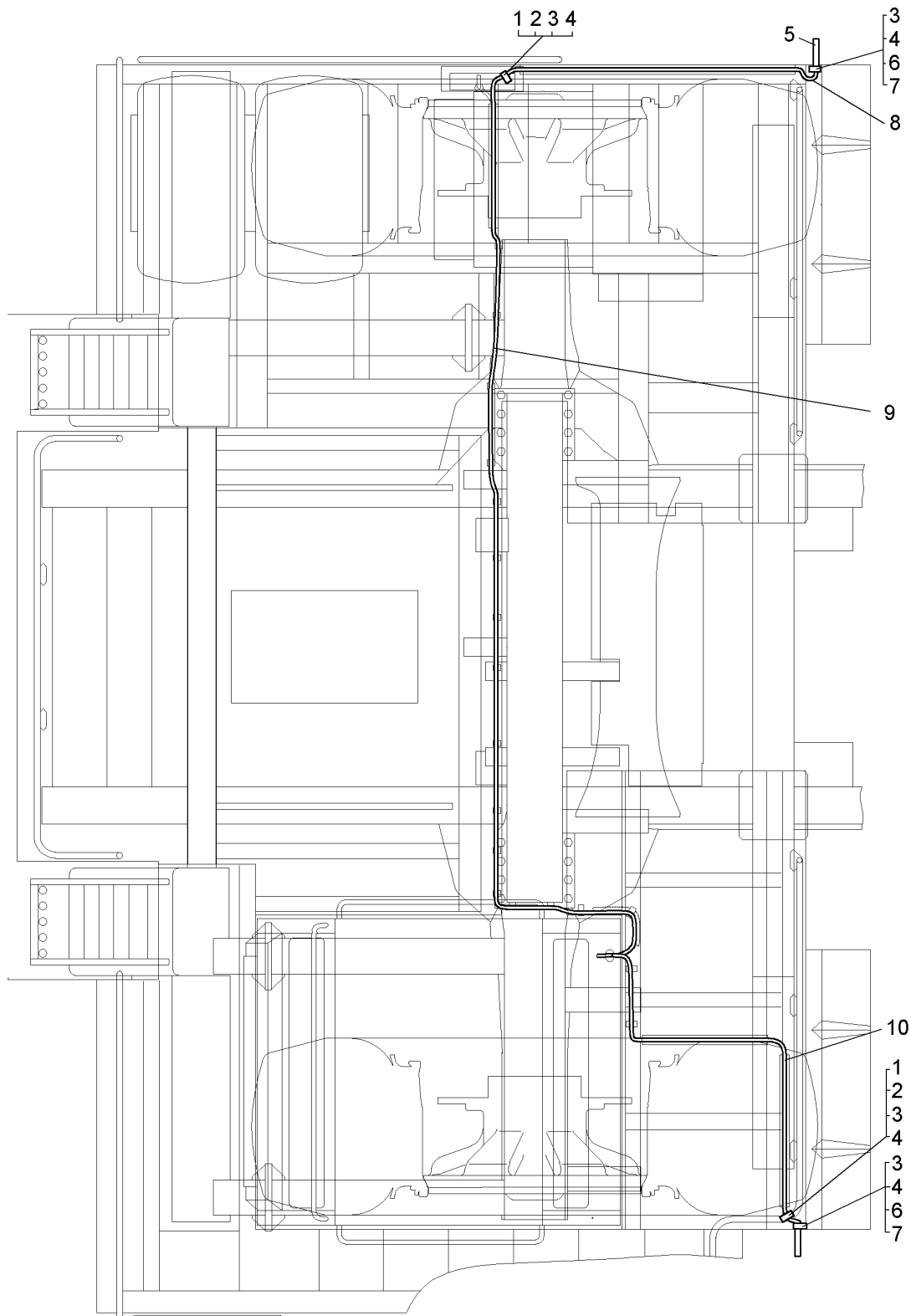
Рисунок 2.13.13 – Монтаж системы контроля давления в шинах по шасси (75131-3700080-30) Figure 2.13.13 – Mounting of the tires pressure control system over chassis
