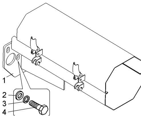
Рисунок 2.19.16 – Установка ограждения карданного вала (75310-2235002) Figure 2.19.16 – Mounting of cardan shaft protective cover
