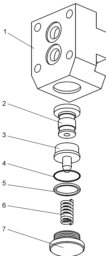
Рисунок 2.19.7– Клапан предохранительный (7823-4617100,78211-4617100) Figure 2.19.7– Safety valve
