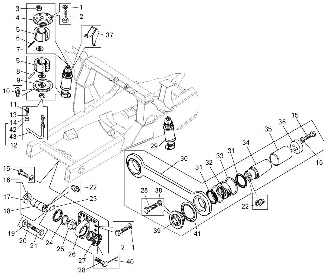
Рисунок 2.8.1 – Установка передней подвески (75131-2900001-60)
