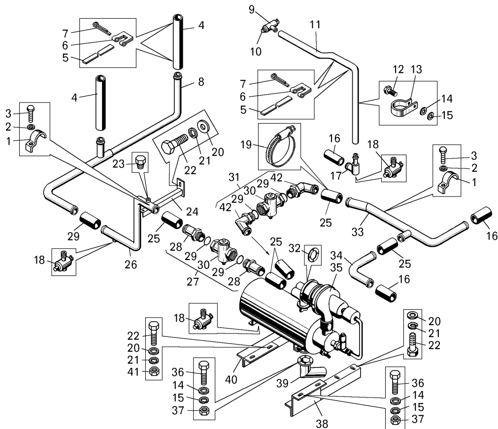
Рисунок 2.1.9 – Установка предпускового подогревателя(75131-1000008-10) Figure 2.1.9 – Mounting of pre-starting heater
