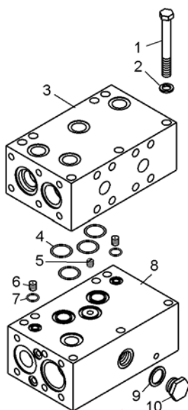
Рисунок 2.10.20 – Блок корпусов с дросселями (75306-3416608-10) Figure 2.10.20 – Set of bodies with throttles
