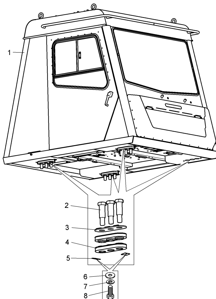
Рисунок 2.16.2 – Кабина (75306-5000012-40). Установка подушек опоры кабины Figure 2.16.2 – Cabin. Mounting of cab support pads
