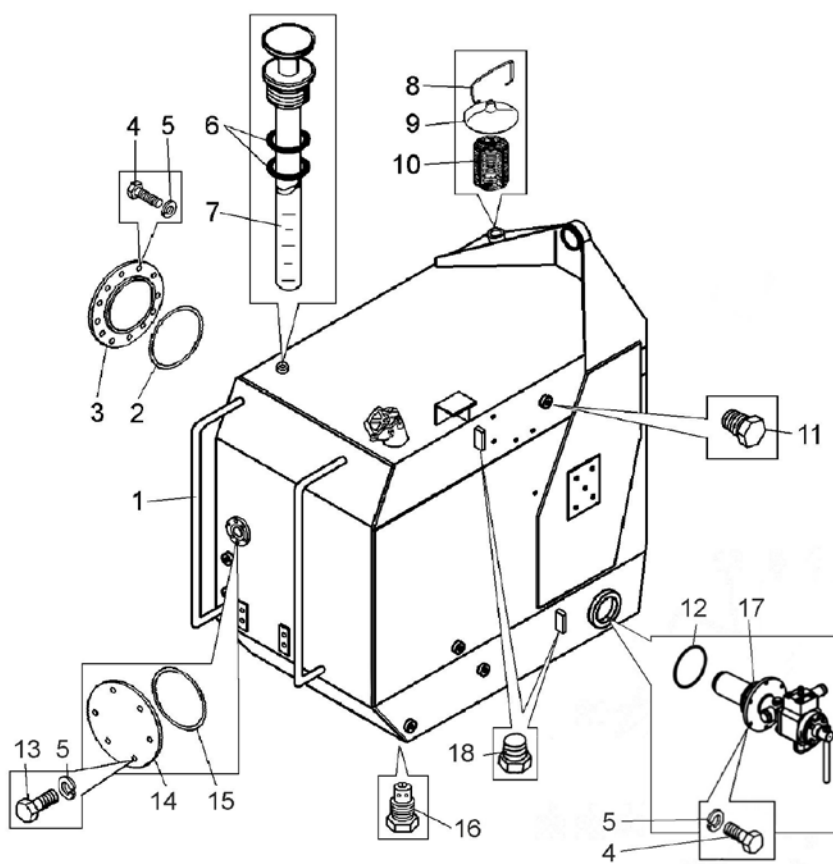
Рисунок 2.2.2 – Бак топливный (75131-1101010-40)
