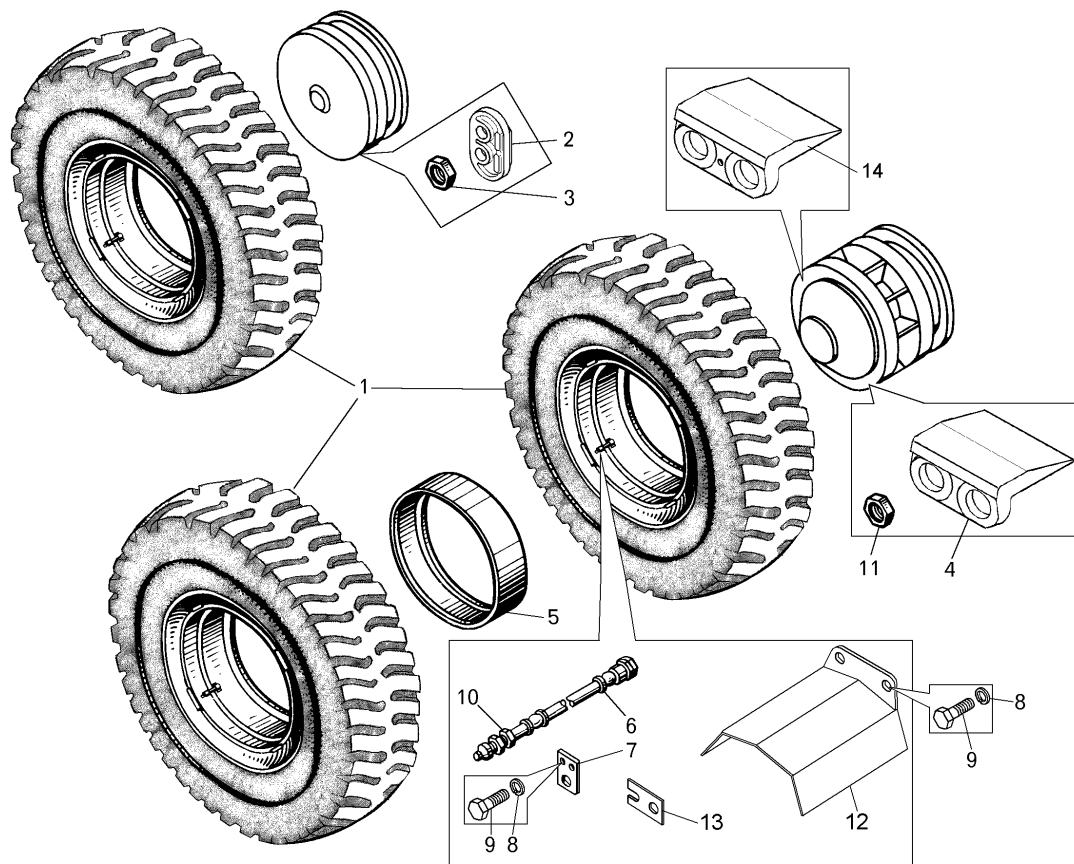
Рисунок 2.9.4 – Колеса и детали их крепления (7513-3100004, 75136-3100005) Figure 2.9.4 – Wheels and parts of their fastening
