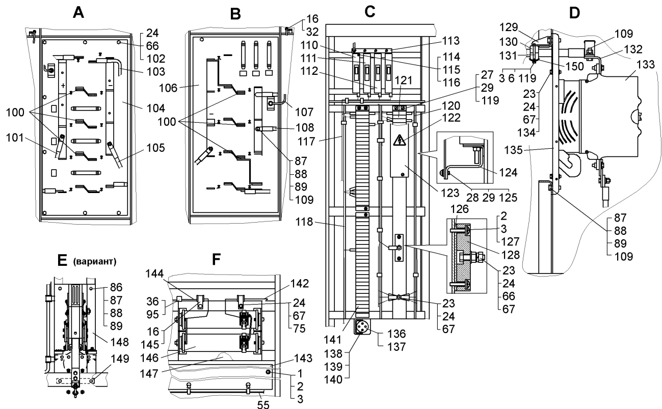
Рисунок 2.5.6 – Шкаф с пускорегулирующей аппаратурой (продолжение рис. 2.5.5) (75131-2112010-31) Figure 2.5.6 – Cabinet with start-up control equipment
