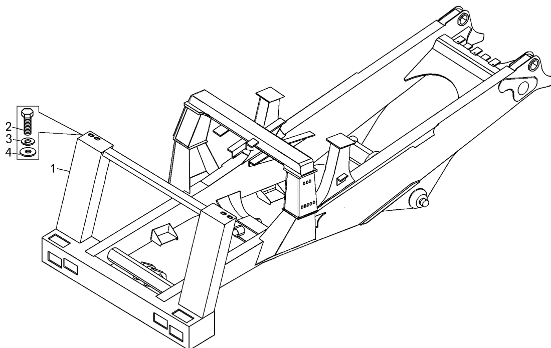
Рисунок 2.7.1 – Рама (75131-2800010-31) Figure 2.7.1 – Frame
