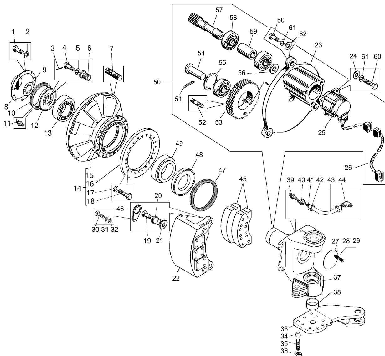
Рисунок 2.9.2 – Кулак поворотный с тормозами и поворотным механизмом (75131-3001006, 75131-3001007)
