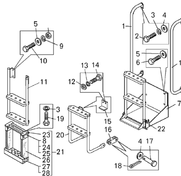
Рисунок 2.16.16 – Установка площадок и поручней (75136-8012006) Figure 2.16.16 – Mounting of platforms and handholds
