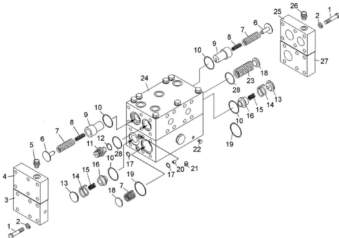
Рисунок 2.10.15 – Распределитель рулевого управления с усилителем потока (75131-3416600) Figure 2.10.15 – Distributor of steering with flow booster
