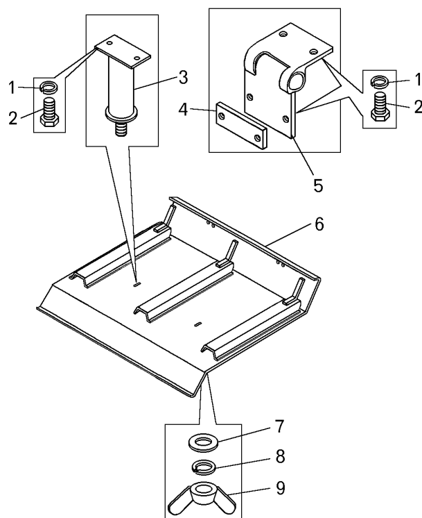
Рисунок 2.16.10 – Установка кожуха пола (75131-5107003) Figure 2.16.10 – Mounting of floor shroud
