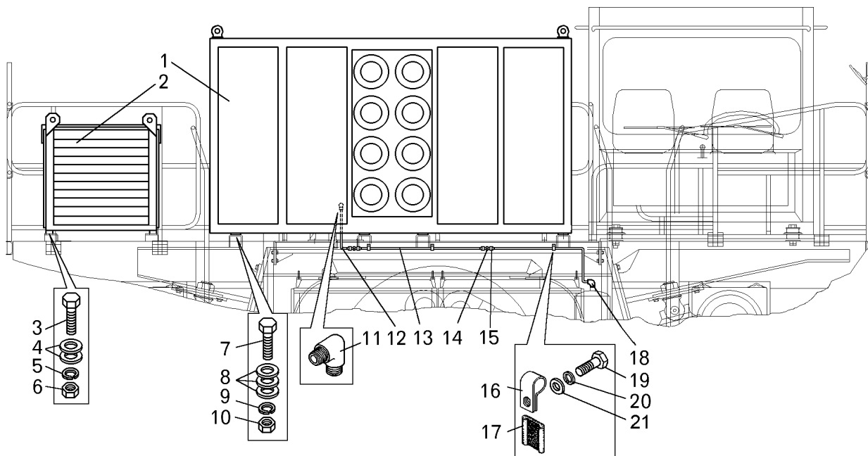
Рисунок 2.5.1 – Установка электрооборудования (75131-210022-14) Figure 2.5.1 – Mounting of electrical equipment
