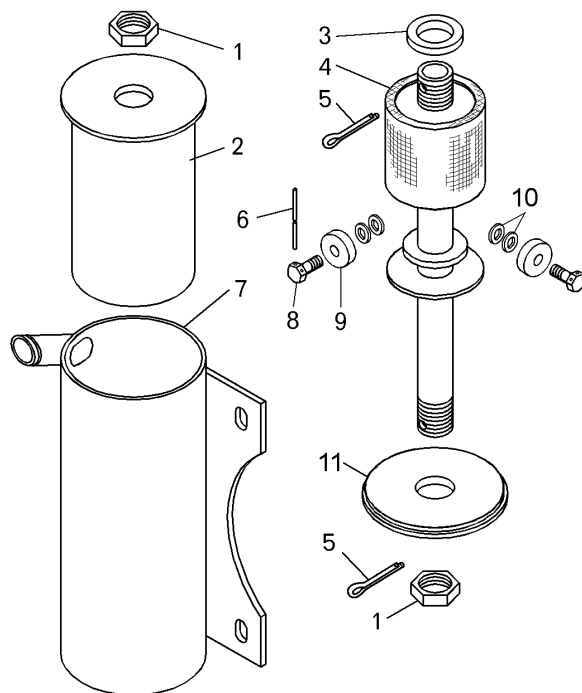
Рисунок 2.6.6 – Фильтр (75132-2405070, 75132-2405071) Figure 2.6.6 – Filter
