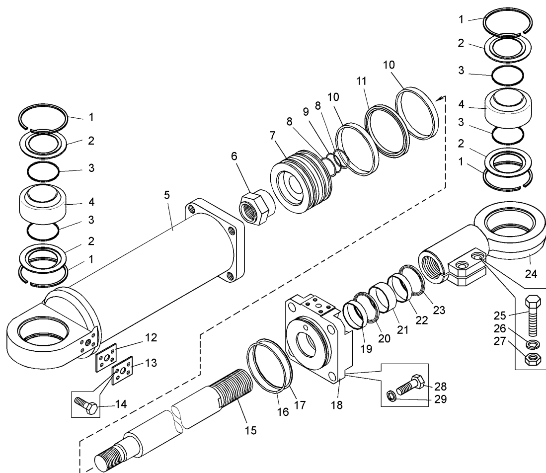
Рисунок 2.10.10 – Цилиндр поворота (75131-3429010-40)
