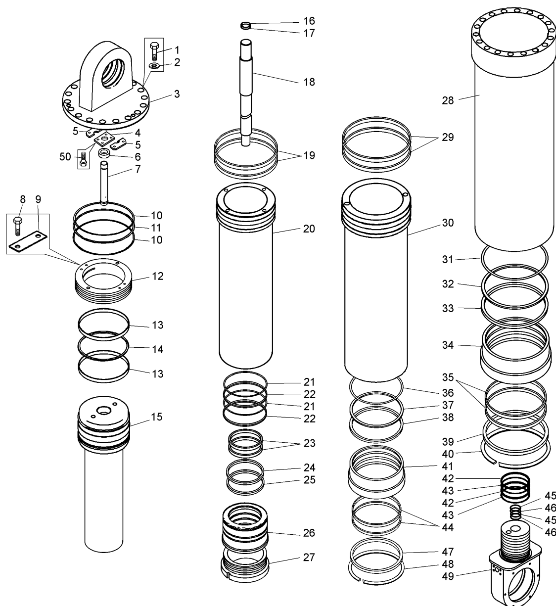
Рисунок 2.19.2 – Цилиндр опрокидывающего механизма (75131-8603010)
