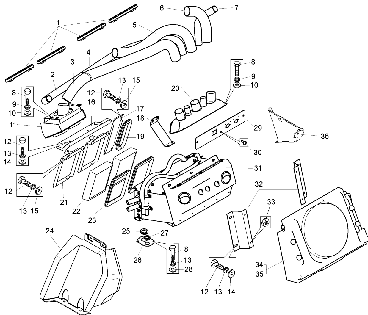
Рисунок 2.16.17 – Установка отопительнокондиционерного блока (7555B-8100002-50) Figure 2.16.17 – Mounting of heating and conditioning unit
