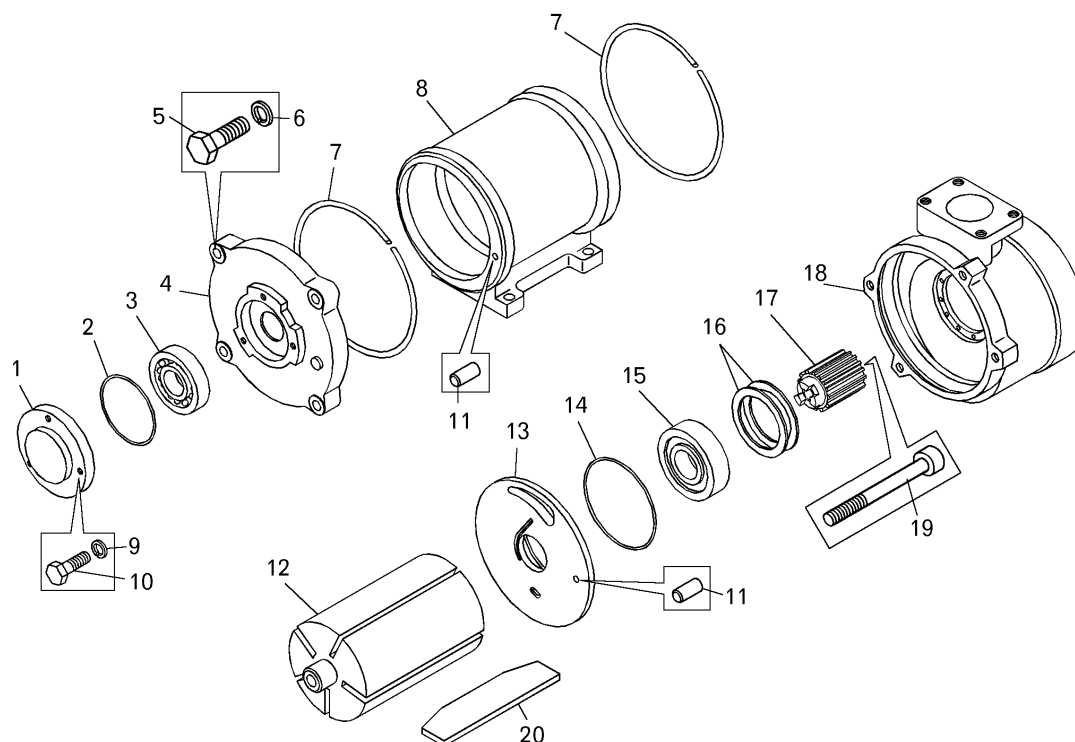
Рисунок 2.1.11 – Пневмодвигатель (7549-1026100)
