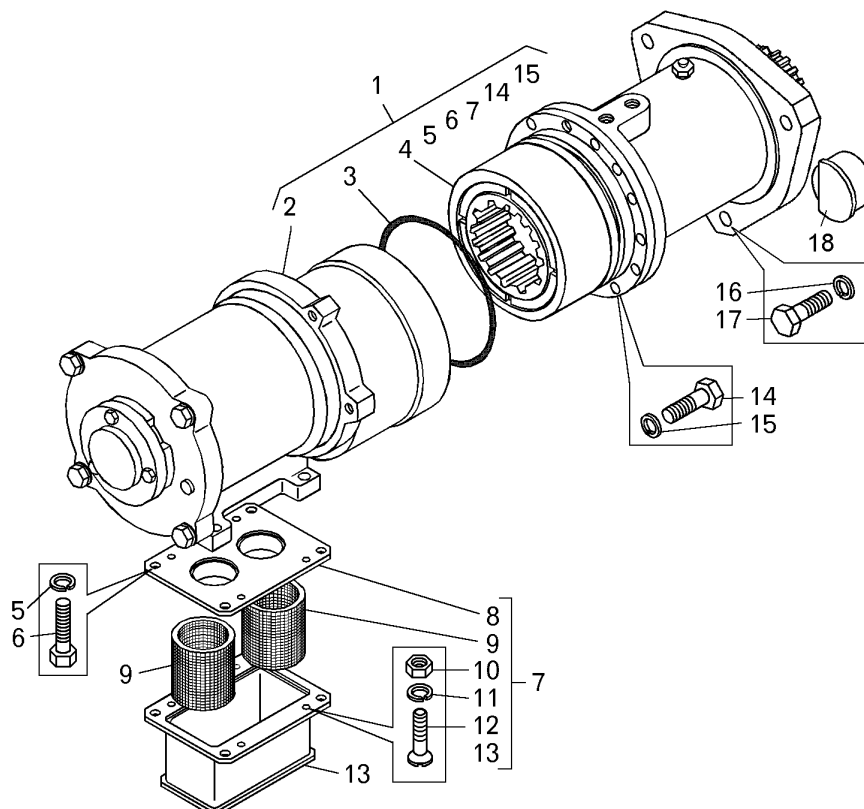
Рисунок 2.1.10 – Пневмостартер и его установка (75131-1026002) Figure 2.1.10 – Pneumatic starter
