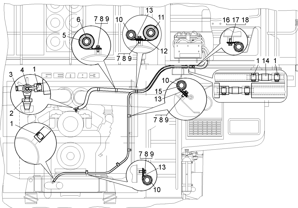
Рисунок 2.16.18 – Установка трубопроводов отопителя кабины (75131-8100005) Figure 2.16.18 – Mounting of pipelines in the cabin heater
