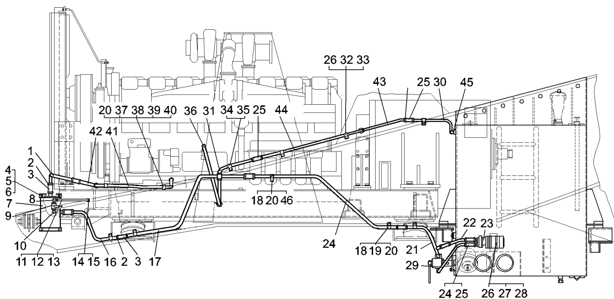
Рисунок 2.2.10 – Топливные трубопроводы (75131-1100006-10)
