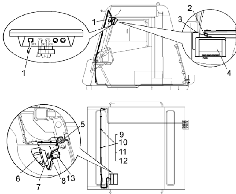
Рисунок 2.17.2 – Установка системы видеообзора по кабине (75131-7912003, 75131-7912003-01) Figure 2.17.2 – Mounting of video survey system in the cabin
