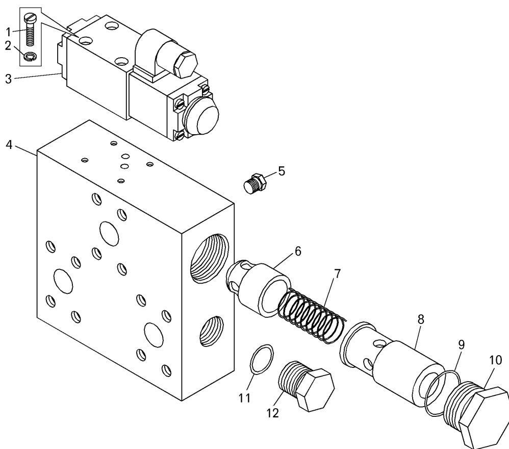
Рисунок 2.10.11 – Коллектор(75132-3408800) Figure 2.10.11 – Collector
