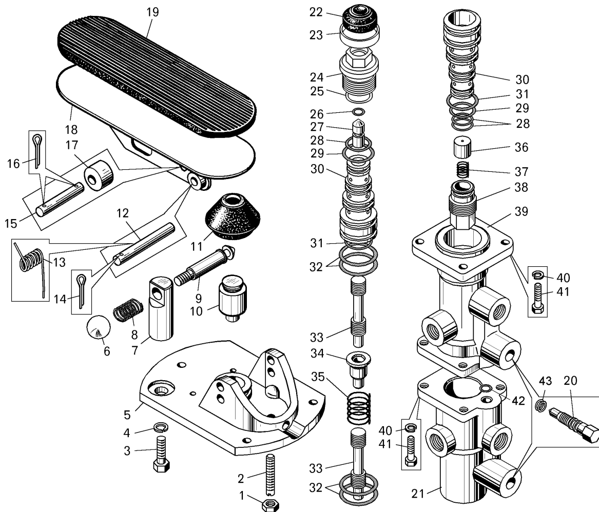
Рисунок 2.11.4– Кран управления тормозами (7555А-3514010-01) Figure 2.11.4 – Control brake valve
