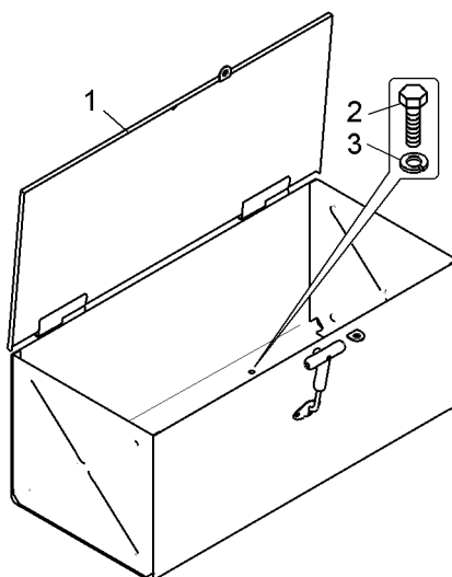
Рисунок 2.15.5 – Установка инструментального ящика (75137-3919005) Figure 2.15.5 – Mounting of instrumental box
