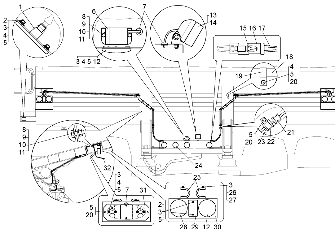
Рисунок 2.13.4 – Установка задних фонарей и фары (75131-3700009-50) Figure 2.13.4 – Mounting of taillights
