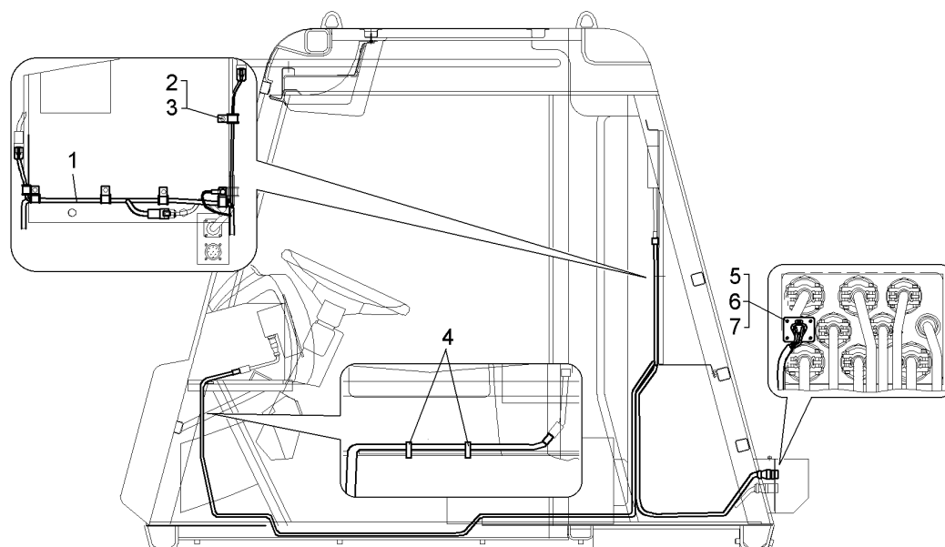
Рисунок 2.17.7 – Монтаж информационной шины по кабине (75180-8077016)
