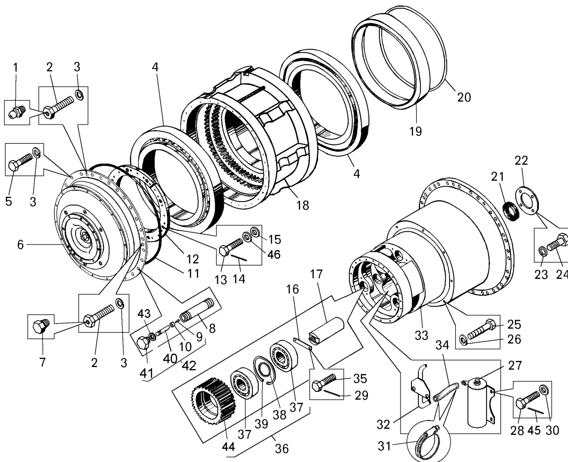
Рисунок 2.6.5 – Редуктор электромотор-колеса (75132-2405010-10) Figure 2.6.5 – Reducer of electromotor-wheel
