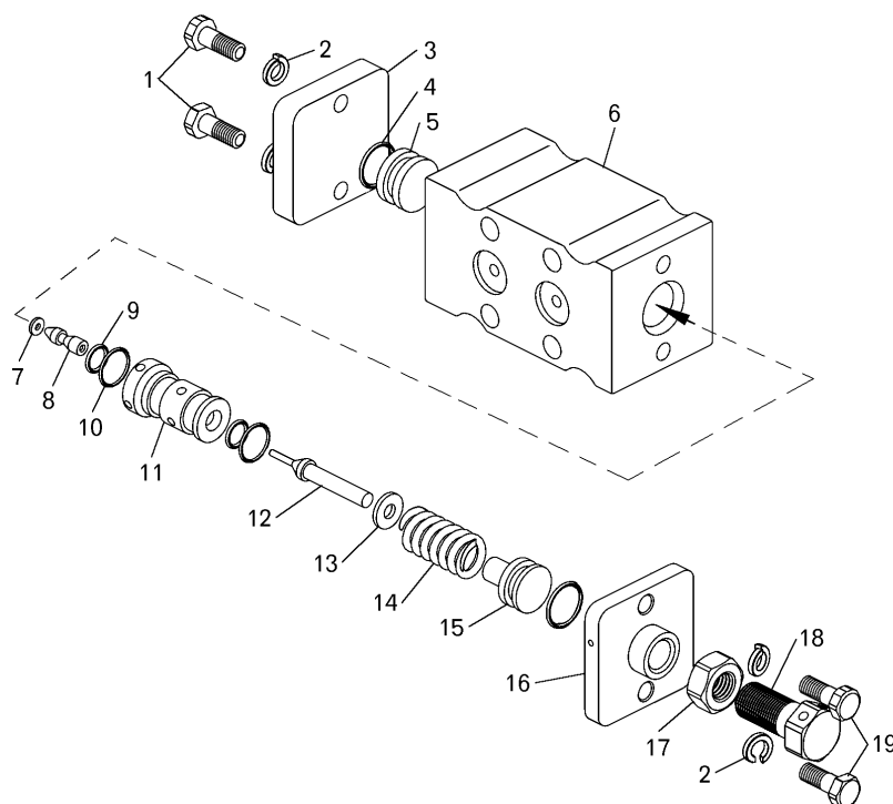
Рисунок 2.19.6 – Клапан вспомогательный (7820-4603100)
