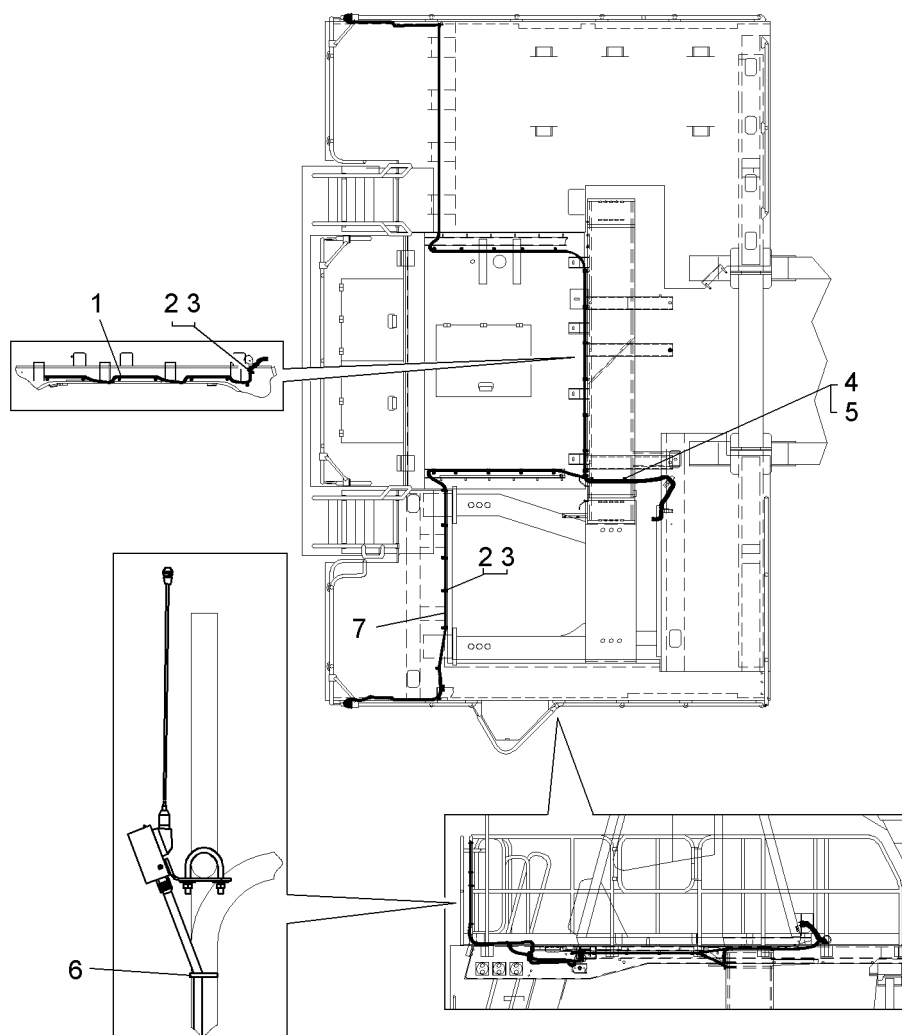
Рисунок 2.13.16 – Установка антенны высоковольтной линии (75131-3733002) Figure 2.13.16 – Mounting device antenna of approaching overhead power line
