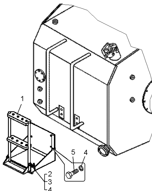
Рисунок 2.16.15 – Установка площадки топливного бака (75131-8012005-10) Figure 2.16.15 – Mounting of fuel tank decks
