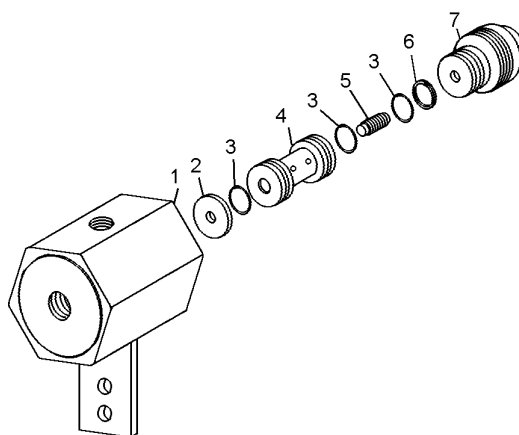
Рисунок 2.11.3 – Клапан двухмагистральный (78221-4619074) Figure 2.11.3 – Double-way valve
