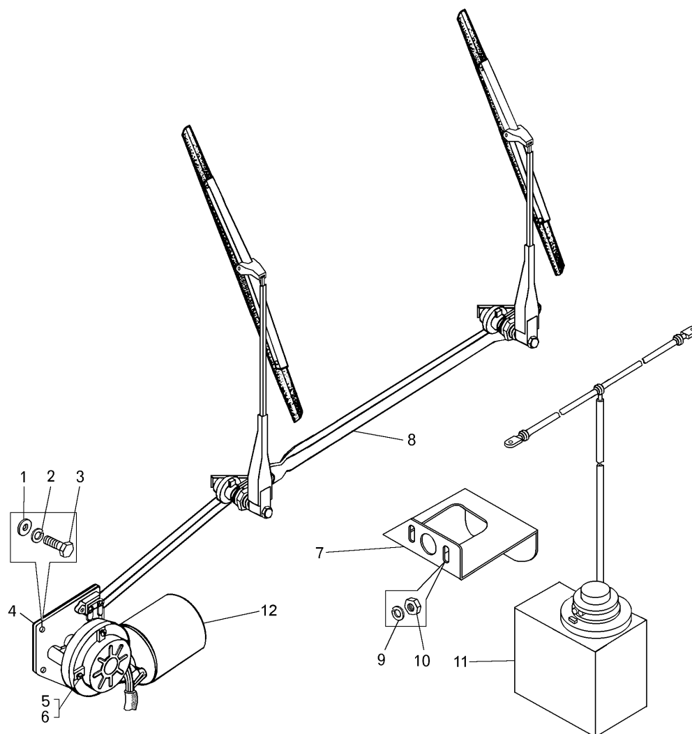
Рисунок 2.16.11 – Установка стеклоочистителя (7555В-5205002) и стеклоомывателя (75306-5208002) Figure 2.16.11 – Mounting of windshield wipers and windshield washer
