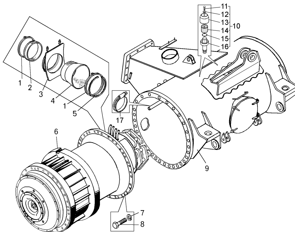
Рисунок 2.6.1 – Мост задний (75132-2400010, 75132-2400010-01, 75132-2400010-02, 75132-2400010-03, 75132-2400010-06) Figure 2.6.1 – Rear axle
