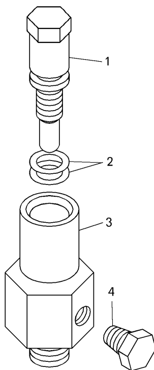
Рисунок 2.11.2– Клапан соединительный (75212-3408430) Figure 2.11.2 – Connective valve
