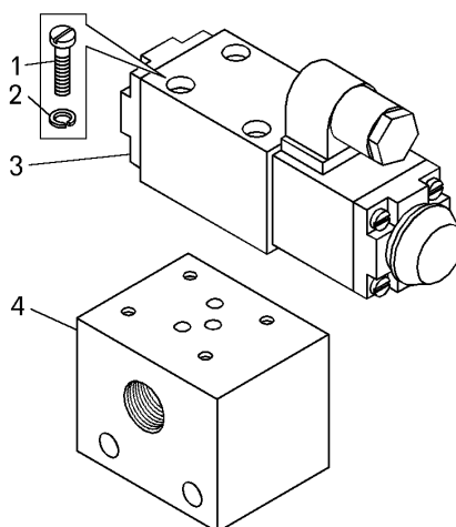
Рисунок 2.11.6 – Распределитель (75450-3537070) Figure 2.11.6 – Distributor
