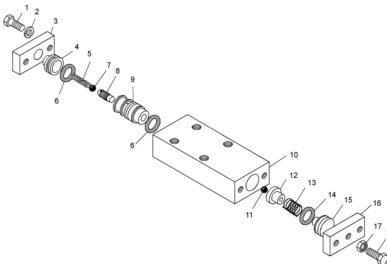
Рисунок 2.19.12 – Блок управления (75131-3428020) Figure 2.19.12 – Control unit
