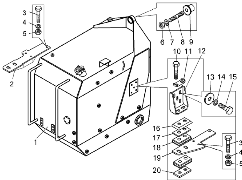
Рисунок 2.2.1 – Установка топливного бака (75131-1100001-40, 75131-1100001-41, * 75131-1100001-43) Figure 2.2.1 – Mounting of fuel tank
