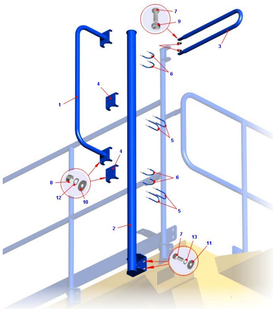
Рисунок 2.16.23 – Установка кронштейнов зеркал правого крыла (75306-8201006-10) Figure 2.16.23 – Mounting of mirrors brackets
