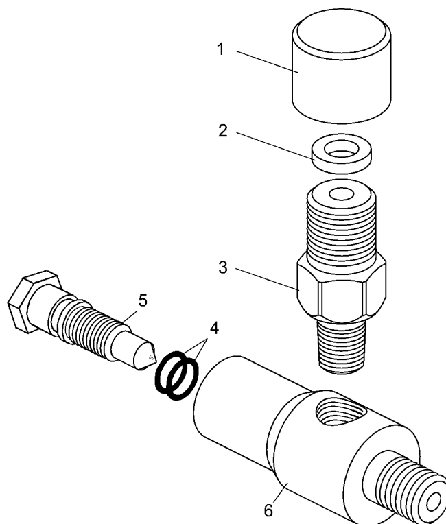
Рисунок 2.19.8 – Клапан (75306-8609360) Figure 2.19.8 – Valve
