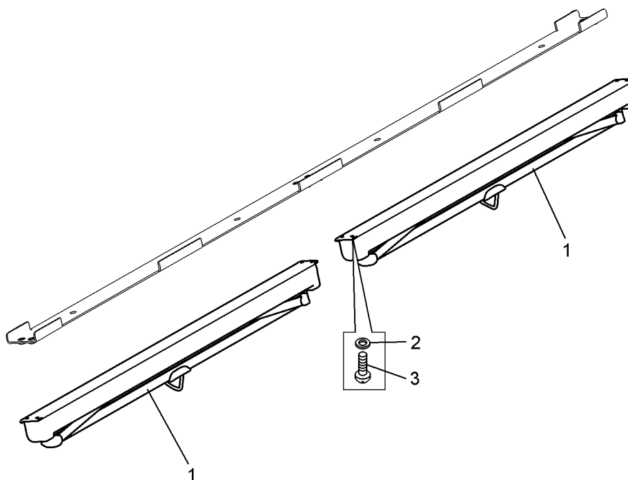
Рисунок 2.16.24 – Установка противосолнечной шторки (7555В-8204005-10) Figure 2.16.24 – Mounting of sun visor
