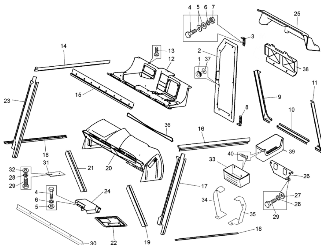
Рисунок 2.16.4 – Кабина (75306-5000012-40). Установка приборных панелей и накладок Figure 2.16.4 – Cabin. Mounting of instrumentation panels and linings
