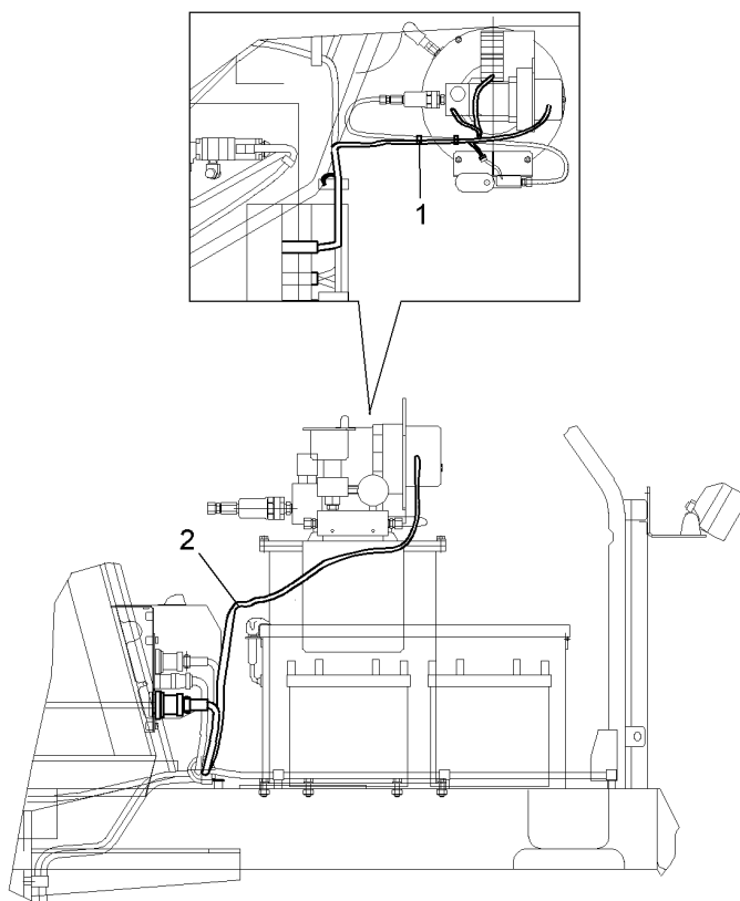
Рисунок 2.13.10– Монтаж проводов системы смазки “Graco” по шасси (7513-3700053) Figure 2.13.10 – Arrangement of wiring of “Graco” lubrication system on chassis
