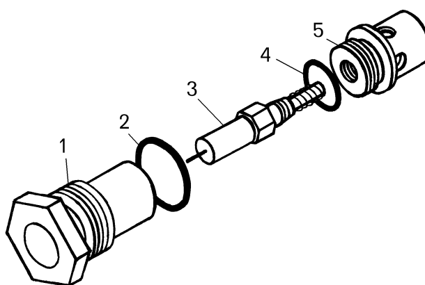
Рисунок 2.19.19 – Датчик аварийного уровня масла (75481-8608172) Figure 2.19.19 – Sensor of emergency oil level
