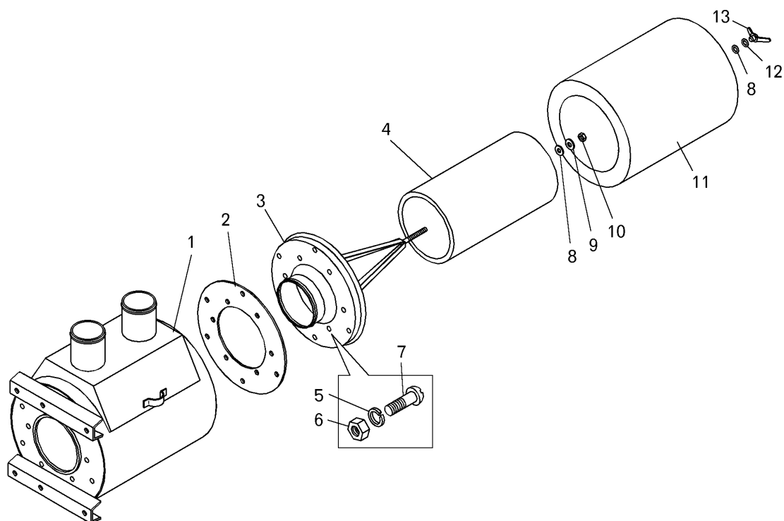
Рисунок 2.2.9 – Фильтр воздушный (7513-1109010-10)
