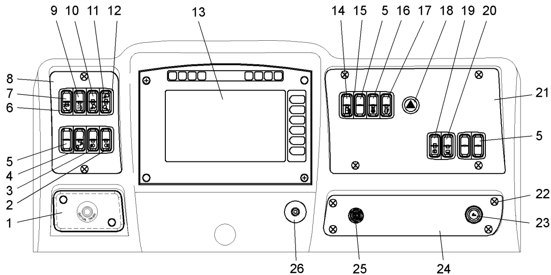
Рисунок 2.13.19 – Установка панели приборов (75131-3800020-50)
