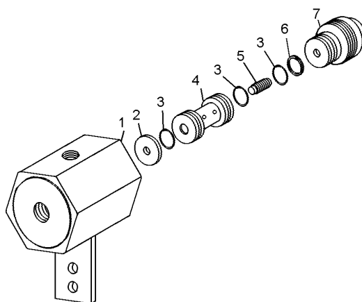
Рисунок 2.19.13 – Клапан двухмагистральный (78221-4619074) Figure 2.19.13 – Double-way valve
