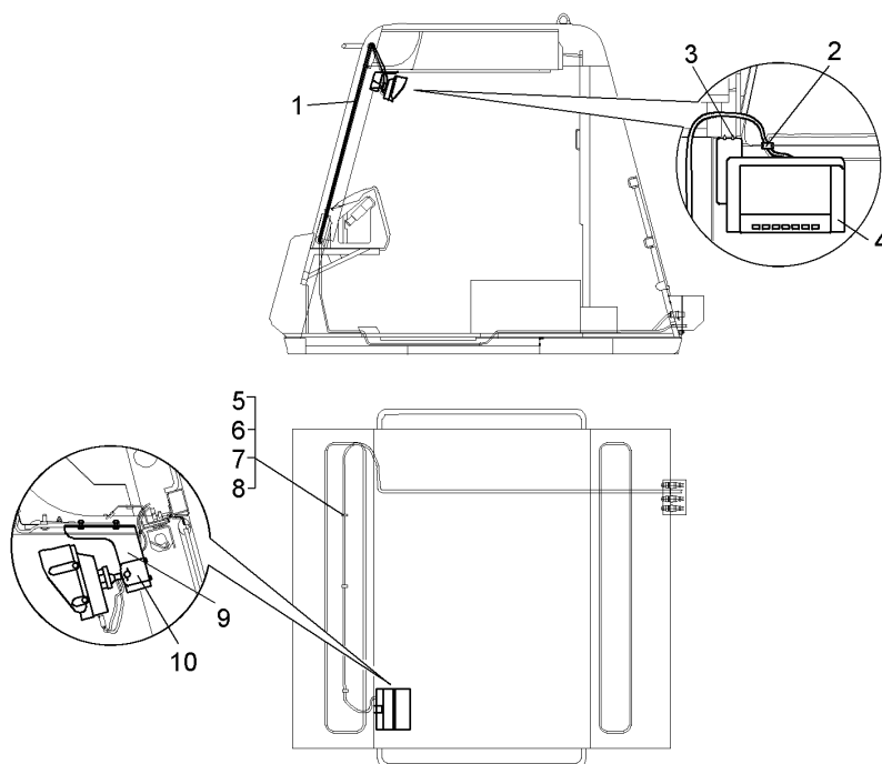
Рисунок 2.17.3 – Установка системы видеобзора по кабине (75131-7912003-02) Figure 2.17.3– Mounting of video survey system in the cabin
