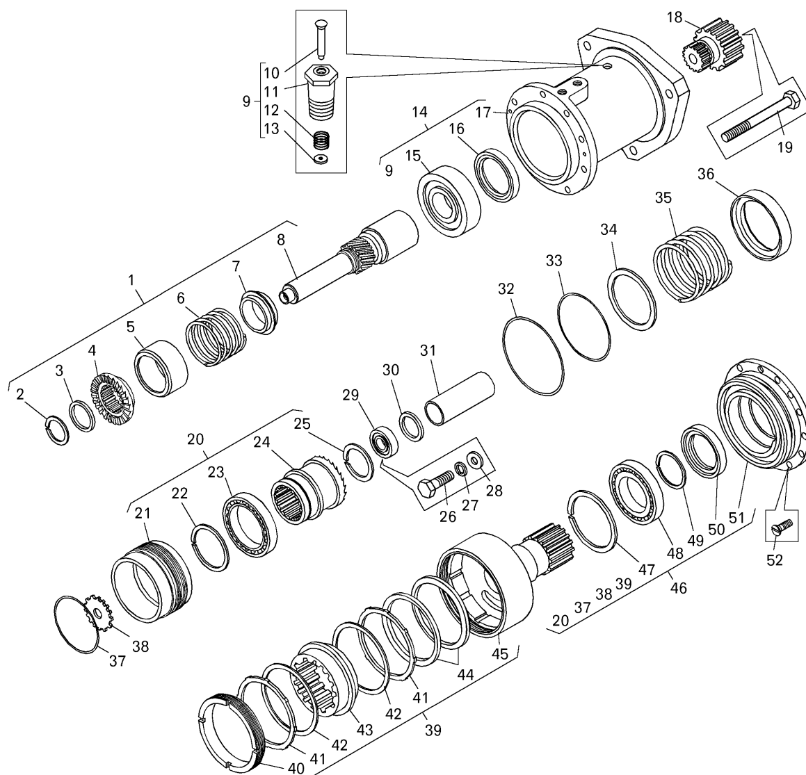
Рисунок 2.1.12 – Привод пневмостартера (75131-1026200)
