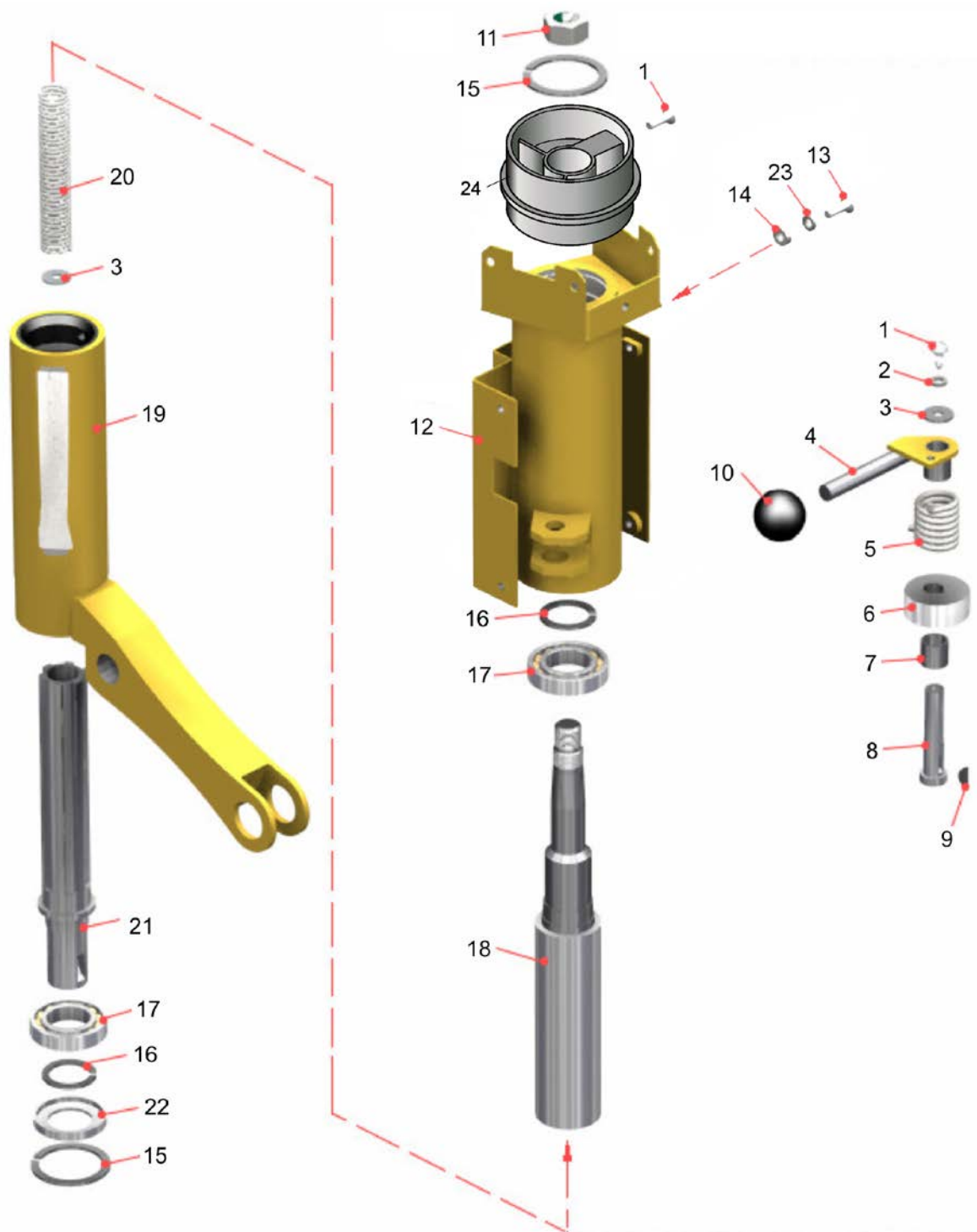
Рисунок 2.10.5 – Колонка рулевого управления (75474-3444010) Figure 2.10.5 – Steering column
