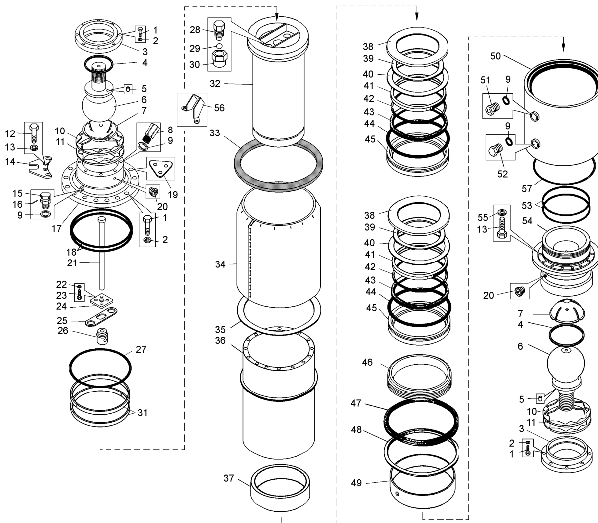
Рисунок 2.8.4 – Цилиндр подвески задний (75131-2917020-10, 75131-2917021-10) Figure 2.8.4 – Rear suspension cylinder
