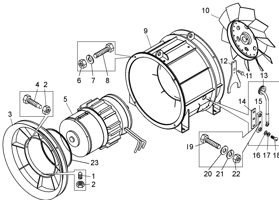
Рисунок 2.5.9 – Вентилятор (75139-2126910, 75139-2126910-01) Figure 2.5.9 – Fan
