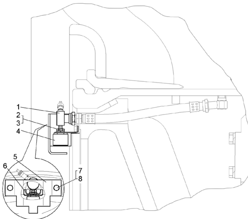
Рисунок 2.9.6 – Установка корпусов СКТ передних колес (75131-3116004-20) Figure 2.9.6 – Mounting of CKT bodies in front wheels
