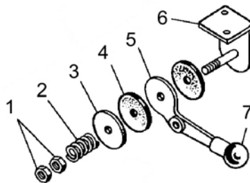
Рисунок 2.2.15 – Ручка (549Б-1108280) Figure 2.2.15 – Handle
