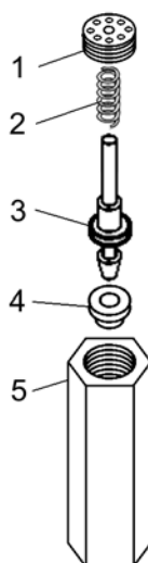
Рисунок 2.1.7 – Клапан обратный (7547-1032120-10)
