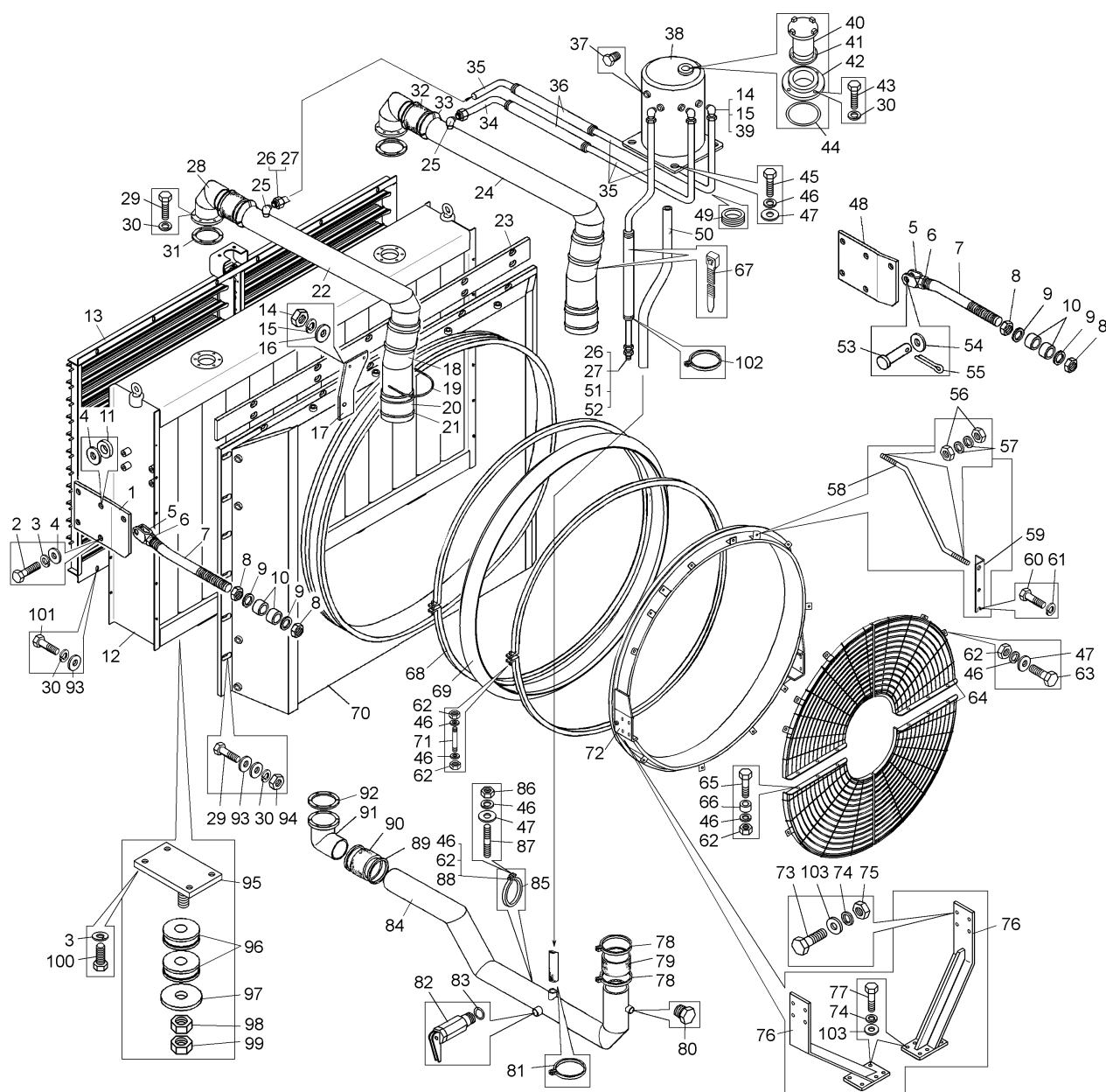
Рисунок 2.4.1 – Установка системы охлаждения двигателя (75131-1300010-40)
