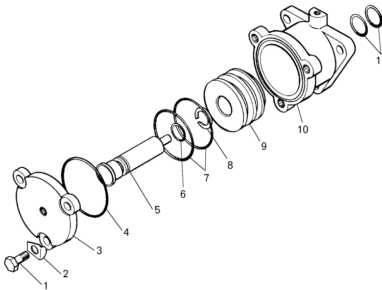
Рисунок 2.4.5 – Пневмопереключатель (549Б-1310300) Figure 2.4.5 – Pneumatic switch
