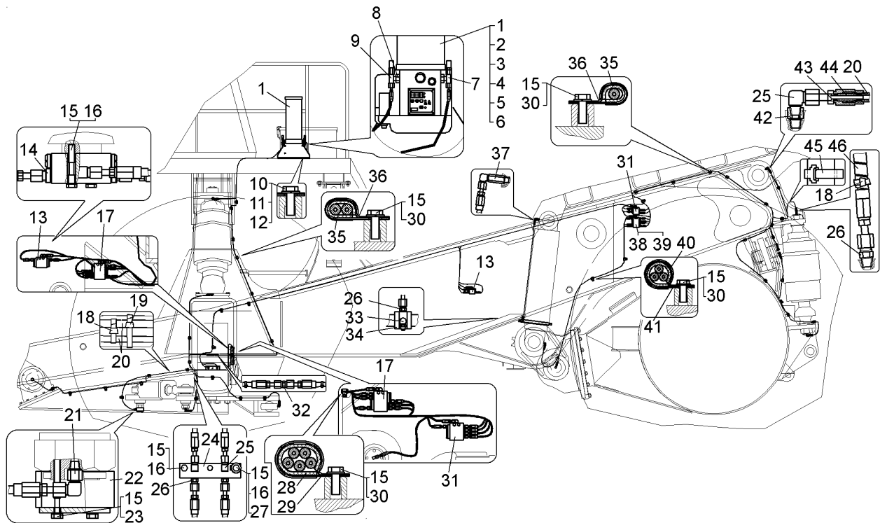
Рисунок 2.15.3 – Установка централизованной системы смазки "Lincoln" (75131-6600030)
