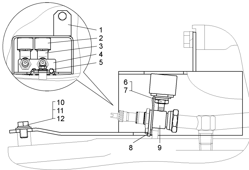
Рисунок 2.9.7 – Установка корпусов СКТ задних колес (75131-3116005-20) Figure 2.9.7 – Mounting of CKT bodies in rear wheels
