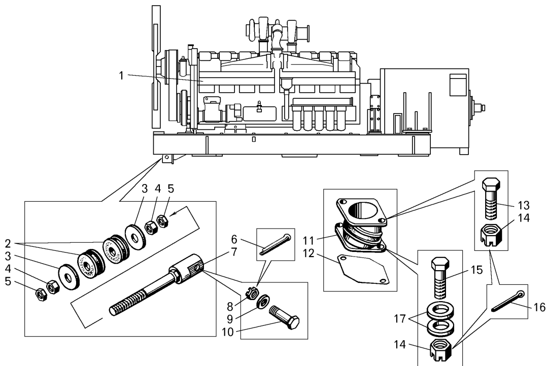
Рисунок 2.1.1 – Установка дизель – генератора (75131-1000003-03)
