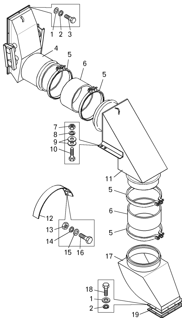
Рисунок 2.5.12 – Установка всасывающих воздухопроводов (75131-2100044-30) Figure 2.5.12 – Mounting of suction air ducts
