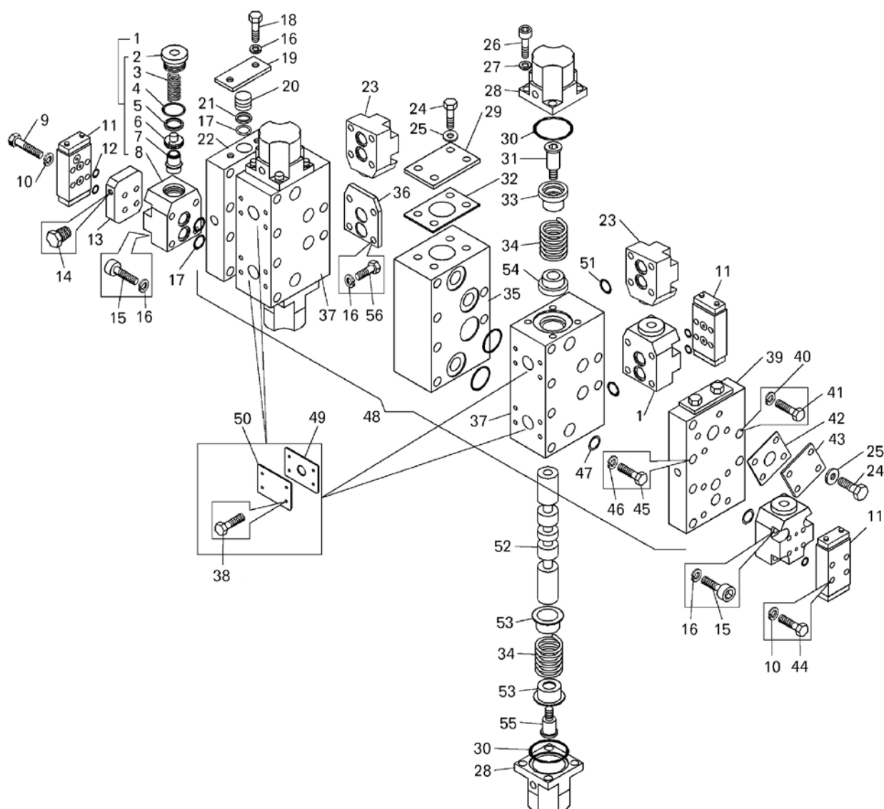
Рисунок 2.19.5 – Гидрораспределитель (75306-8606100-10) Figure 2.19.5 – Hydraulic distributor
