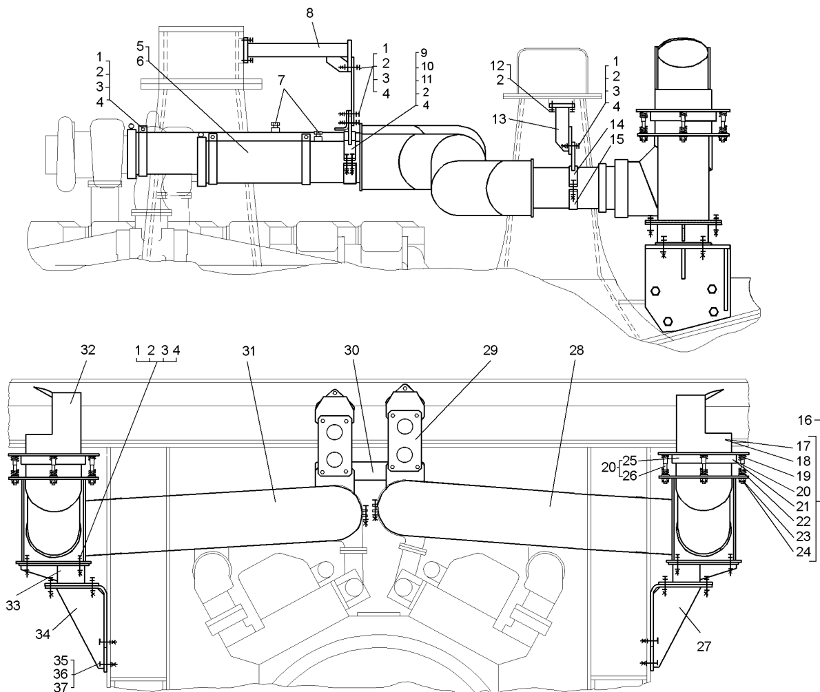
Рисунок 2.3.1 – Установка системы выпуска отработавших газов (75131-1200003-20) Figure 2.3.1 – Mounting of the exhaust system
