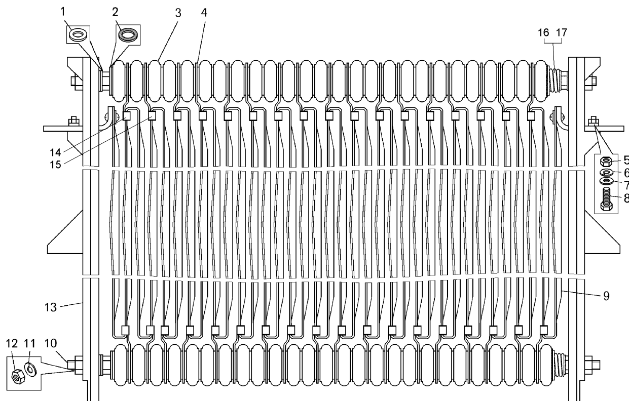
Рисунок 2.5.10 – Секция резистора (75139-2126080-10)
