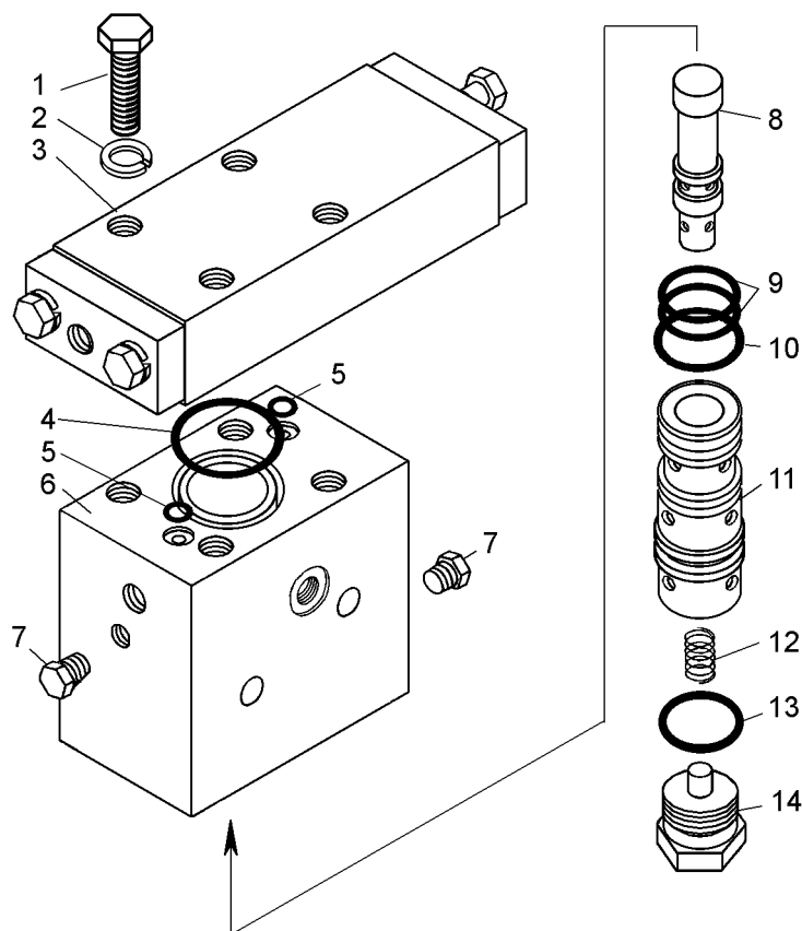
Рисунок 2.19.11 – Автомат разгрузки насоса (75131-3428010)
