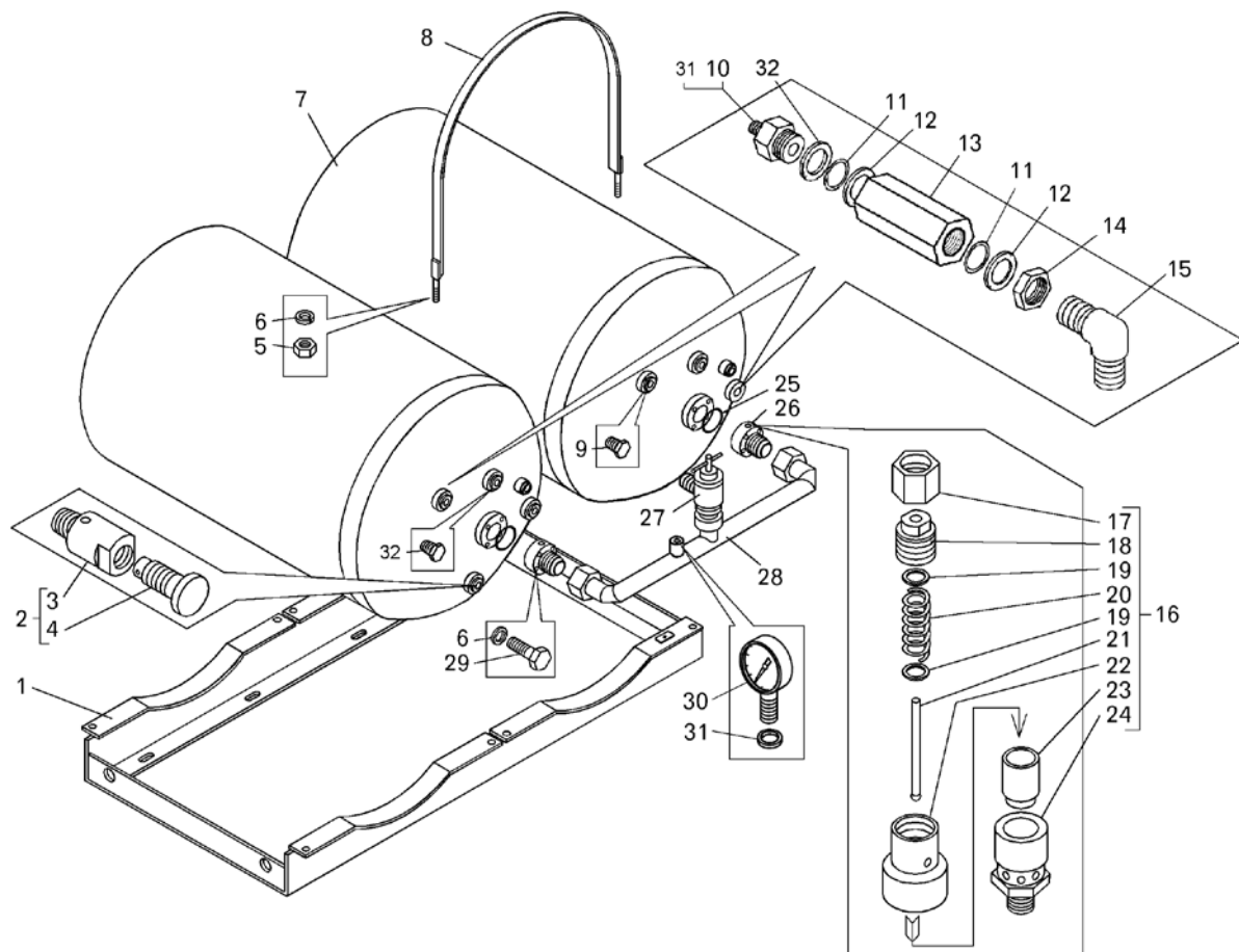
Рисунок 2.1.4 – Баллон воздушный с кронштейном (7513-1031010) Figure 2.1.4 – Air cylinder with bracket
