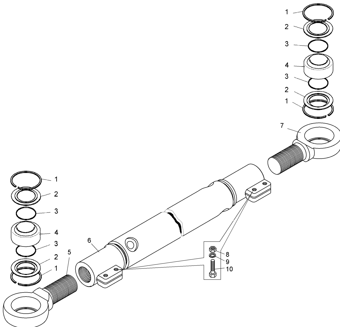
Рисунок 2.10.9 – Тяга рулевой трапеции (75131-3003052-11) Figure 2.10.9 – Steering trapezoid link
