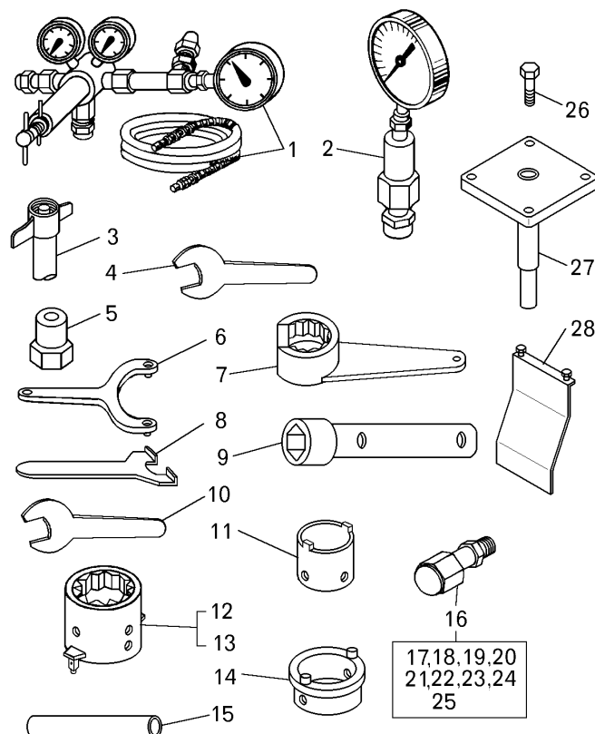
Рисунок 2.14.2 – Инструмент специальный на 5 машин (75131-3900006) Figure 2.14.2 – Special tools for 5 trucks
