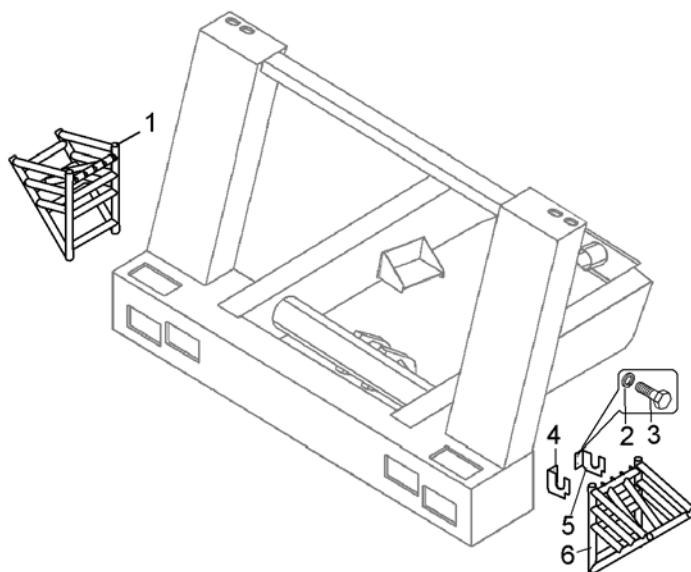
Рисунок 2.15.2 – Установка противооткатных упоров(75131-3927002) Figure 2.15.2 – Mounting of anti-rollback stops
