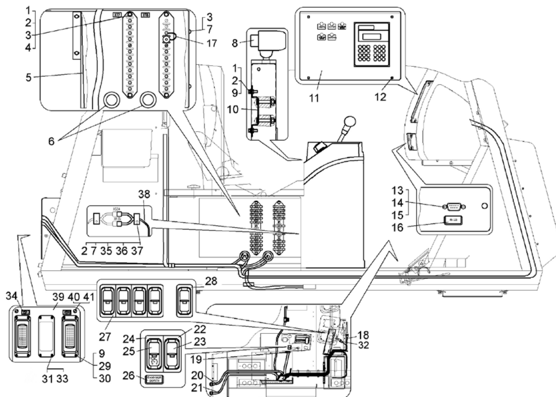
Рисунок 2.5.15 – Монтаж электрооборудования в кабине (75131-2100062-90) Figure 2.5.15 – Mounting of electrical equipment in the cab
