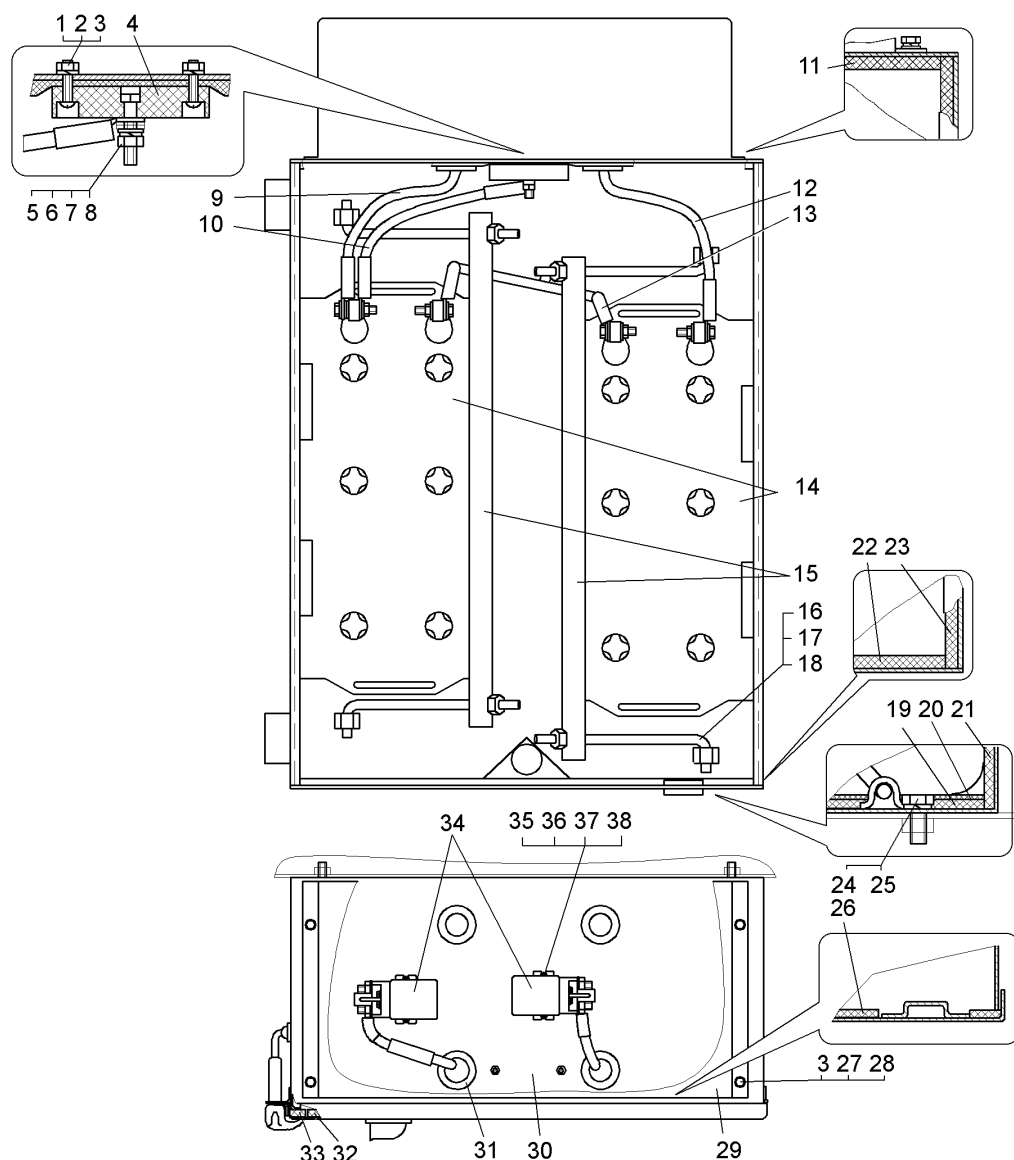
Рисунок 2.13.5 – Установка аккумуляторных батарей и монтаж проводов (75131-3700008-40) Figure 2.13.5 – Installation of storage batteries and cables montage
