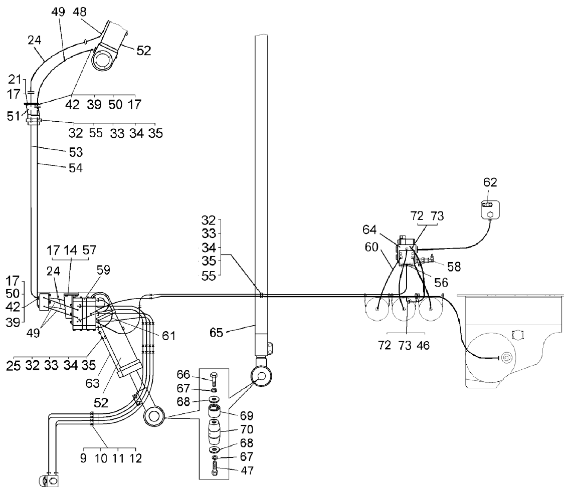
Рисунок 2.10.14 – Трубопроводы рулевого управления (вид II – продолжение рисунка 2.10.13) Figure 2.10.14 – Steering pipelines (view II - continuation of figure 2.10.13)
