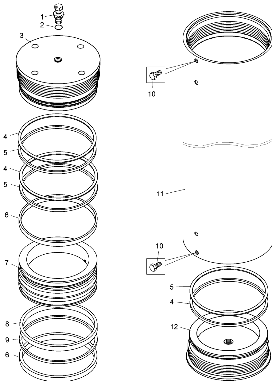
Рисунок 2.11.7 – Пневмогидроаккумулятор (75450-3415010) Figure 2.11.7 – Pneumatic hydroaccumulator
