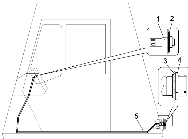
Рисунок 2.13.7 – Монтаж проводов системы смазки “Lincoln” в кабине (75137-3700051)
