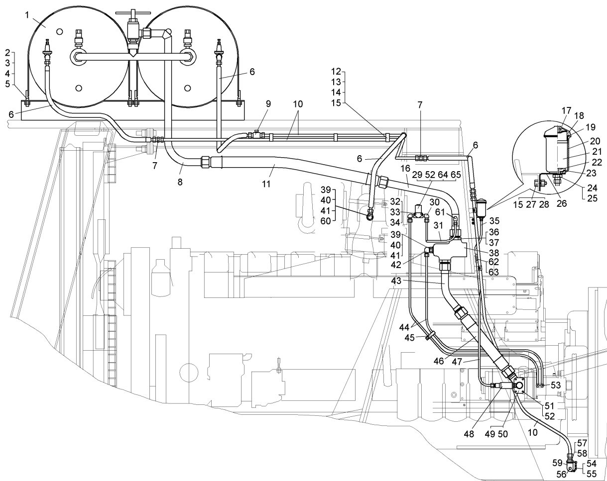
Рисунок 2.1.3 – Установка системы пневмостартерного пуска двигателя (75131-1000007-10) Figure 2.1.3 – Mounting of engine pneumatic start-up system
