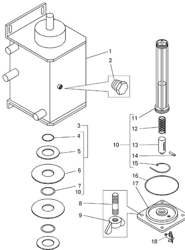
Рисунок 2.2.13 – Обогреватель топлива с фильтром (7512-1138010) Figure 2.2.13 – Fuel heater with filter
