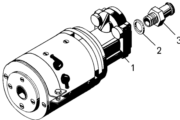
Рисунок 2.2.12 – Насос топливный (7512-1113010) Figure 2.2.12 – Fuel pump
