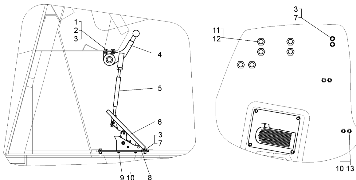
Рисунок 2.2.14 – Установка педали привода управления подачей топлива (75131-1108002-20)
