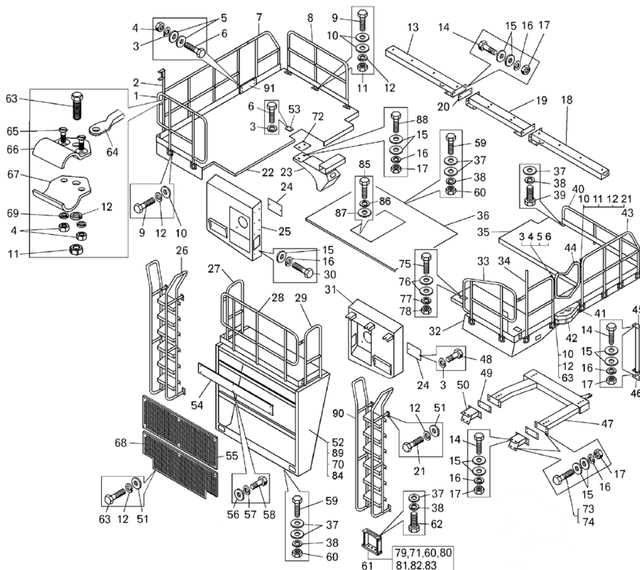
Рисунок 2.16.25 – Капоты и оперение (75131-8400002-31) Figure 2.16.25 – Hoods and fendering
