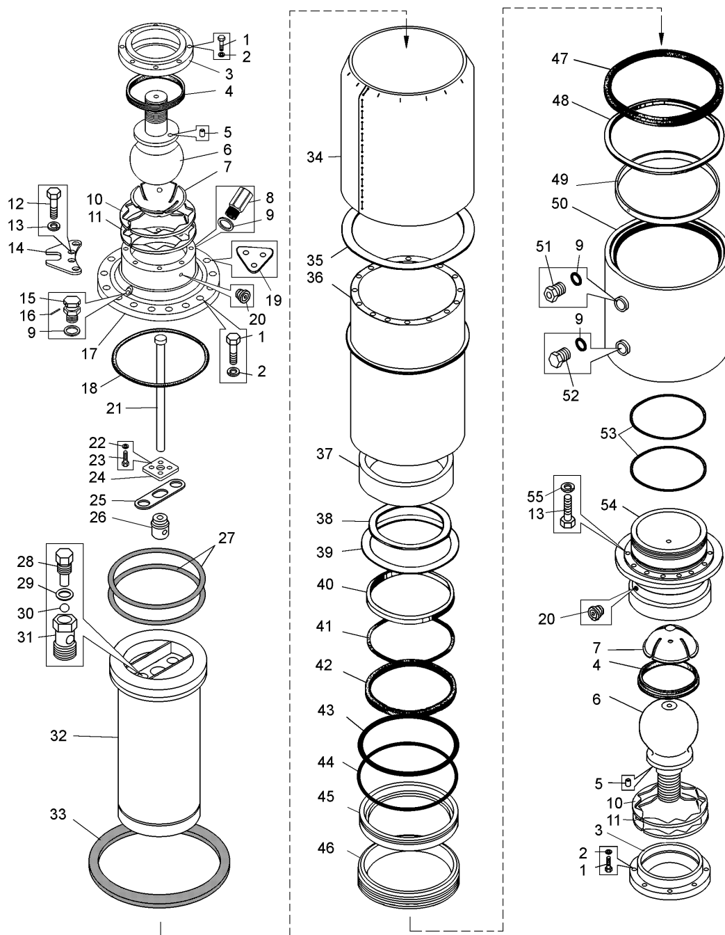
Рисунок 2.8.3 – Цилиндр подвески передний (75131-2907020-11)
