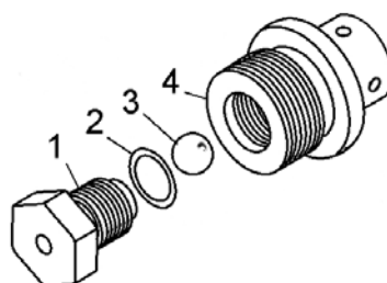
Рисунок 2.10.16 – Клапан обратный с дросселем (7822-3416590-20) Figure 2.10.16 – Check valve with throttle
