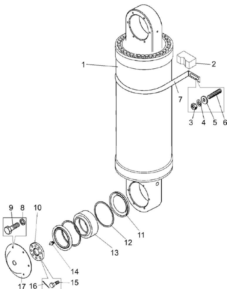
Рисунок 2.19.1 – Установка цилиндров опрокидывающего механизма (75131-8600001) Figure 2.19.1 – Mounting of hoist cylinders
