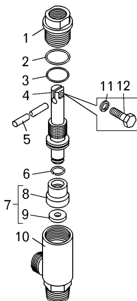
Рисунок 2.1.6 – Кран запорный (75211-1032800-10) Figure 2.1.6 – Stopcock
