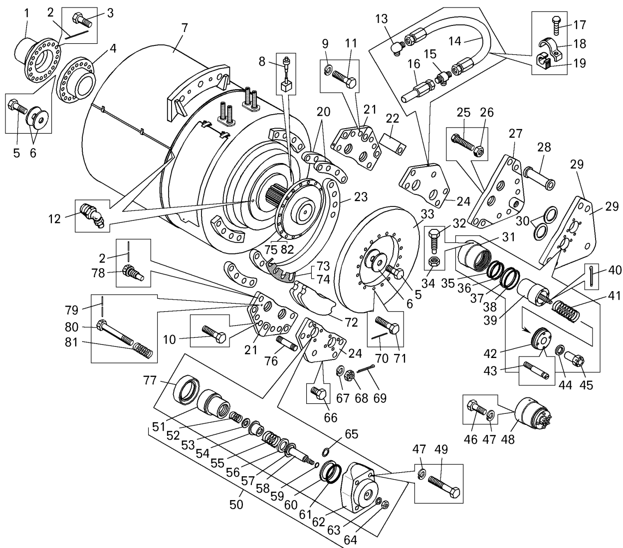
Рисунок 2.6.4 – Электродвигатели тяговые ЭК-420, ЭК-590, ТЭД-6, ЭДП-600 с тормозными механизмами (75132-2103004-01, 75132-2103004-02, 75132-2103004-03, 75132-2103004-06) Figure 2.6.4 – Haul electromotors ЭК-420, ЭК-590, ТЭД-6, ЭДП-600 with brake mechanisms
