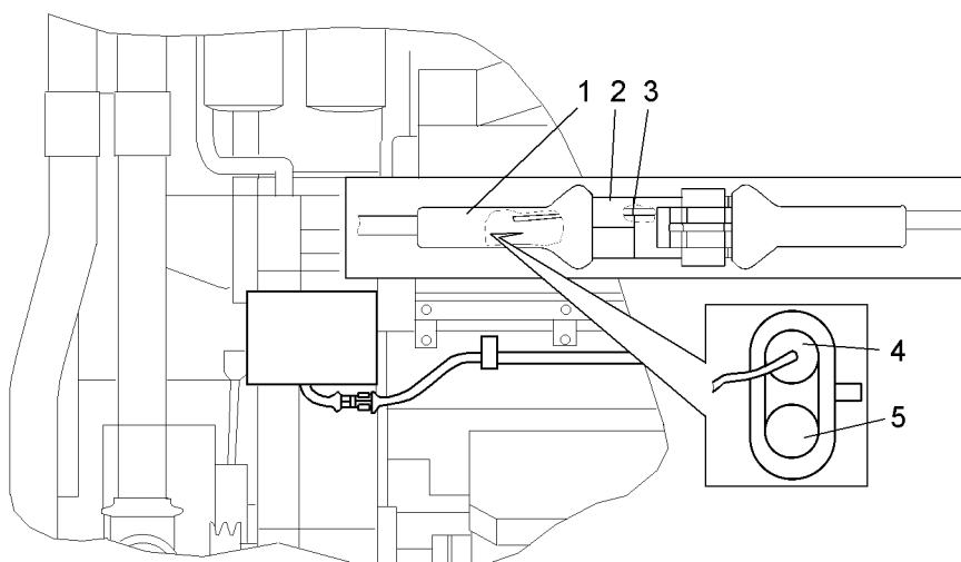
Рисунок 2.13.12 – Подключение компрессора кондиционера (75306-3700076-20) Figure 2.13.12 – Connection of compressor conditioner
