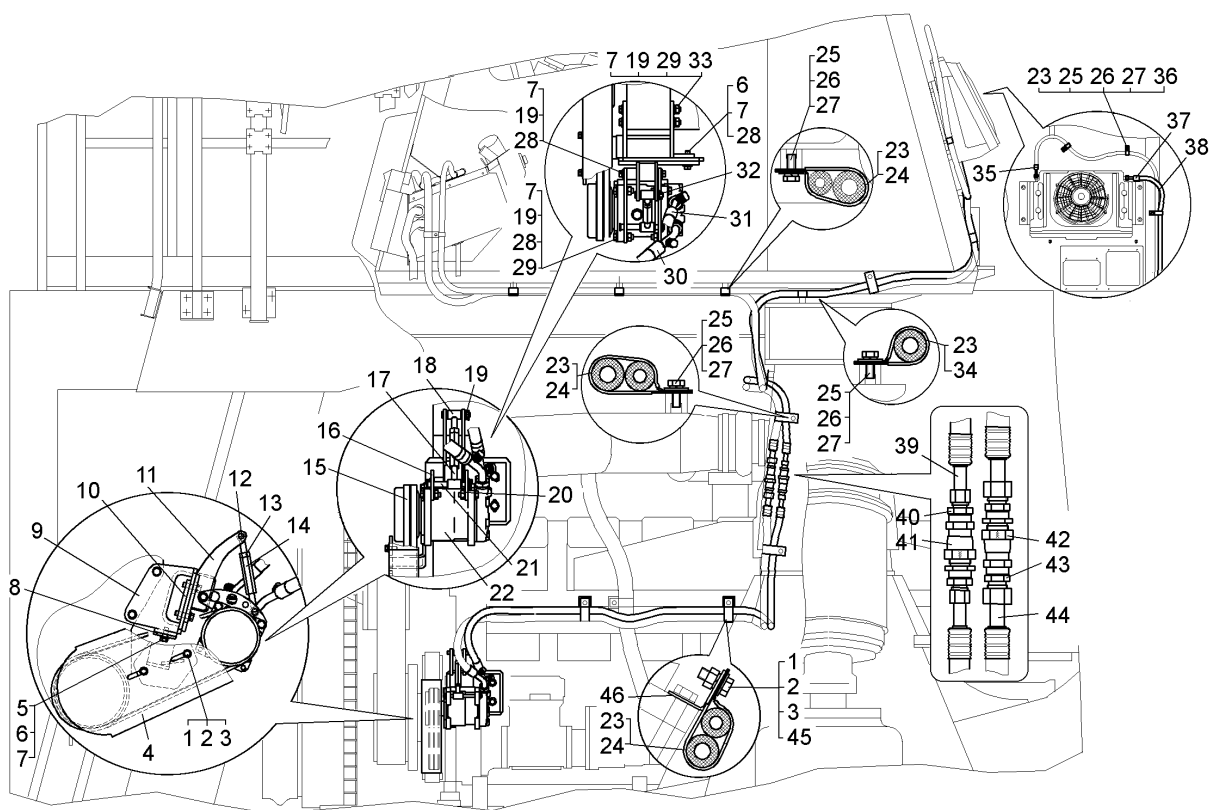
Рисунок 2.16.19 – Установка трубопроводов кондиционера (75131-8100008-50) Figure 2.16.19 – Mounting of conditioner pipelines
