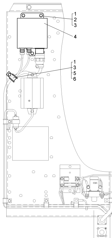
Рисунок 2.13.14 – Монтаж системы контроля давления в шинах по кабине (75310-3700081-10)
