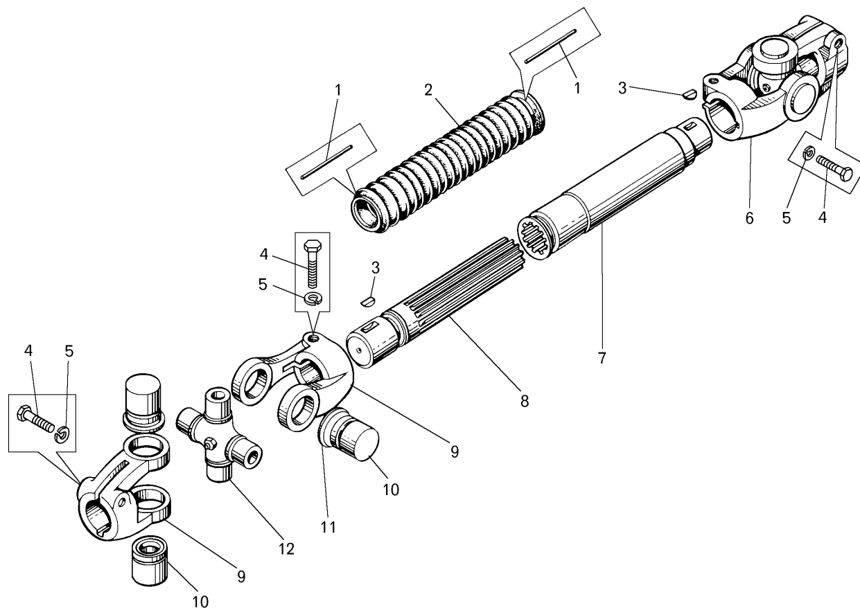
Рисунок 2.10.6 – Вал карданный рулевого управления (7555-3401048) Figure 2.10.6 – Steering cardan shaft
