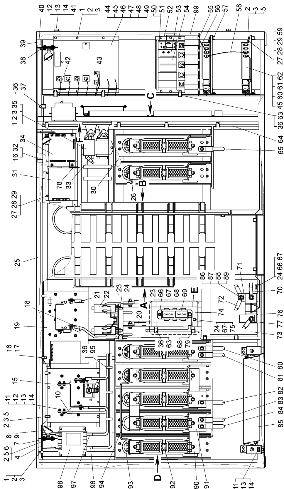
Рисунок 2.5.5 – Шкаф Рисунок– Шкаф с пускорегулирующей аппаратурой (главный вид) (75131-2112010-31) Figure 2.5.5 – Cabinet with start-up control equipment
