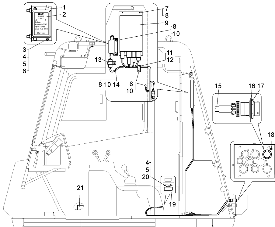
Рисунок 2.17.5 – Установка системы контроля загрузки по кабине (75131-8070003-10) Figure 2.17.5 – Mounting of the load system in the cabin
