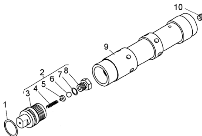
Рисунок 2.10.18 – Золотник усилителя потока (7822-3416530-01) Figure 2.10.18 – Flow booster spool-valve
