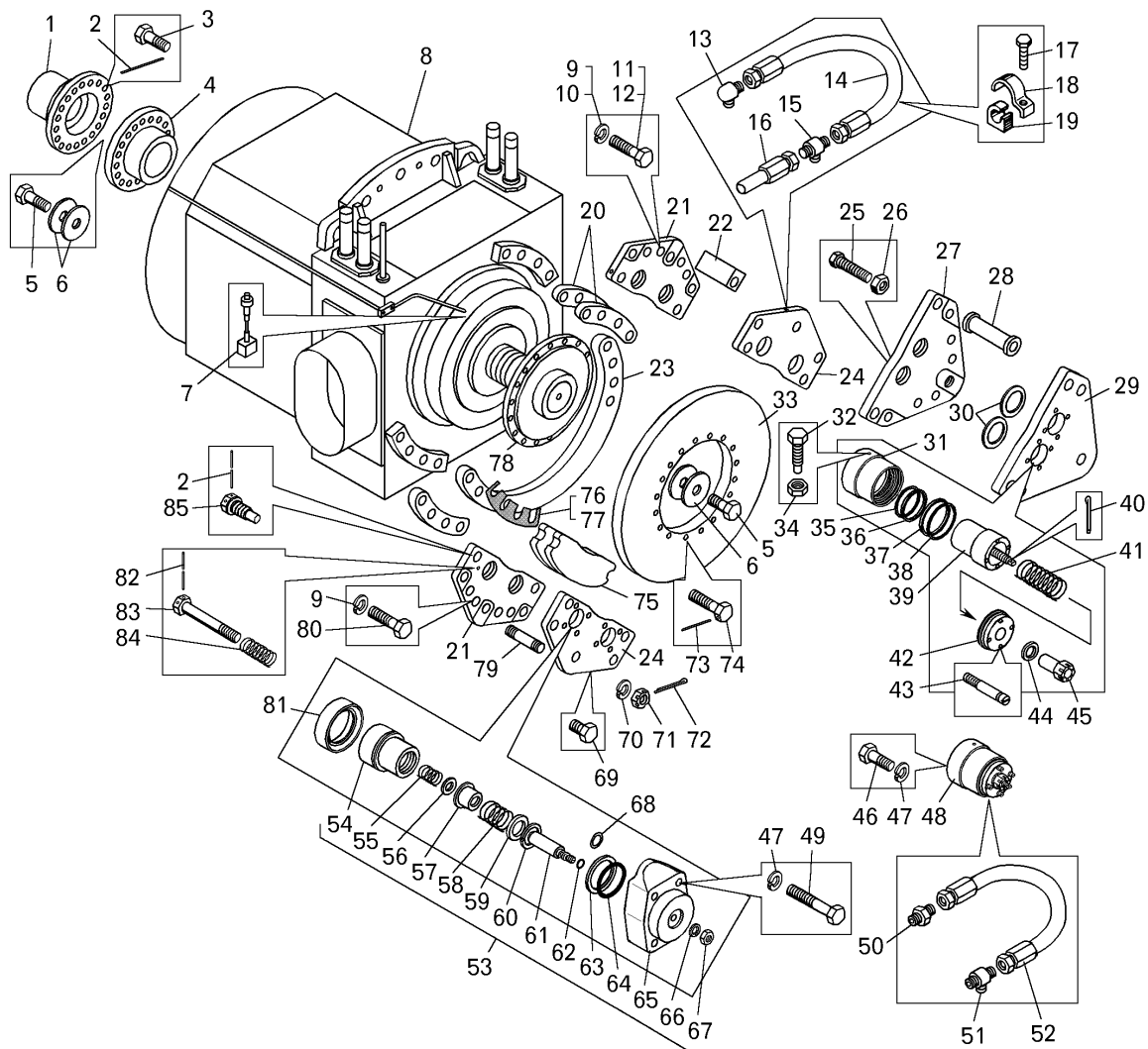
Рисунок 2.6.3 – Электродвигатель тяговый ЭД 136 с тормозными механизмами (75132-2103004) Figure 2.6.3 – Haul electromotor ЭД-136 with brake mechanisms
