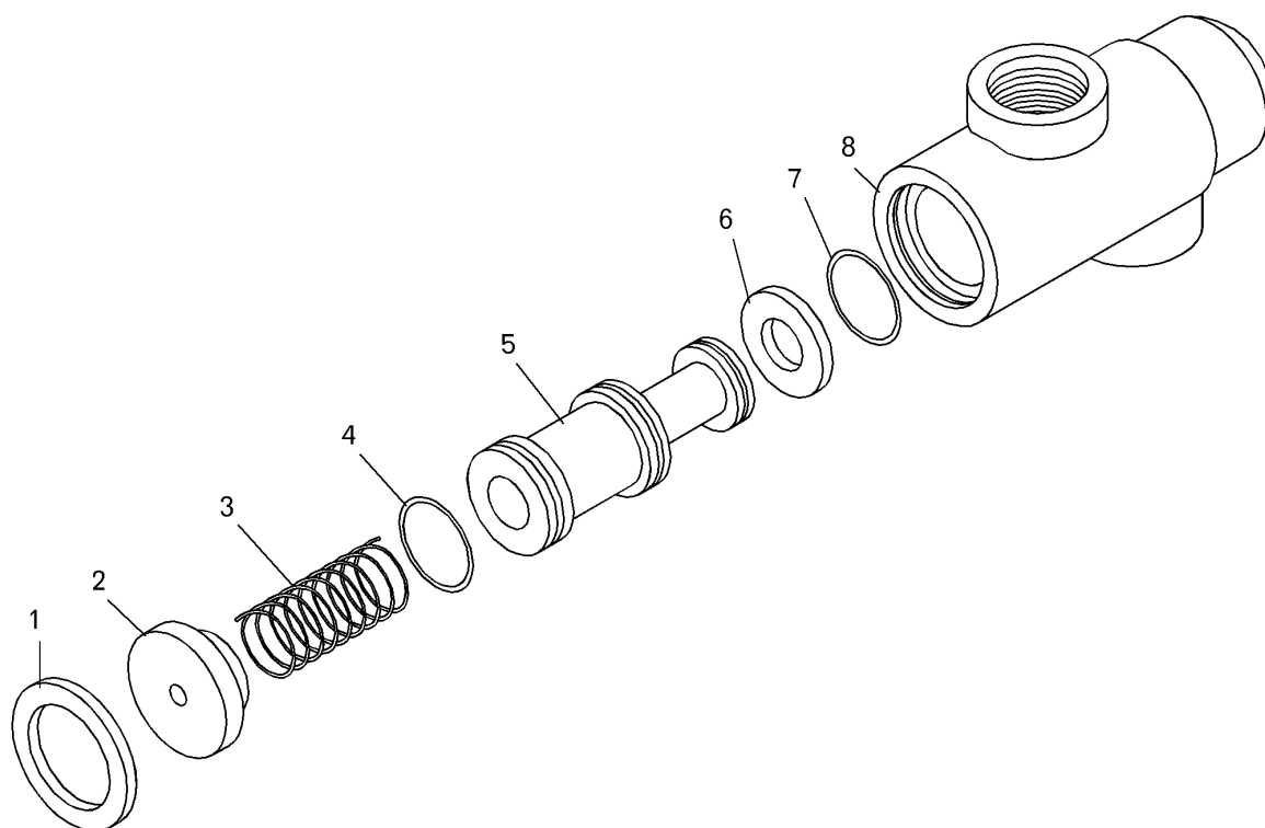
Рисунок 2.1.5 – Клапан пусковой (7549-1032180) Figure 2.1.5 – Starting valve
