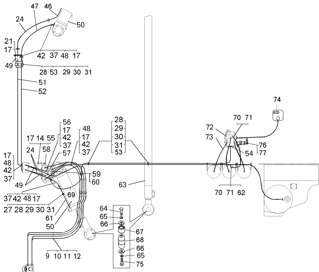
Рисунок 2.10.8 – Трубопроводы рулевого управления (вид II – продолжение рисунка 2.10.7) Figure 2.10.8 – Steering pipelines (view II - continuation of figure 2.10.7)
