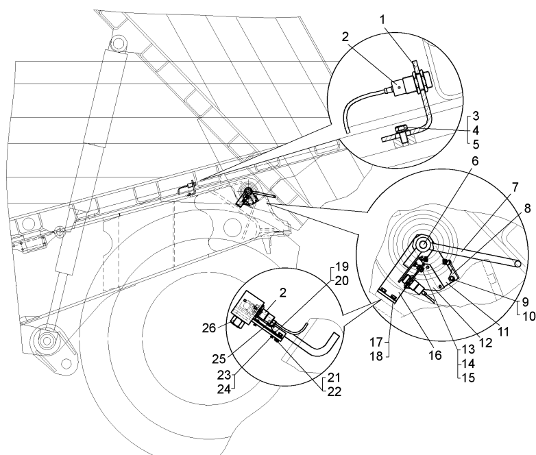
Рисунок 2.19.20 – Установка выключателя (75131-8606002-10) и датчика положения платформы (7513-8601002)
