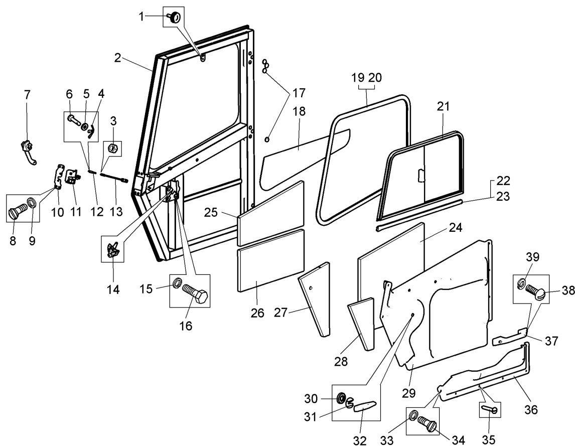
Рисунок 2.16.6 – Дверь кабины (7555В-6100010-10, 7555В-6100011-10)
