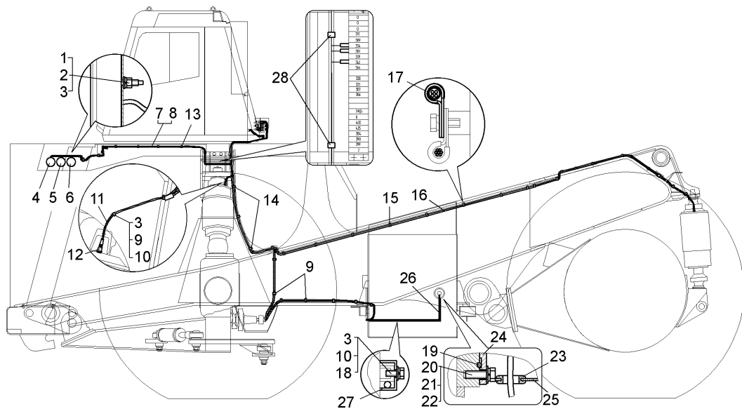
Рисунок 2.17.4 – Установка системы контроля загрузки по шасси (75131-8070002-70) Figure 2.17.4 – Mounting of the load system over chassis
