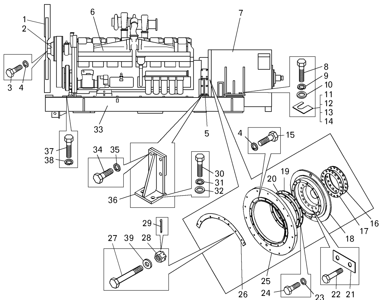
Рисунок 2.1.2 – Дизель – генератор (75131-1000004-25, 75131-1000004-26, 75131-1000004-27) Figure 2.1.2 – Diesel generator
