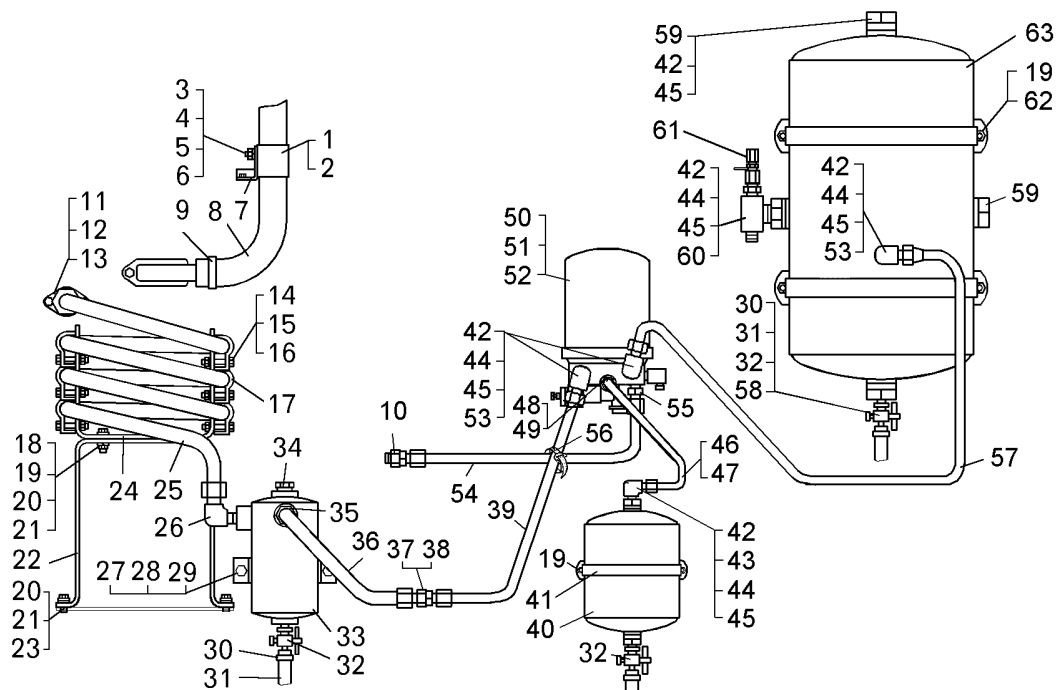
Рисунок 2.12.1 – Монтаж трубопроводов компрессора (75131-3500016-10) Figure 2.12.1 – Mounting of compressor pipelines
