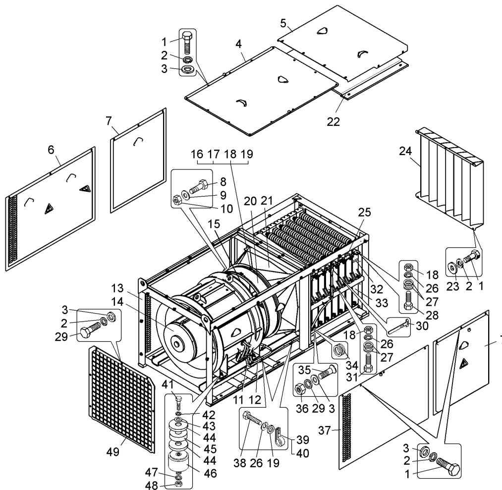
Рисунок 2.5.8 – Вентилируемая тормозная установка (75139-2126004, 75139-2126004-01) Figure 2.5.8 – Vented brake unit
