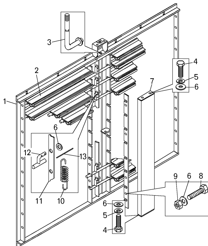
Рисунок 2.4.6 – Жалюзи радиатора (75131-1310110-10) Figure 2.4.6 – Radiator shutters
