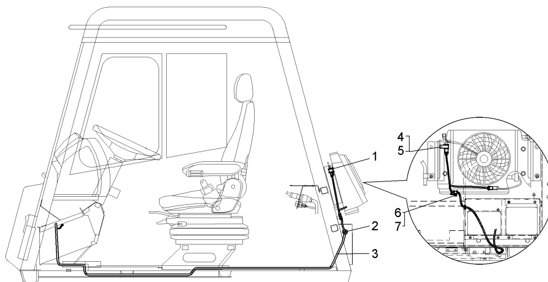
Рисунок 2.13.11 – Монтаж проводов кондиционера (75137-3700072-10)
