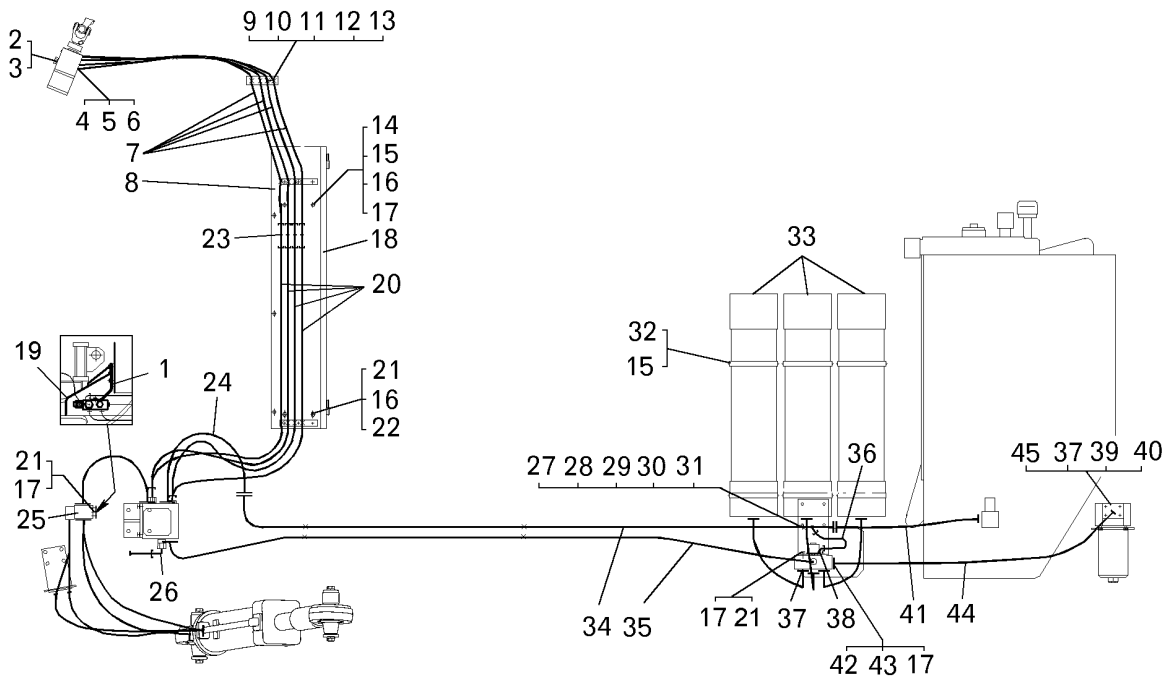
Рисунок 2.10.7 – Трубопроводы рулевого управления (вид I), (75131-3400001-30) Figure 2.10.7 – Steering pipelines (view I)
