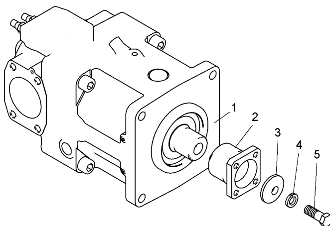
Рисунок 2.19.15 – Насос (75131-8604011-20) Figure 2.19.15 – Pump
