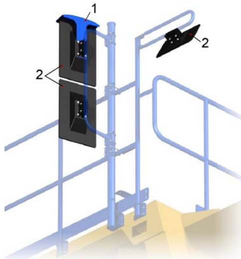
Рисунок 2.16. 21 – Установка зеркал заднего вида правого крыла (75306-8201005-10) Figure 2.16. 21 – Mounting of rear view mirrors
