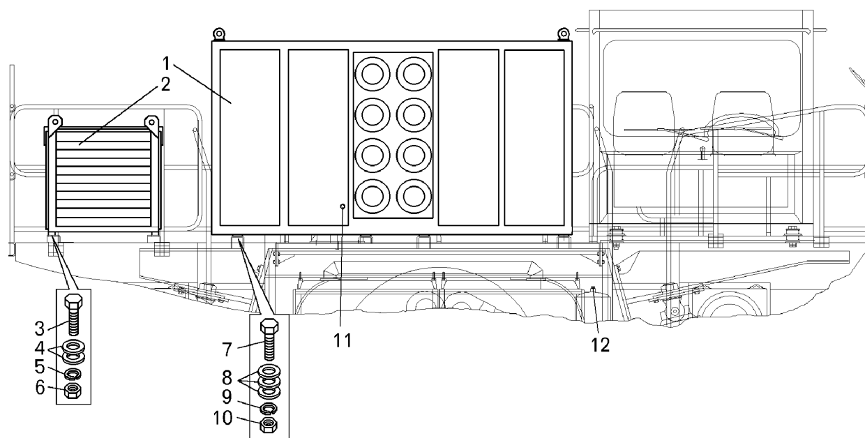
Рисунок 2.5.2 – Установка электрооборудования (75131-2100022-31) Figure 2.5.2 – Mounting of electrical equipment
