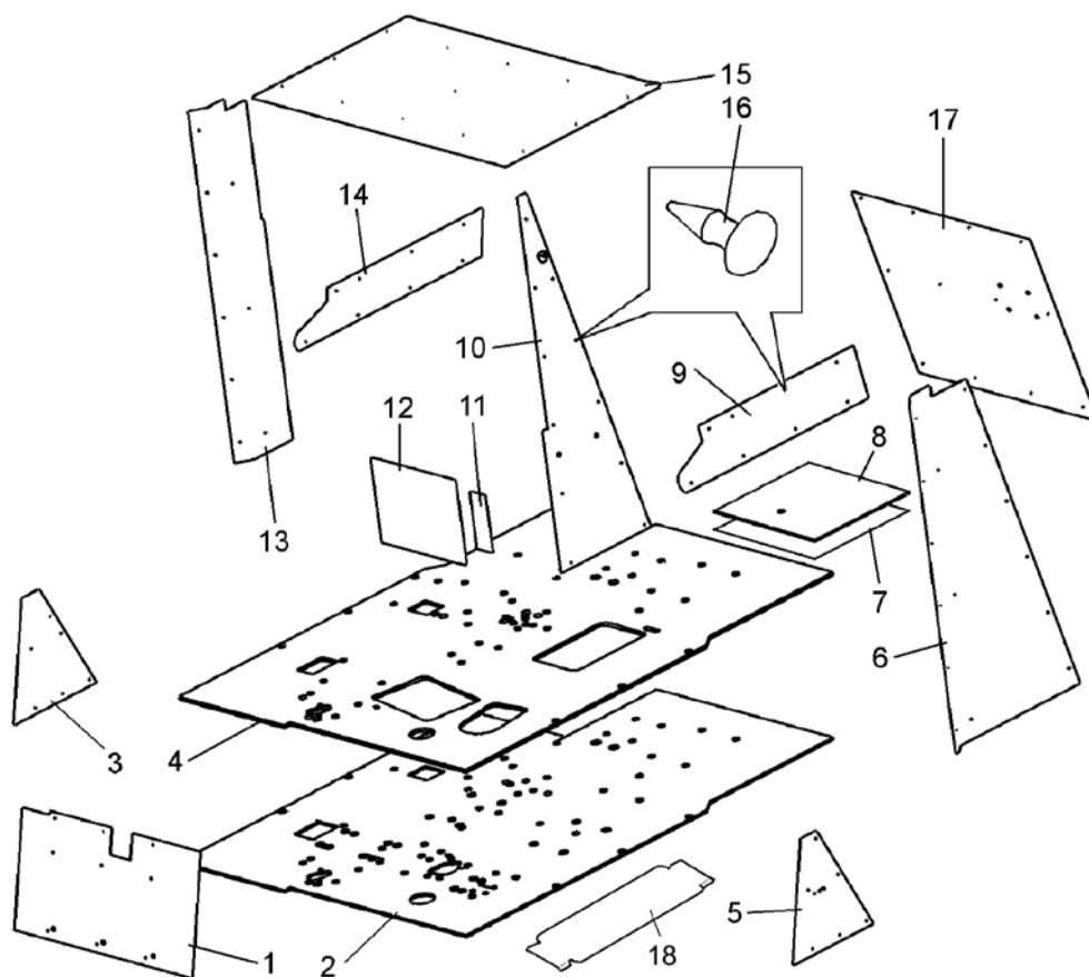
Рисунок 2.16.5 – Кабина. (75306-5000012-40). Установка декоративных панелей Figure 2.16.5 – Cabin. Mounting of decorative panels
