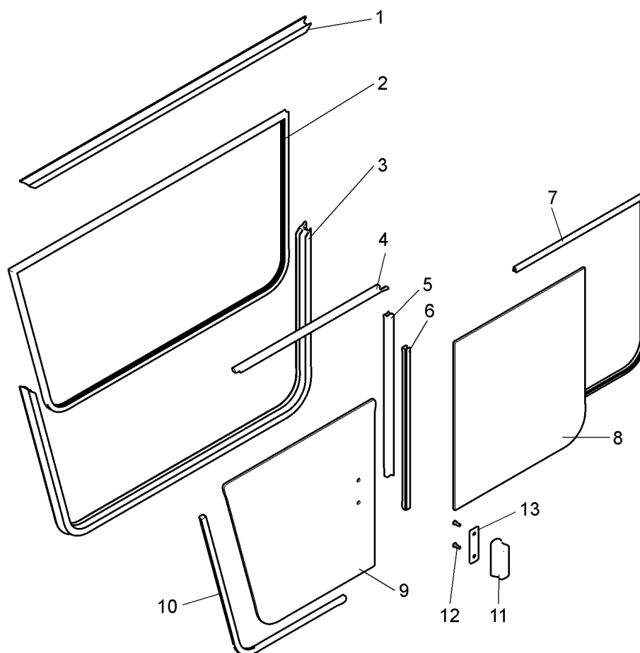
Рисунок 2.16.7 – Окно раздвижное (7555B-5403010, 7555B-5403011) Figure 2.16.7 – Sliding window
