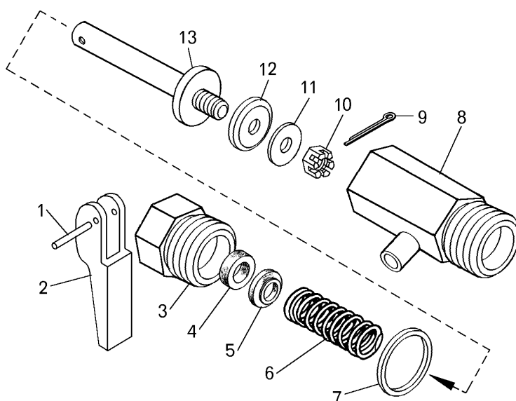
Рисунок 2.4.3 – Кран сливной (549A-1305010) Figure 2.4.3 – Drain cock
