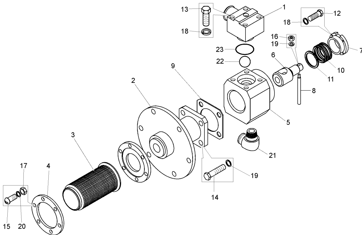
Рисунок 2.2.5 – Кран топливный с фильтром (75131-1116010) Figure 2.2.5– Fuel cock with filter
