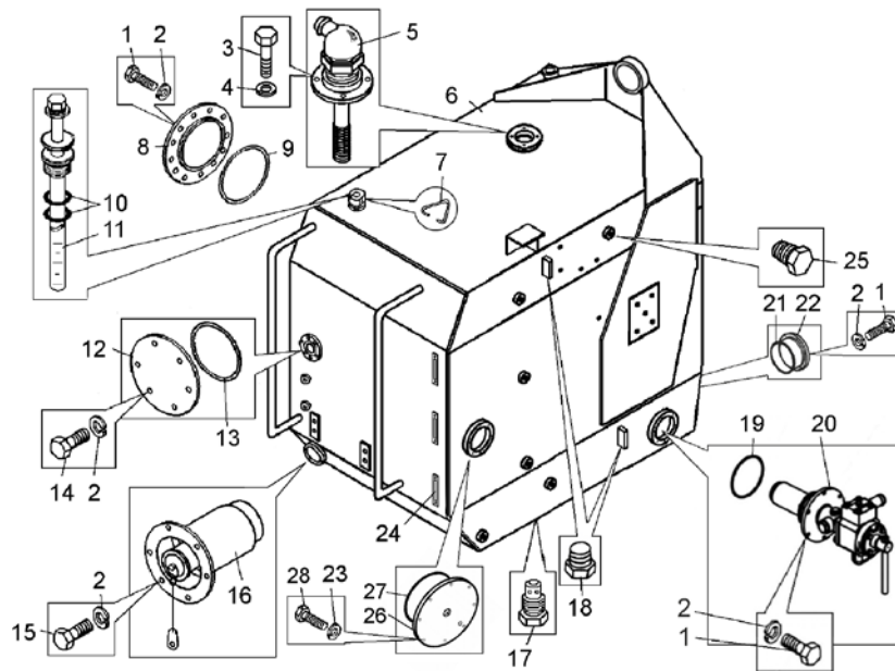
Рисунок 2.2.4 – Бак топливный (75131-1101010-43)
