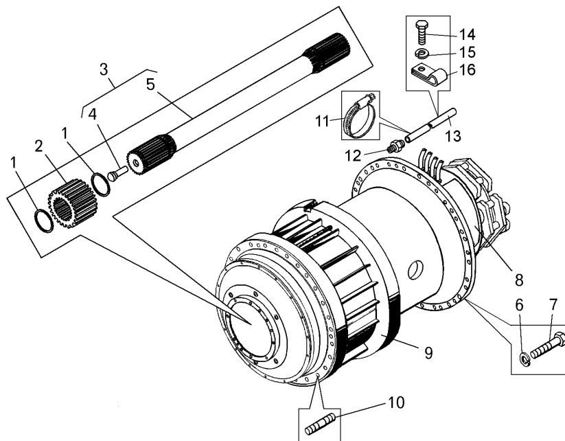
Рисунок 2.6.2 – Электродвигатель-колесо (75132-3112010, 75132-3112010-01, 75132-3112010-02, 75132-3112010-03, 75132-3112010-06)
