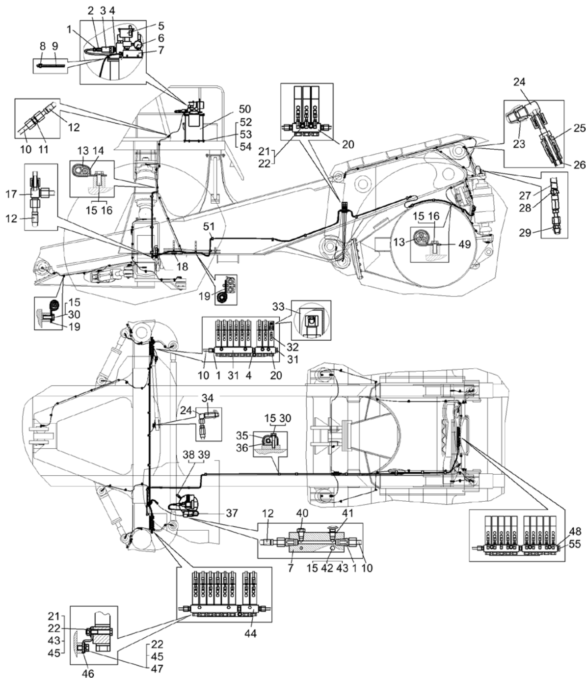
Рисунок 2.15.4 – Установка централизованной системы смазки "Graco" (7513-6600030-30) Figure 2.15.4 – Centralized lubrication system arrangement chart "Graco"
