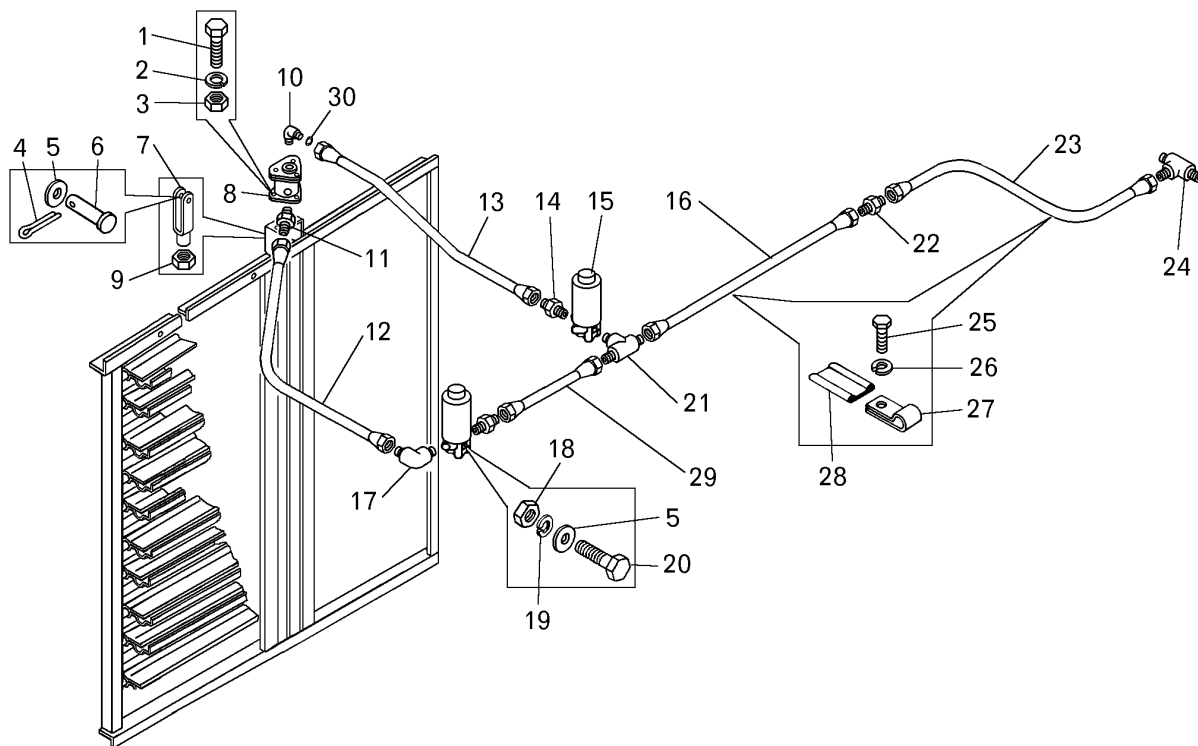
Рисунок 2.4.4 – Установка привода жалюзи радиатора (75131-1300015)
