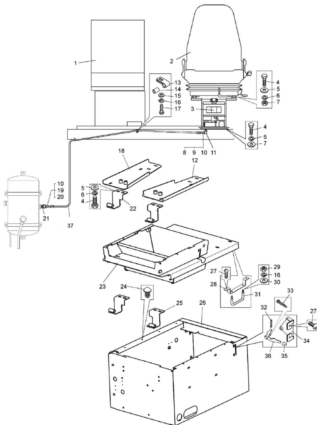
Рисунок 2.16.13 – Установка сидений и трубопроводов (7555В-6800006-20, 75131-6800008) Figure 2.16.13 – Mounting of seats and pipelines
