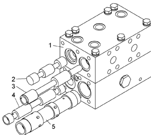
Рисунок 2.10.17 – Корпус с золотниками (75131-3416606) Figure 2.10.17 – Body with spool-valves
