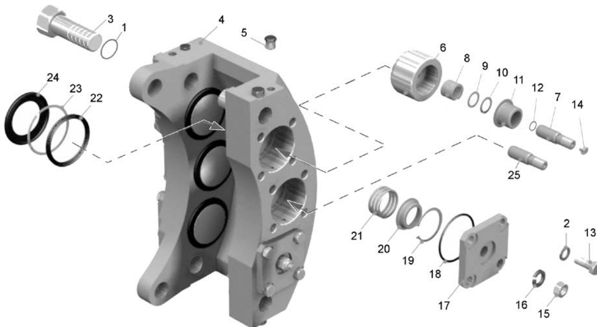
Рисунок 2.9.3 – Корпус тормоза (75570-3501080-10) Figure 2.9.3 – Brake body
