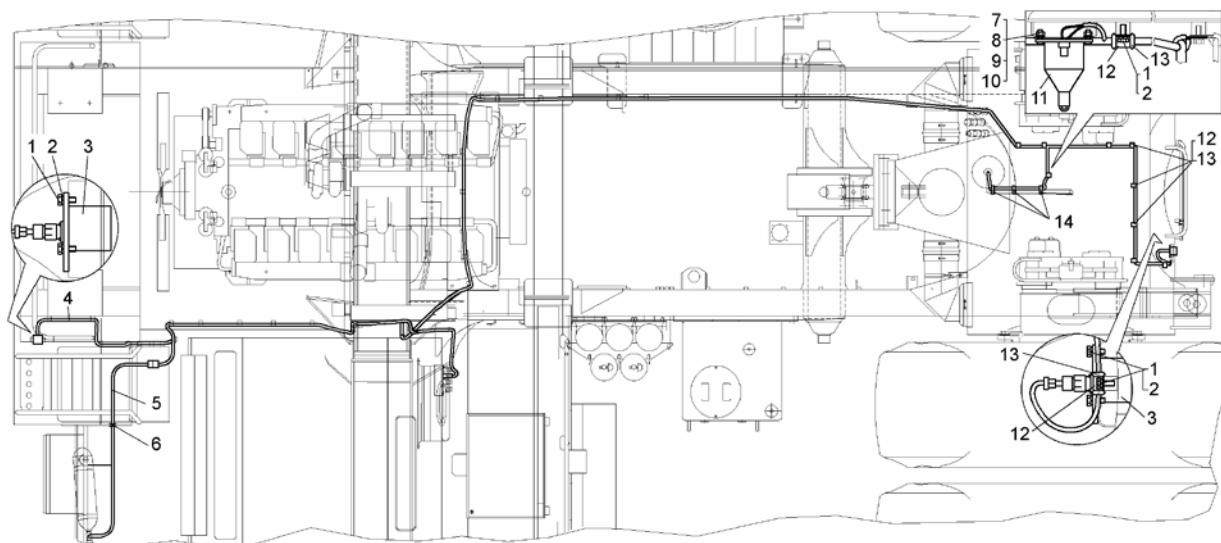
Рисунок 2.13.18 – Монтаж электрооборудования системы пожаротушения по шасси (75131-3767010-10) Figure 2.13.18 – Arrangement of wiring of fire fighting system on chassis
