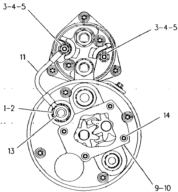
VIEW A-A
