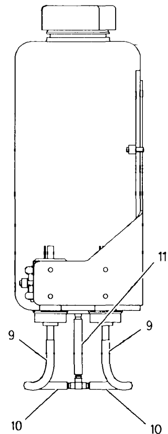
SECTION A-A
