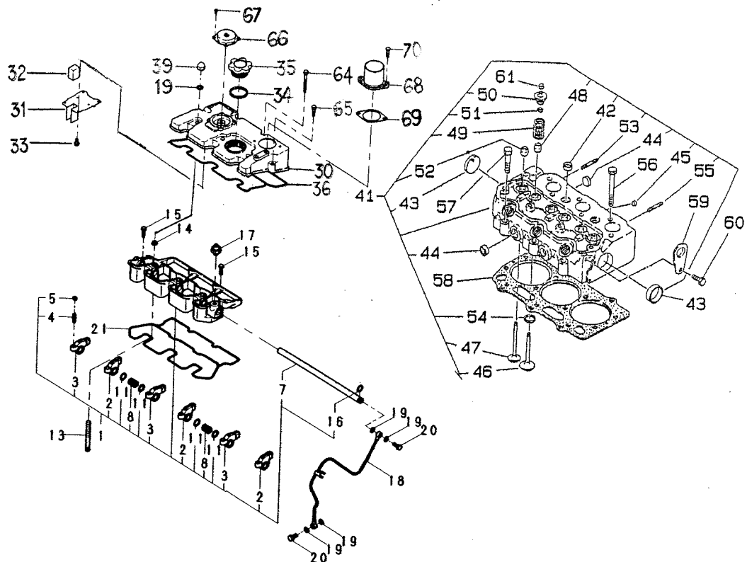
FIG.103 シリンダヘッド, ロッカーアーム CYLINDER HEAD, ROCKER ARM
