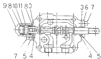
FIG.229 アタッチメントバルブ；二連 ATTACHMENT VALVE ; 2-SPOOL
