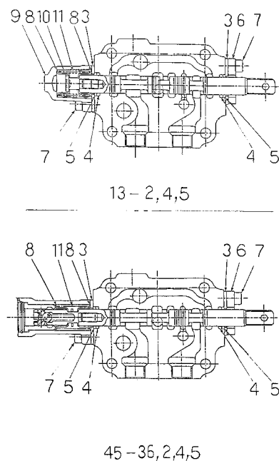
アタッチメントバルブ；二連 ATTACHMENT VALVE ; 2-SPOOL
