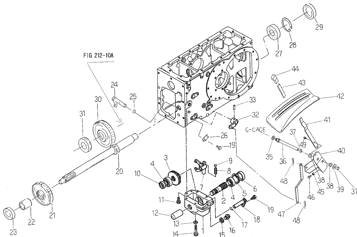
FIG.211 ミッド PTO MID P. T. O
