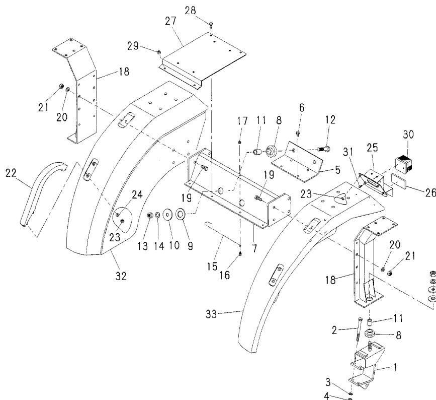
安全フレーム FIG.215 SAFETY FRAME
