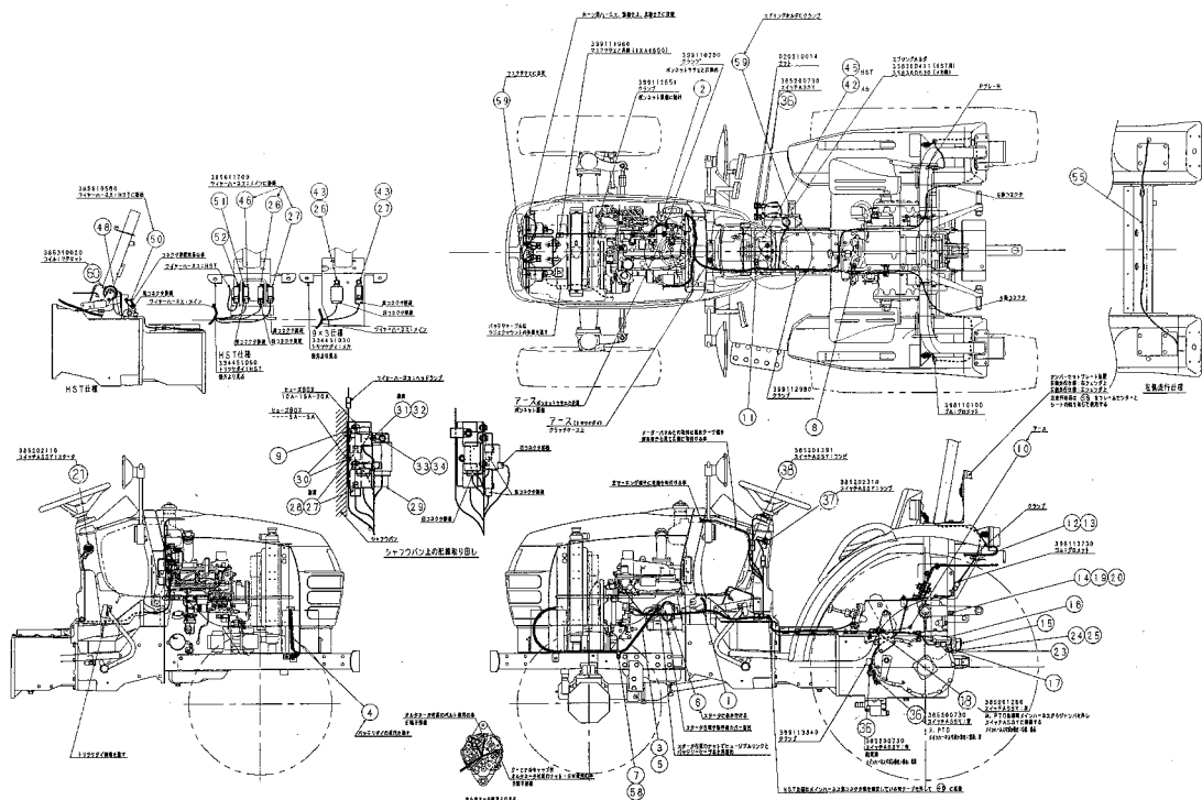
FIG.240 電装品関係 ELECTRICAL GROUP
