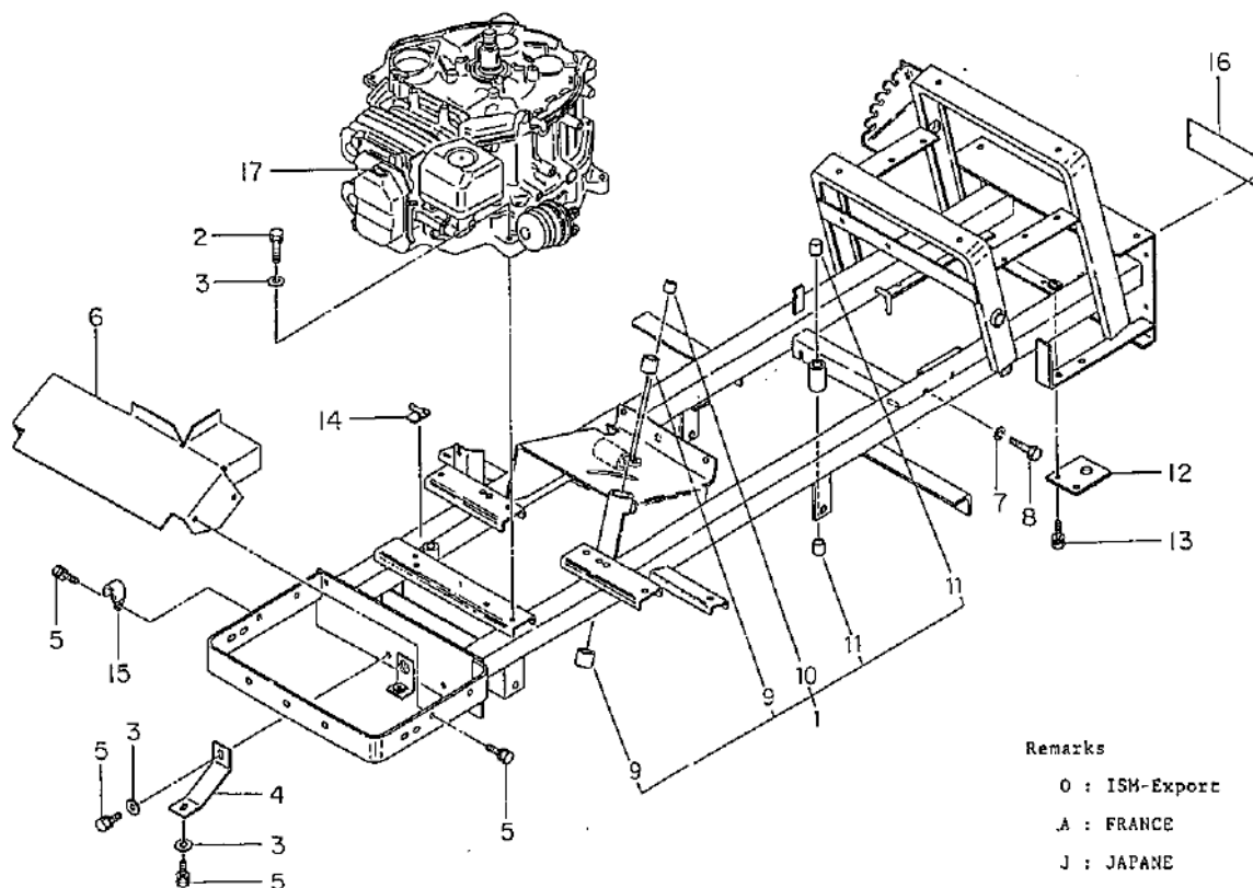
FIG.201 シャーシ CHASSIS ; LT 14
