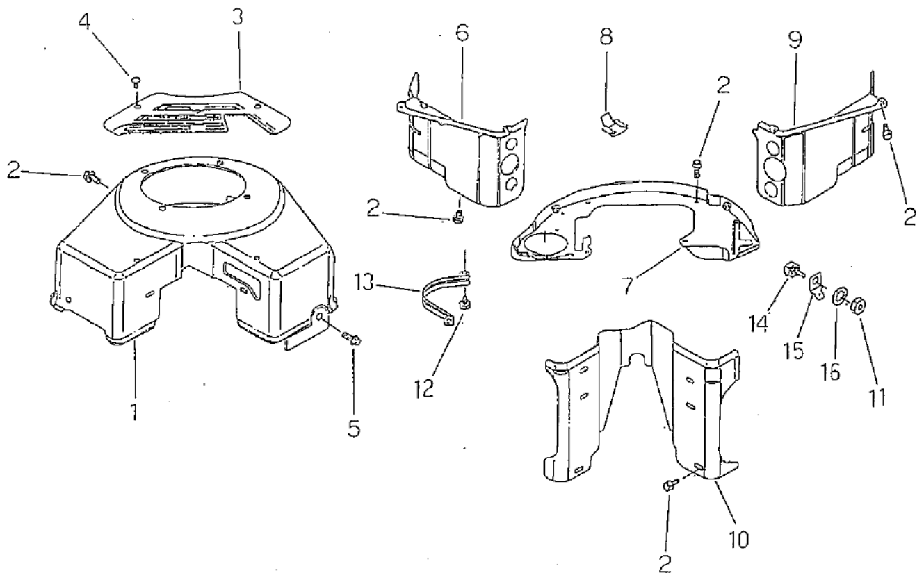
FIG.116 クーリングカバー, マフラ COOLING COVER, MUFFLER
