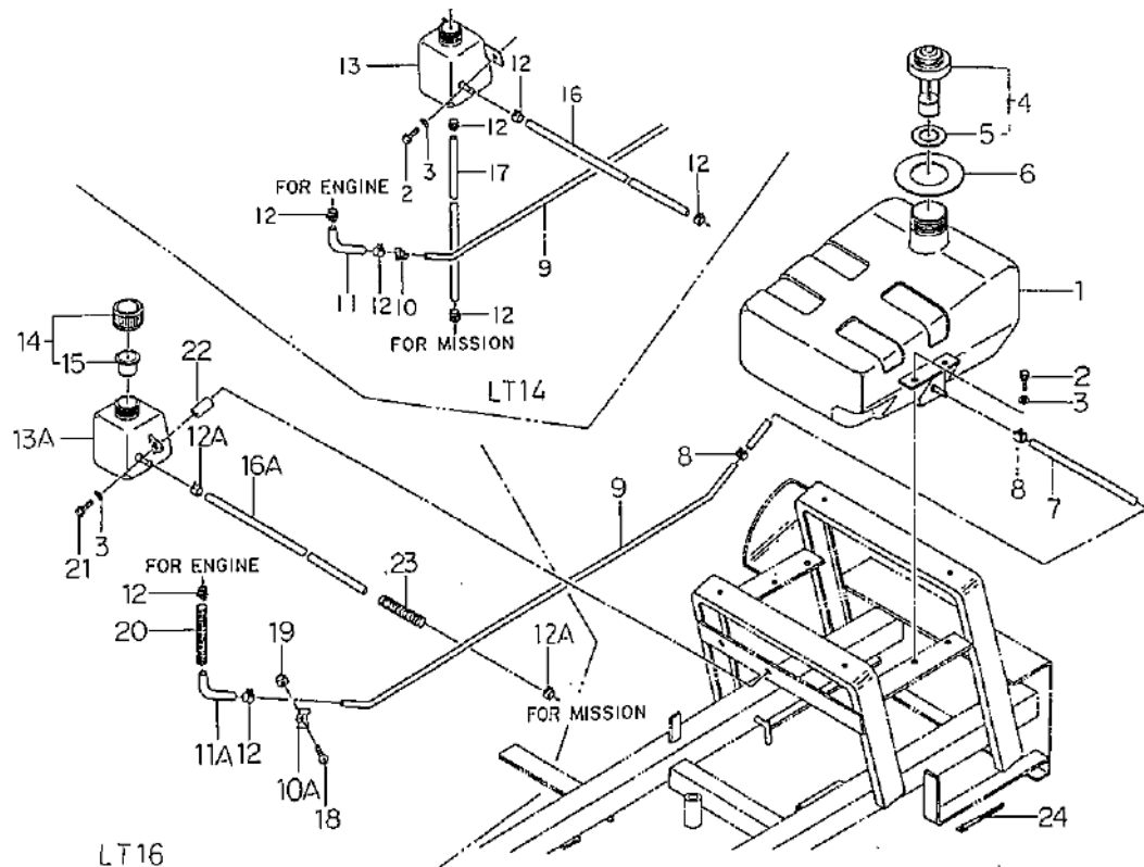
FIG.206 フューエルタンク, オイルタンク FUEL TANK, OIL TANK
