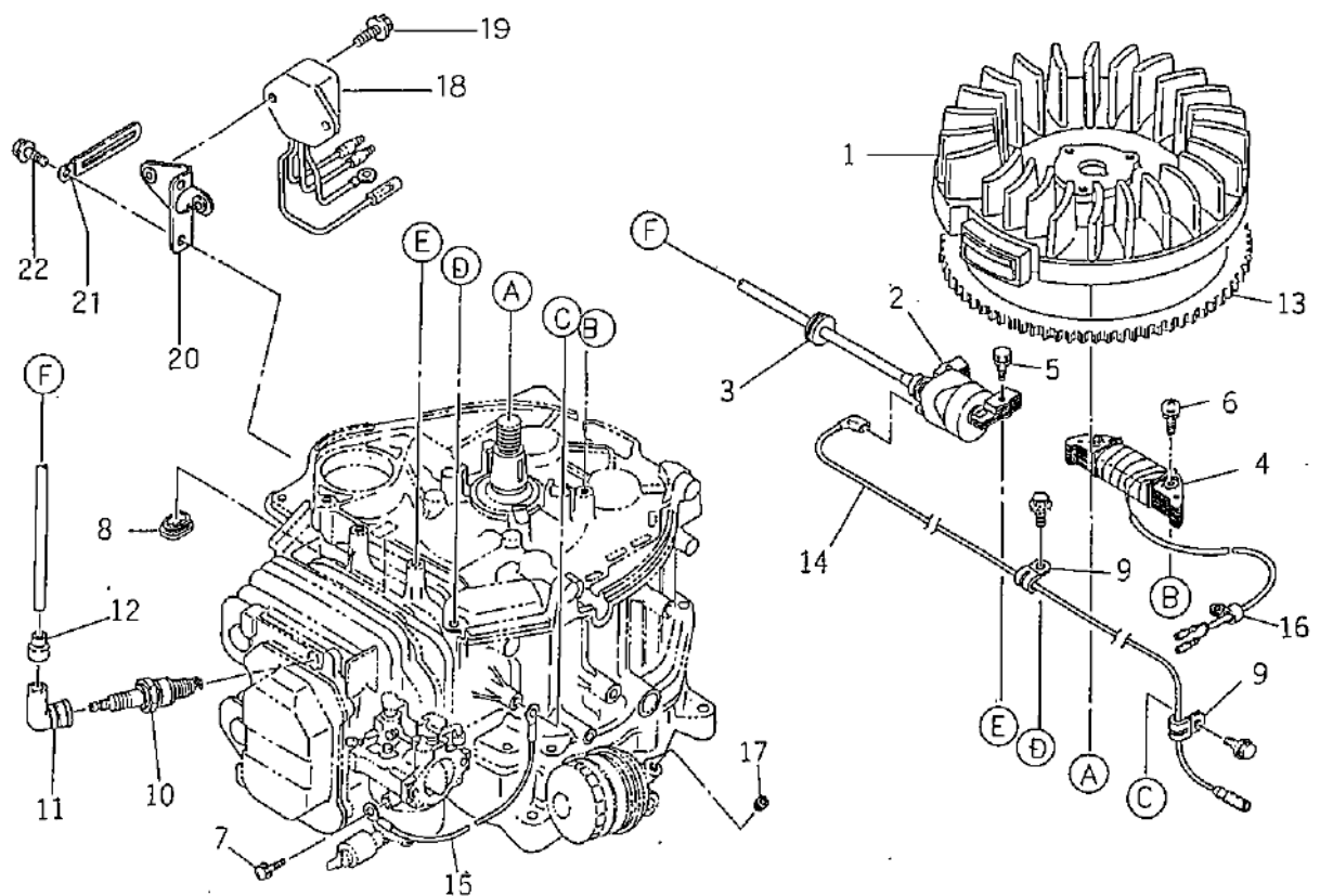
https://truck-manuals.com/ イグニッションデバイス FIG.107 IGNITION DEVICE
