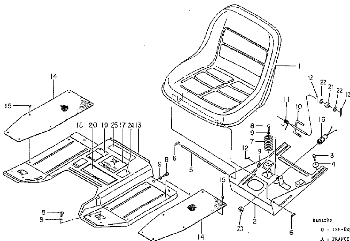
FIG.213 シート, ステップ SEAT, STEPS
