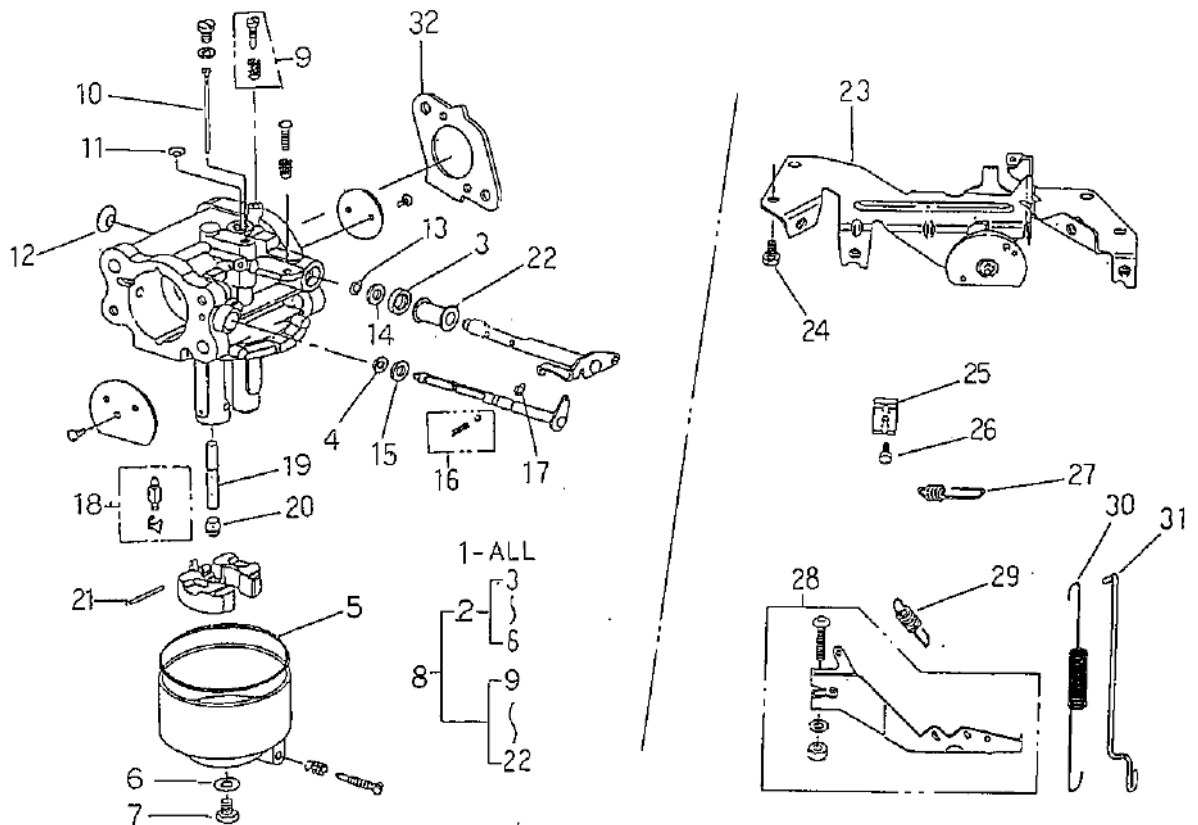
FIG.114 キャブレータ, ガバナ CARBURETER, GOVERNOR
