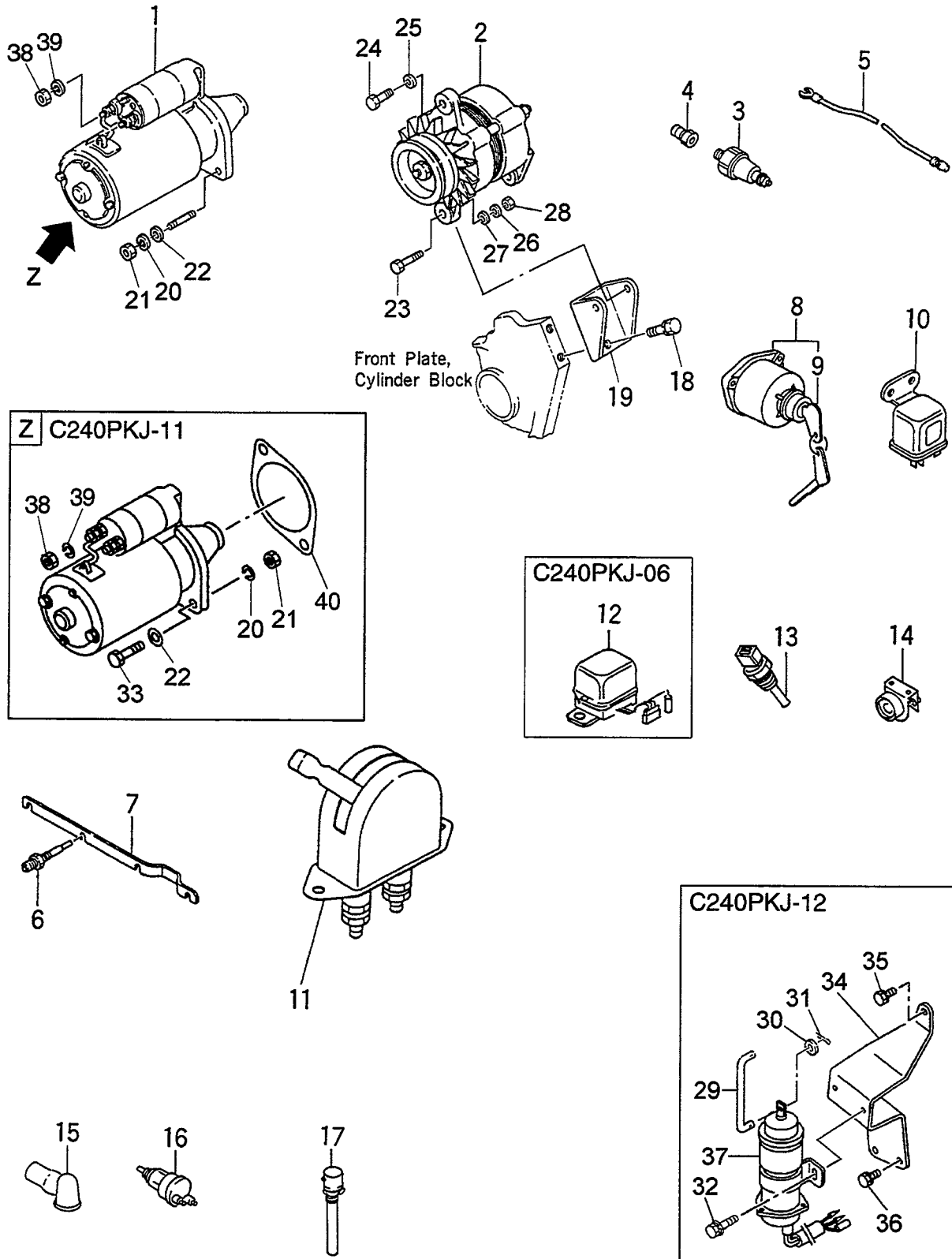
FIG. 27 STARTER, GENERATOR & ELECTRICAL PARTS スタータ、ジェネレータ&エレクトリカルパーツ
