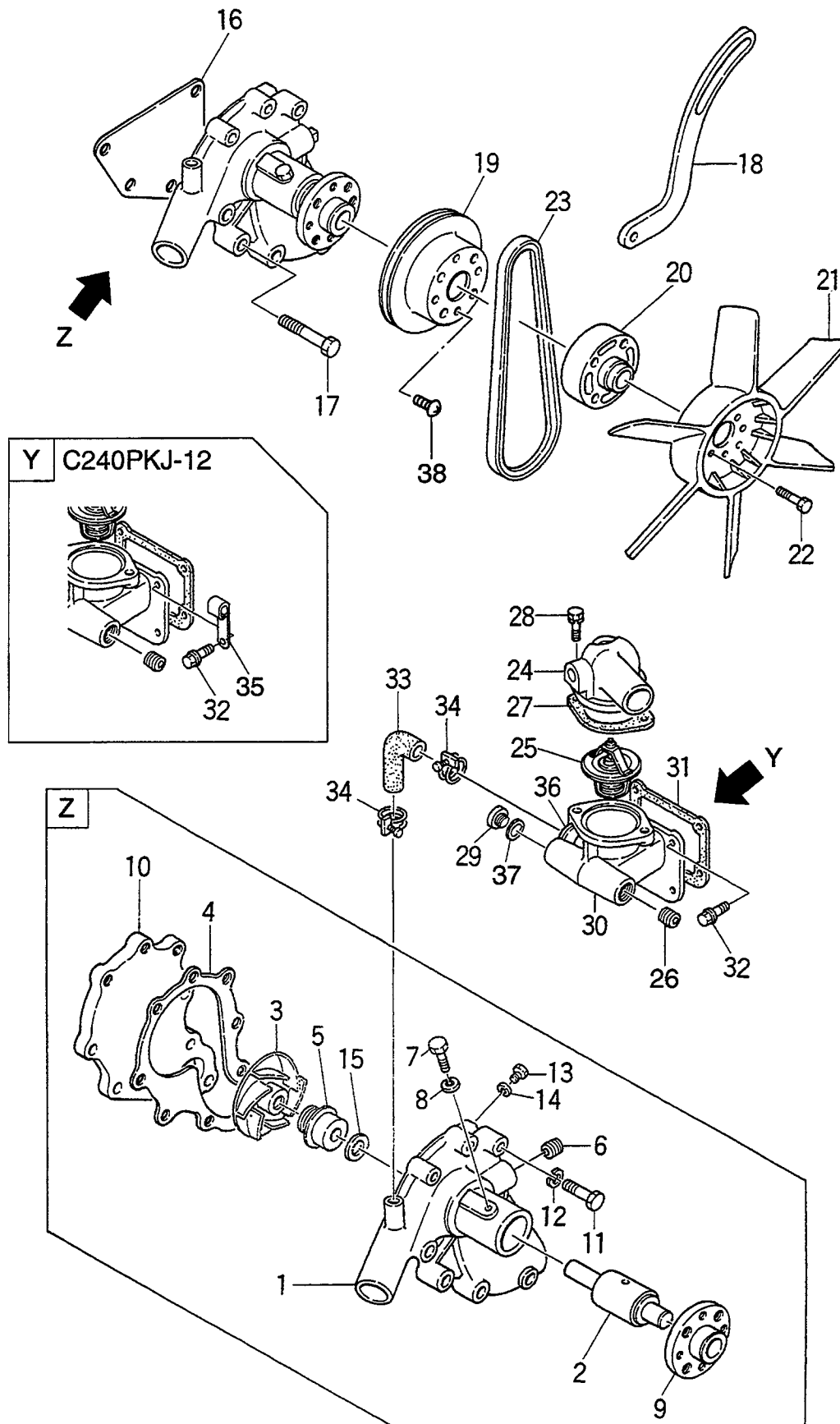
FIG. 15 COOLING SYSTEM クーリングシステム
