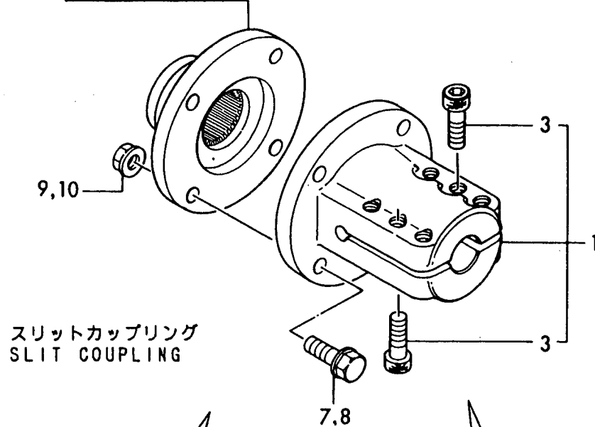
Fig. 55 カップリング COUPLING
