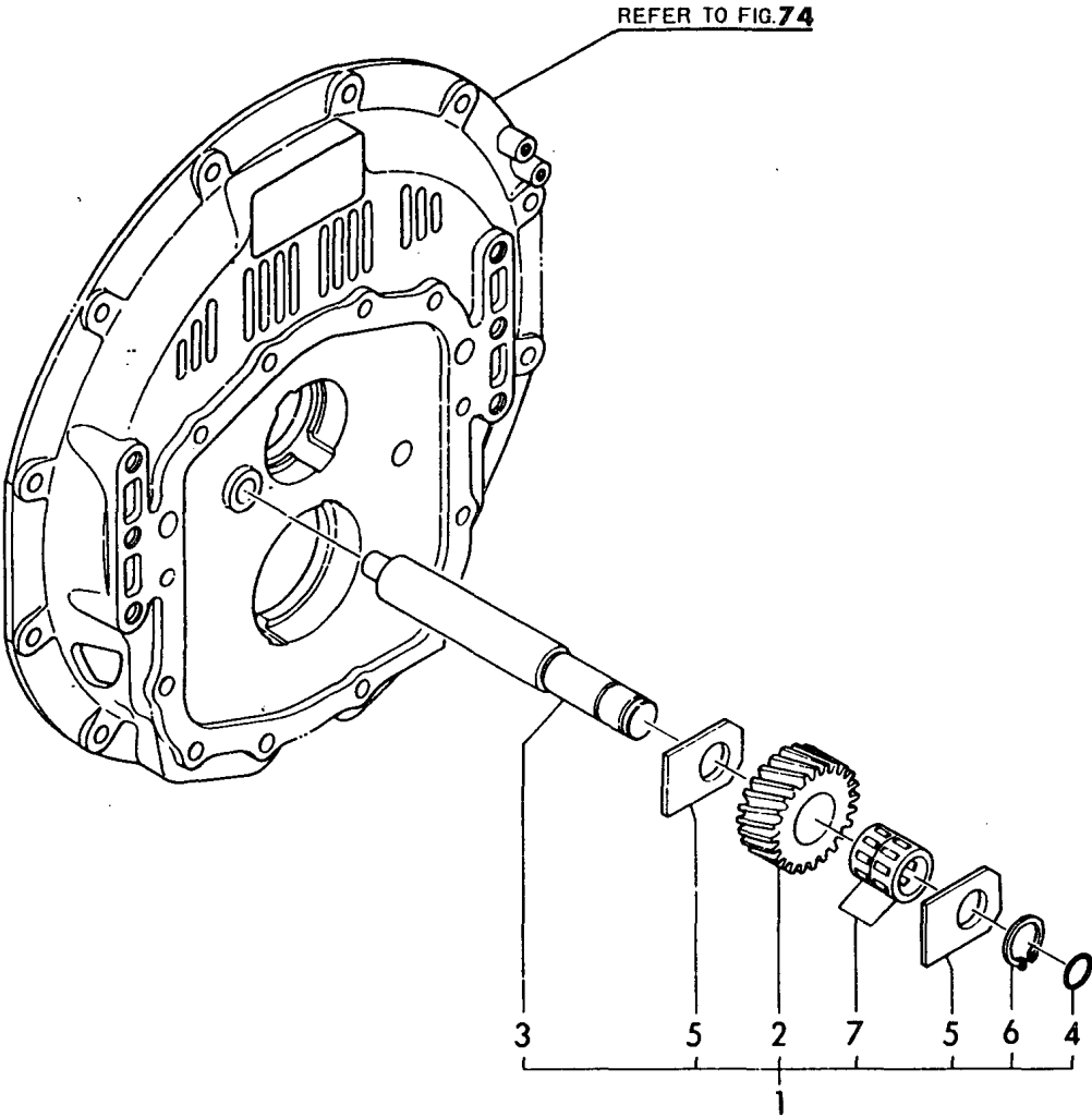
Fig.76 チュウカンジク COUNTER SHAFT
