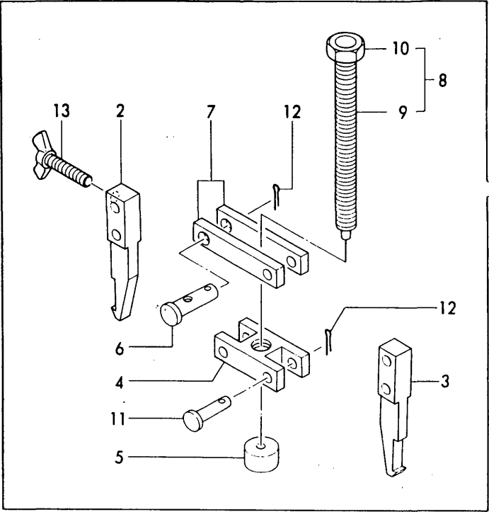
Fig.92 ブンカイコウグ(オプション) TOOL(OPTIONAL PART)
