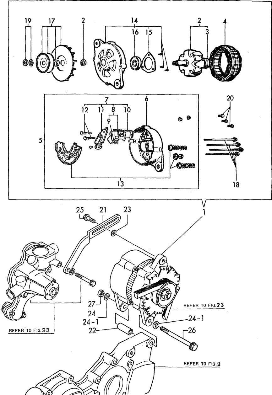
Fig.42 ジェネレータ GENERATOR
