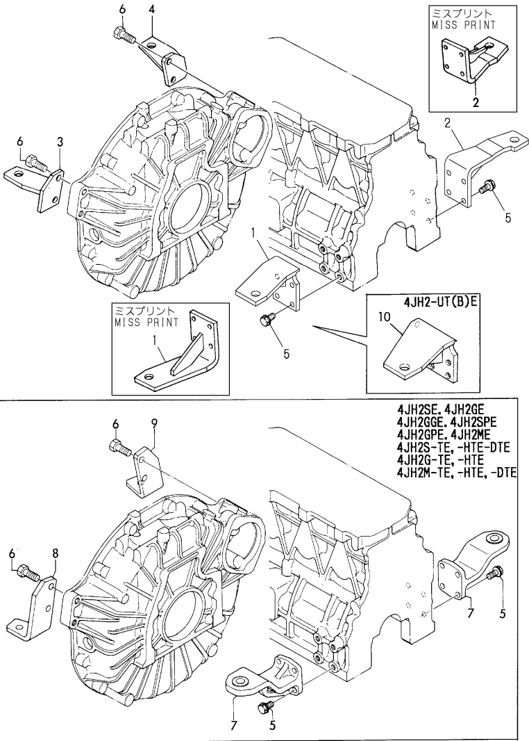
Fig.6 マウンティングフート MOUNTING FOOT
