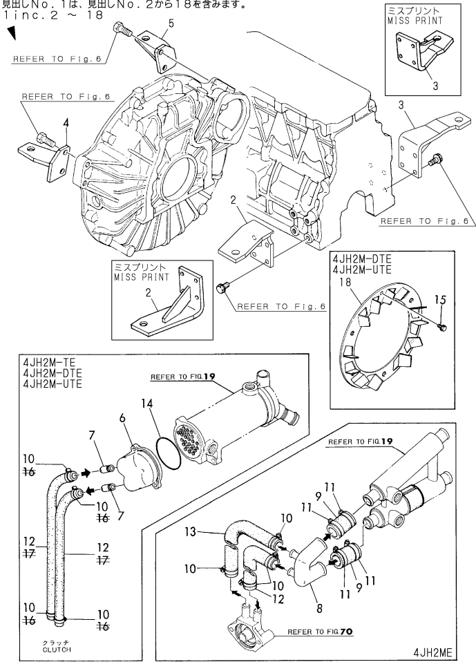
Fig.63 改装キット REEQUP MENT KIT
