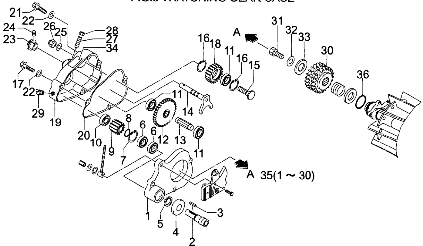
https://truckmanualshub.com/ サッチングギヤケース関係 FIG.5 THATCHING GEAR CASE
