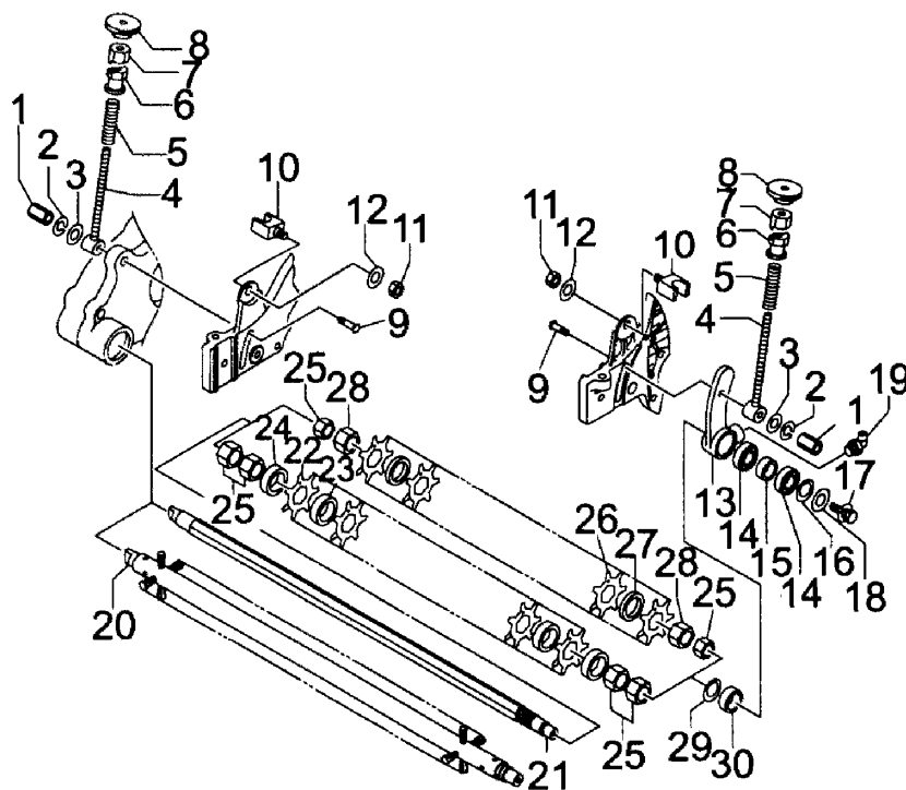
ゲルミニングカッター関係 FIG.9 GROOMING CUTTER
