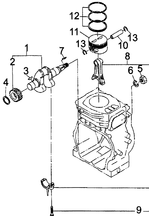
クランクシャフトとピストン FIG.2 CRANK SHAFT, PISTON
