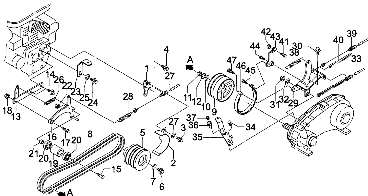
https://trucks.mitsubishi.com/ ディスカバリートラックのブレーキ関係 FIG.4 TENSION & BRAKE
