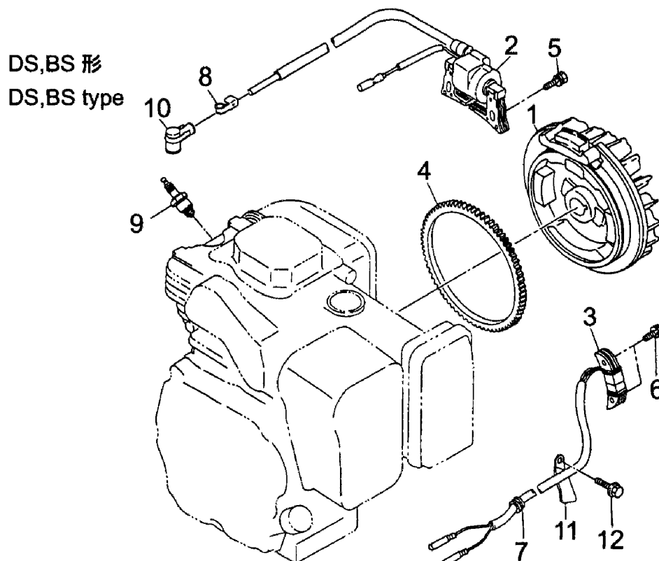
エレクトリック デバイス (セル付) FIG.8 ELECTRIC DEVICE (SEL STICK)
