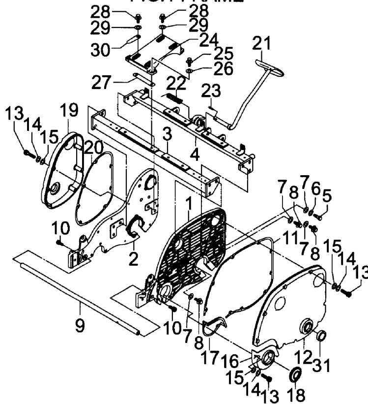
FIG.1 FRAME
