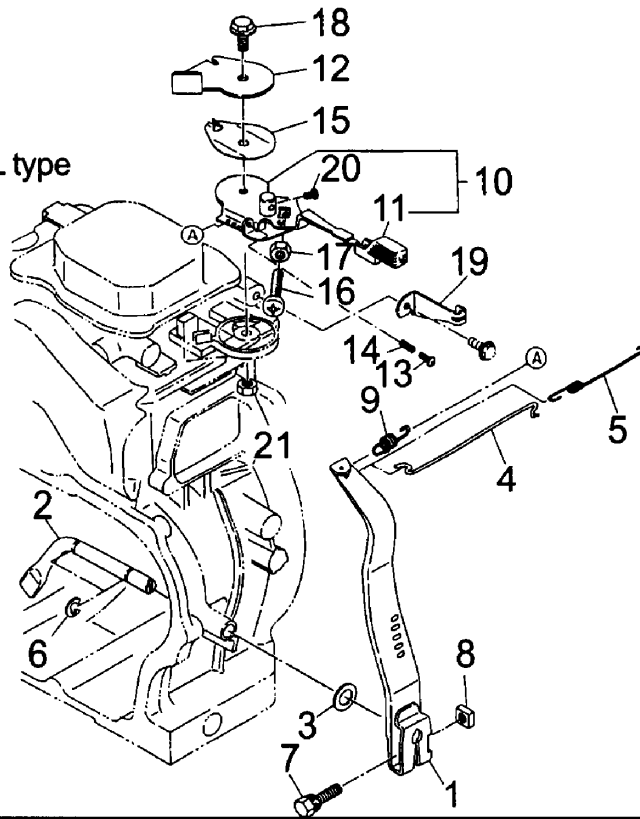
https://truckmanualshub.com/ ガバナ、オペレーション FIG.4 GOVERNOR, OPERATE
