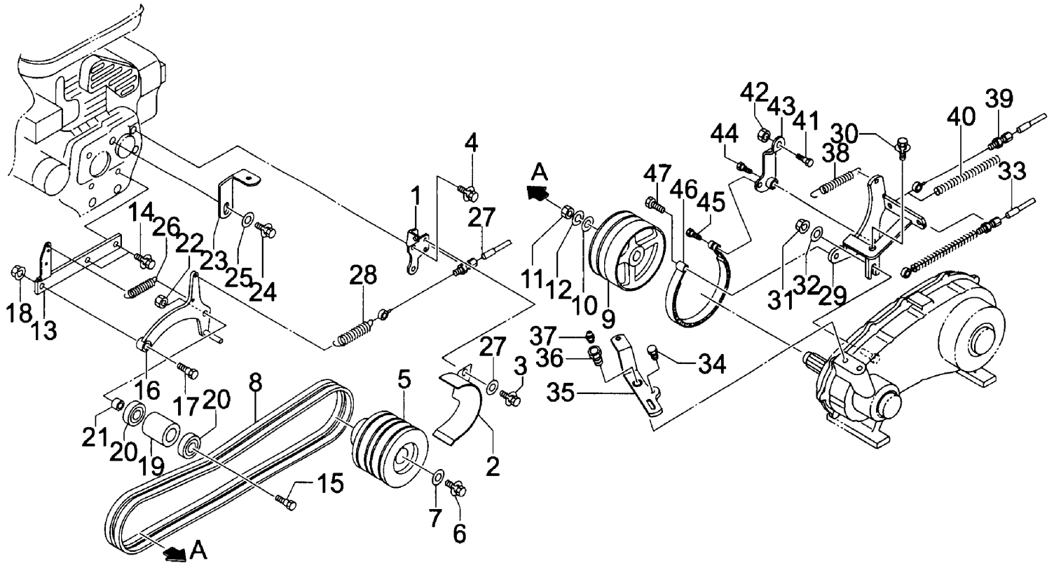
https://truckmanualshub.com/ テンション及びブレーキ関係 FIG.4 TENSION & BRAKE
