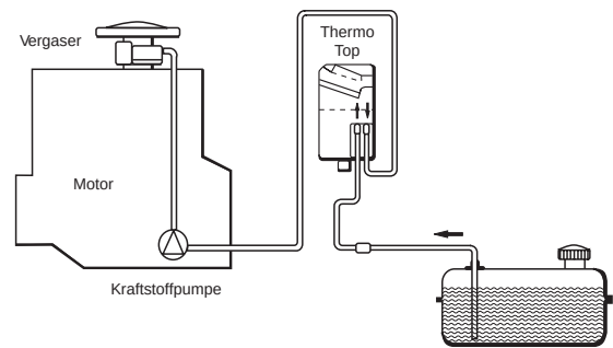
Abb. 805 Kraftstoffeinspeisung im Einleitungssystem (Vergasermotor ohne Rücklaufleitung) "Inline-Einbindung zwischen Kraftstofftank und -pumpe"
