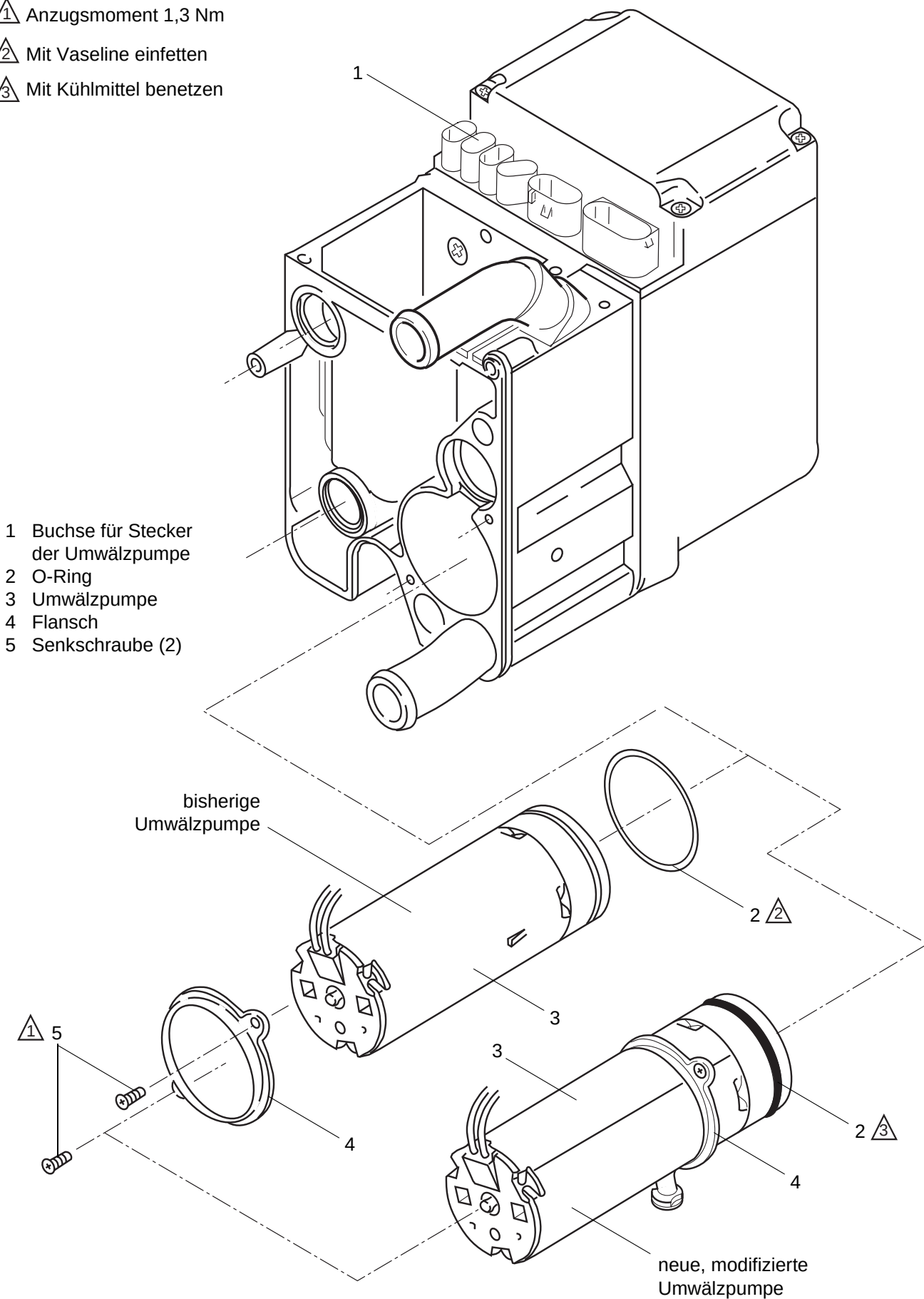
Abb. 902 Wechsel der Umwälzpumpe
