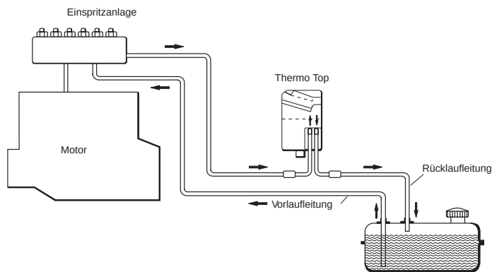
Abb. 804 Kraftstoffeinspeisung im Zweileitungssystem (Vergaser- bzw. Einspritzmotor mit Rücklaufleitung) "Inline-Einbindung im Rücklauf"
