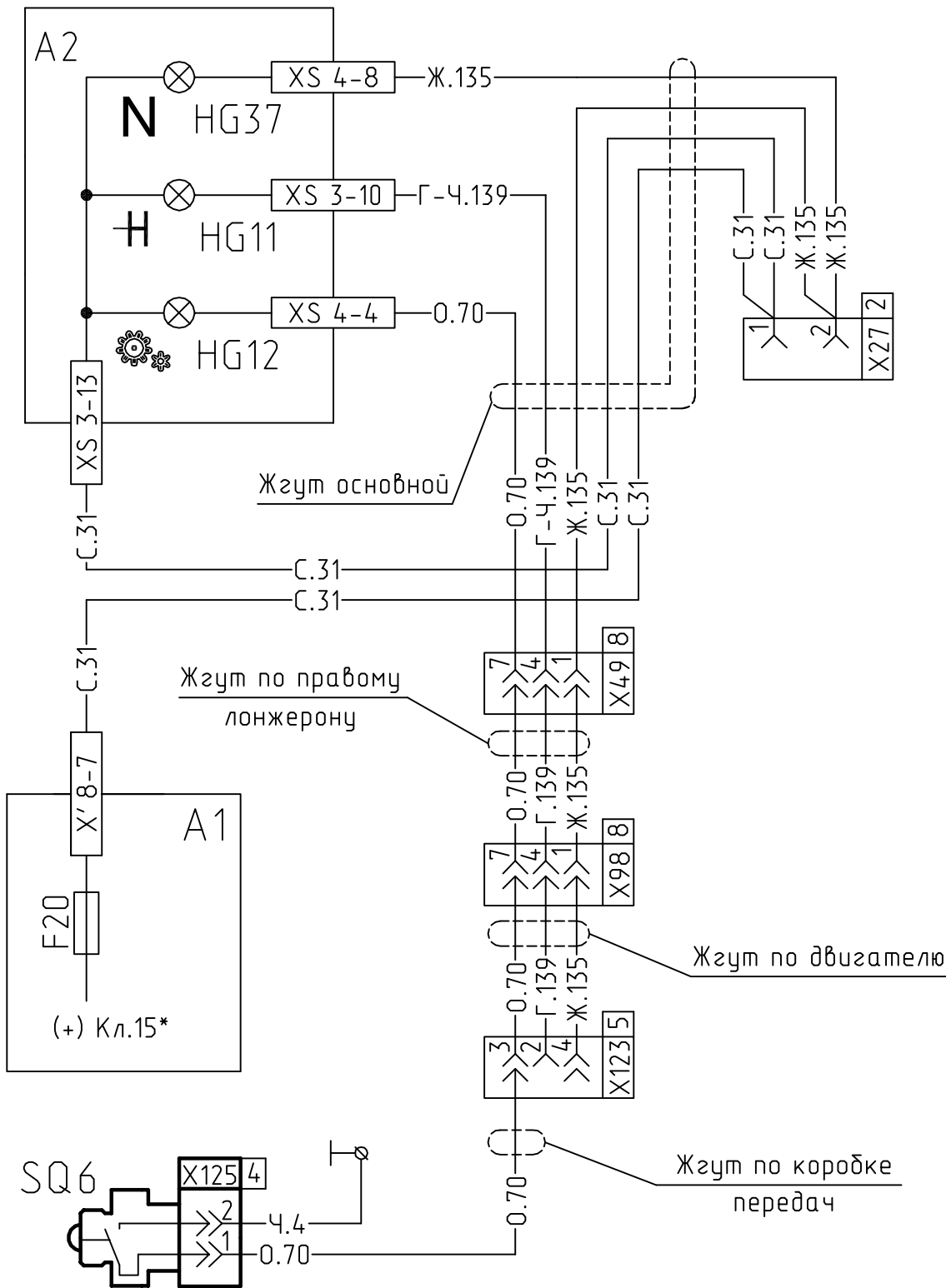
Схема включения контрольных ламп делителя КПП на коробках ЯМЗ-238М, МЗКТ 65151
