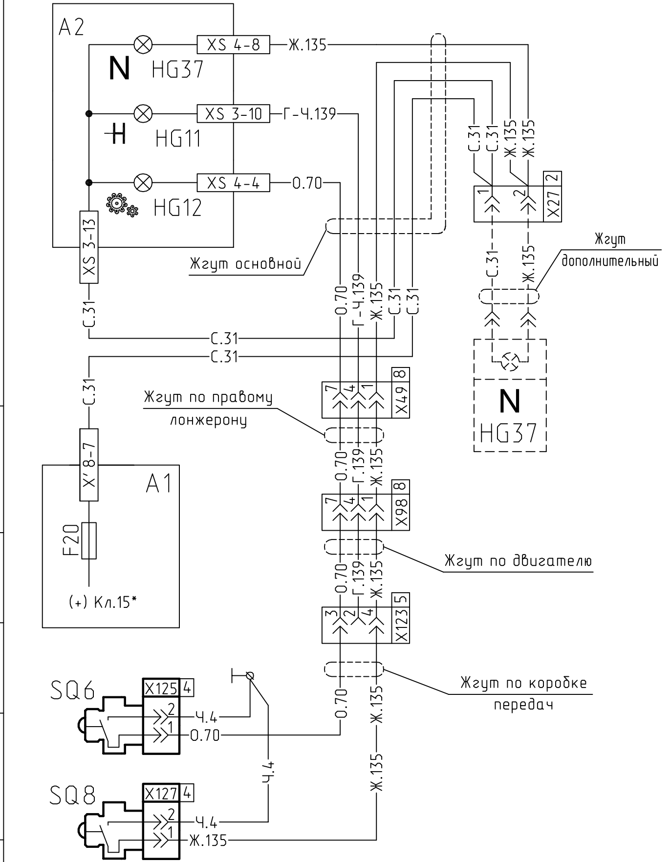
Схема включения контрольных ламп делителя и нейтрали КПП на коробках ЯМЗ-239,
