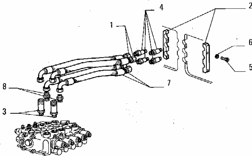
BACK-HOE RETROSCAVATORE
