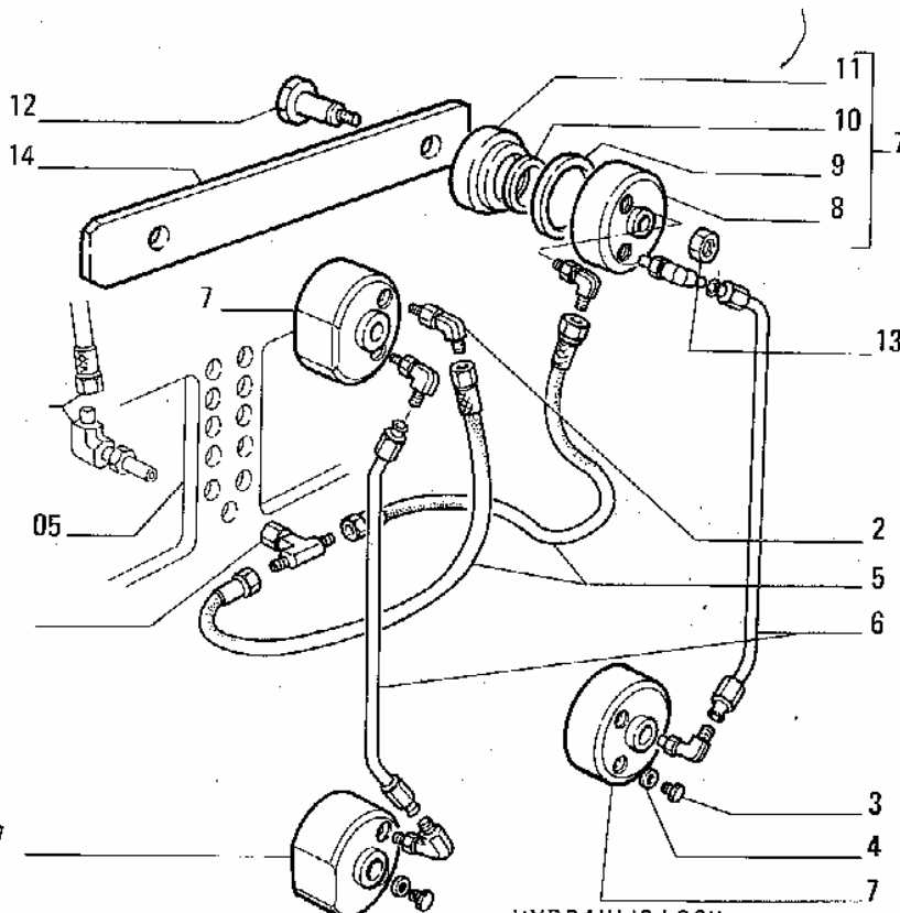
HYDRAULIC LOCK BLOCCAGGIO IDRAULICO
