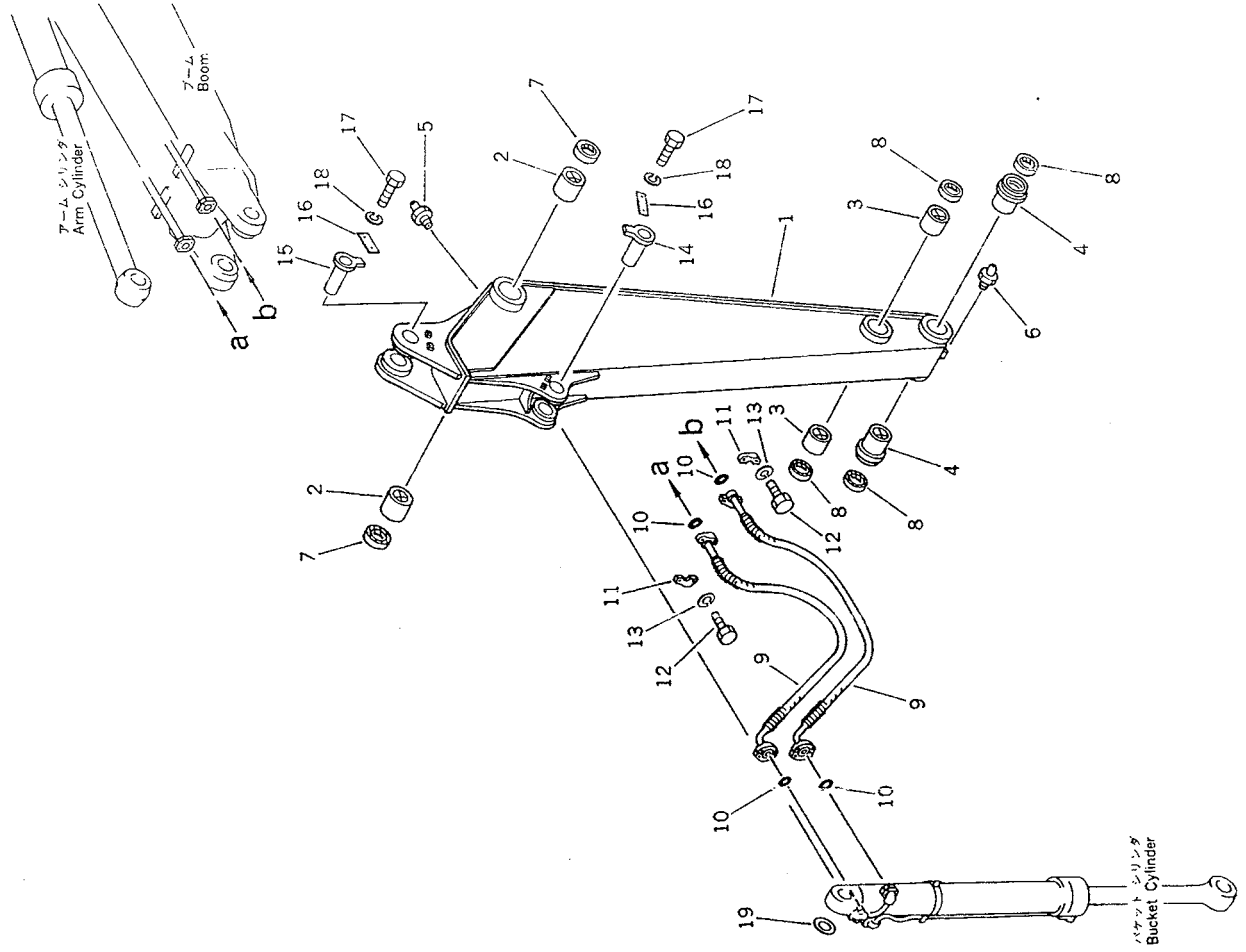
7-4 FIG. 7005 ARM 2250MM
