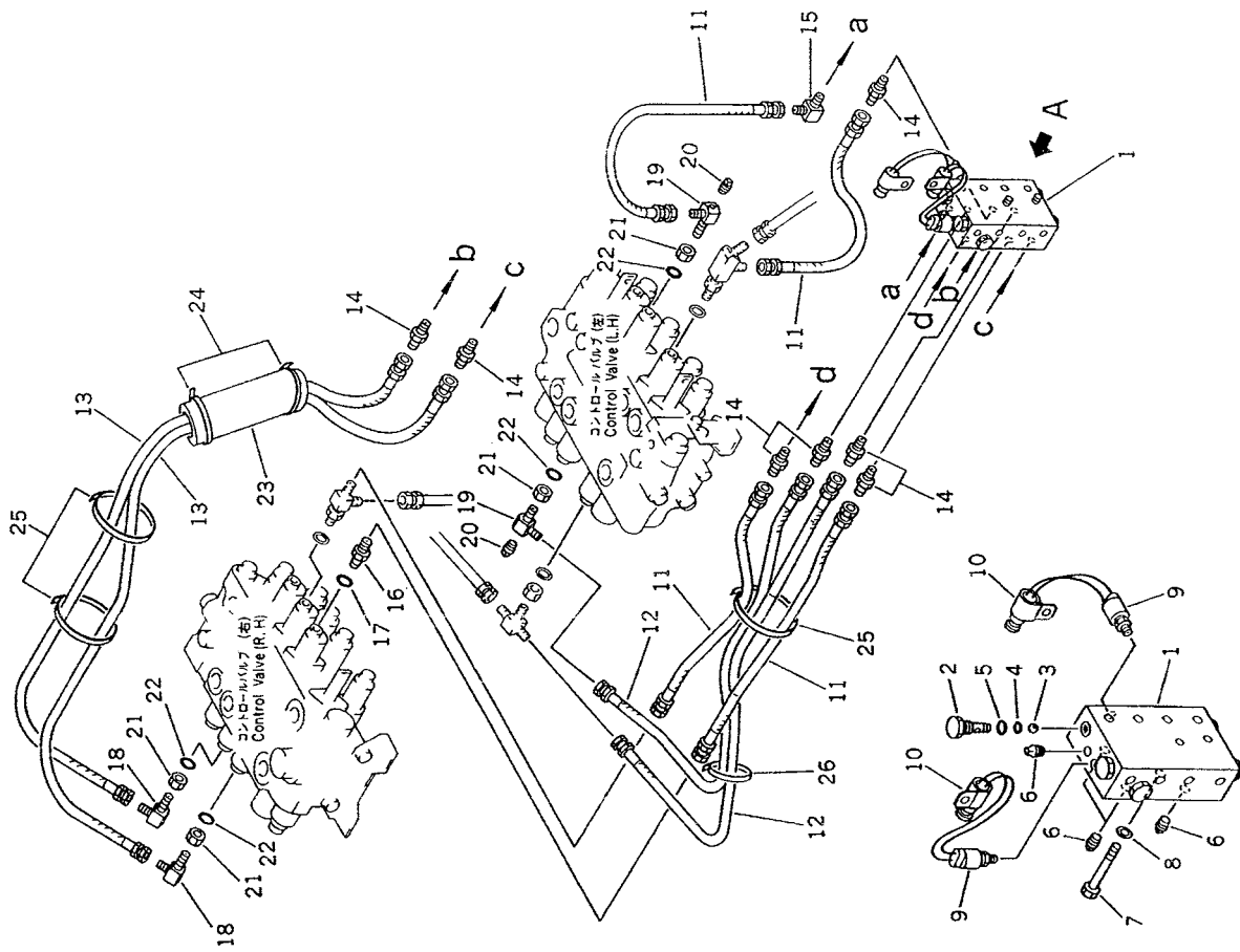
FIG. 4425 HYDRAULIC PIPING (VALVE TO SHUTTLE VALVE) バルブ → シャトル バルブ 旋回メカニカルブレーキ付 (WITH SWING MECHANICAL BRAKE)
