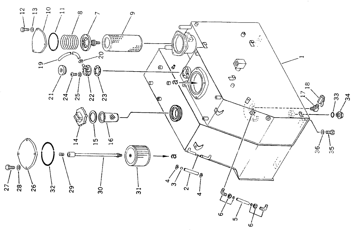
FIG. 6103 HYDRAULIC OIL および フュエル タンク フュエルセルフサプライボンプ取付に適用 (APPLICABLE FOR MOUNTING FUEL SELF SUPPLY PUMP)
