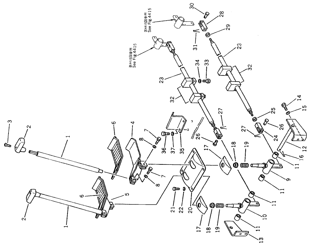
走行 コントロール レバー および ペダル FIG. 4413 TRAVEL CONTROL LEVER AND PEDAL
