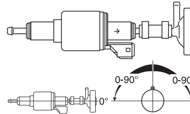
Bild 16: Dosierpumpe DP 30
