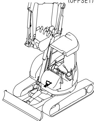
Fig. 31 操縦装置 (ブレード) CONTROL EQUIP. (BLADE)
