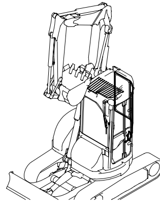
Fig. 47 キャビン (フロントガラス) CABIN (FRONT GLASS)
