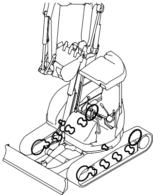
Fig. 26 クローラ CRAWLER
