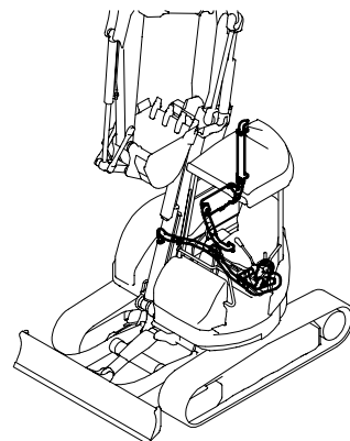
Fig. 8 アクセル ACCELERATOR
