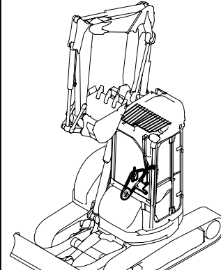
Fig. 22 コンデンサ&コンプレッサ (クーラ仕様) CONDENSER & COMPRESSOR (COOLER SPEC.)
