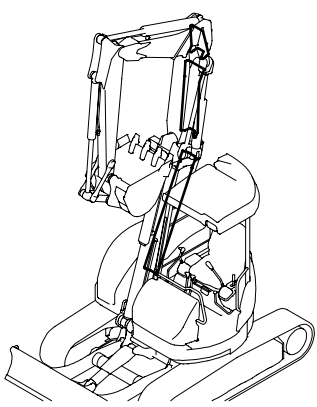
Fig. 36 カバー (ブーム) COVER (BOOM)
