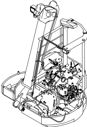
Fig. 15 電装品 (ワイヤリング:クレーン仕様) ELECTRIC PART (WIRING:CRANE)
