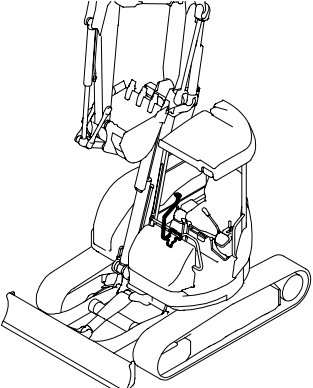
Fig. 32 操縦装置 (ローハイペダル) CONTROL EQUIP. (LOW-HIGH PEDAL)
