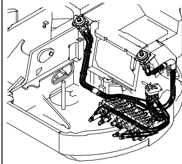
Fig. 83 コントロール配管 (2ウェイマルチチェンジ : クレーン) CONTROL PIPING (2-WAY MULTI CHANGE : CRANE)
