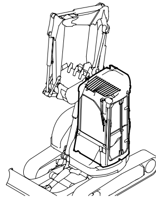
Fig. 46 キャビン (リアガラス) CABIN (REAR GLASS)
