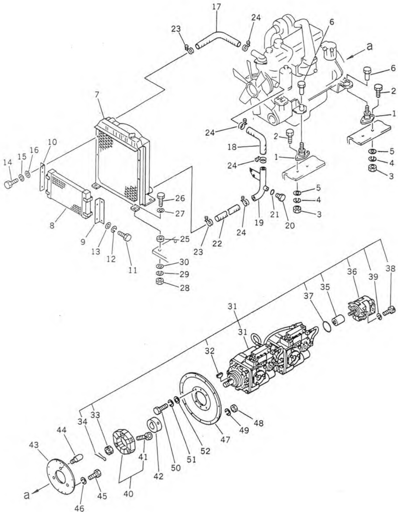
エンジン 関連 部品 FIG. 101 ENGINE RELATED PARTS
