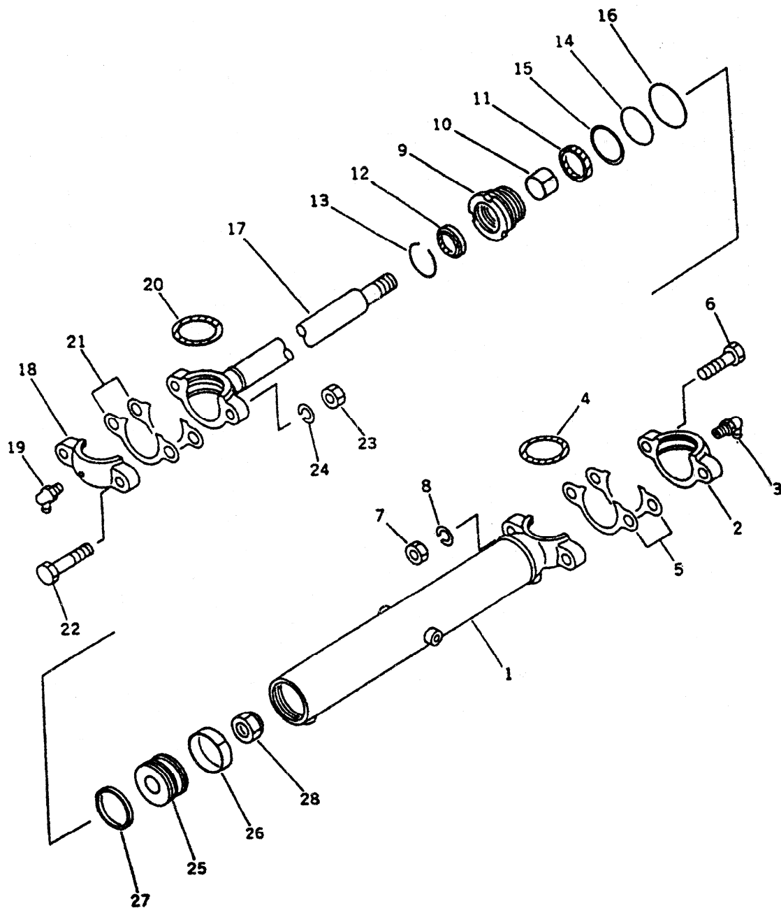
FIG. 6301 牵引架倾斜油缸 DRAWBAR SHIFT CYLINDER
