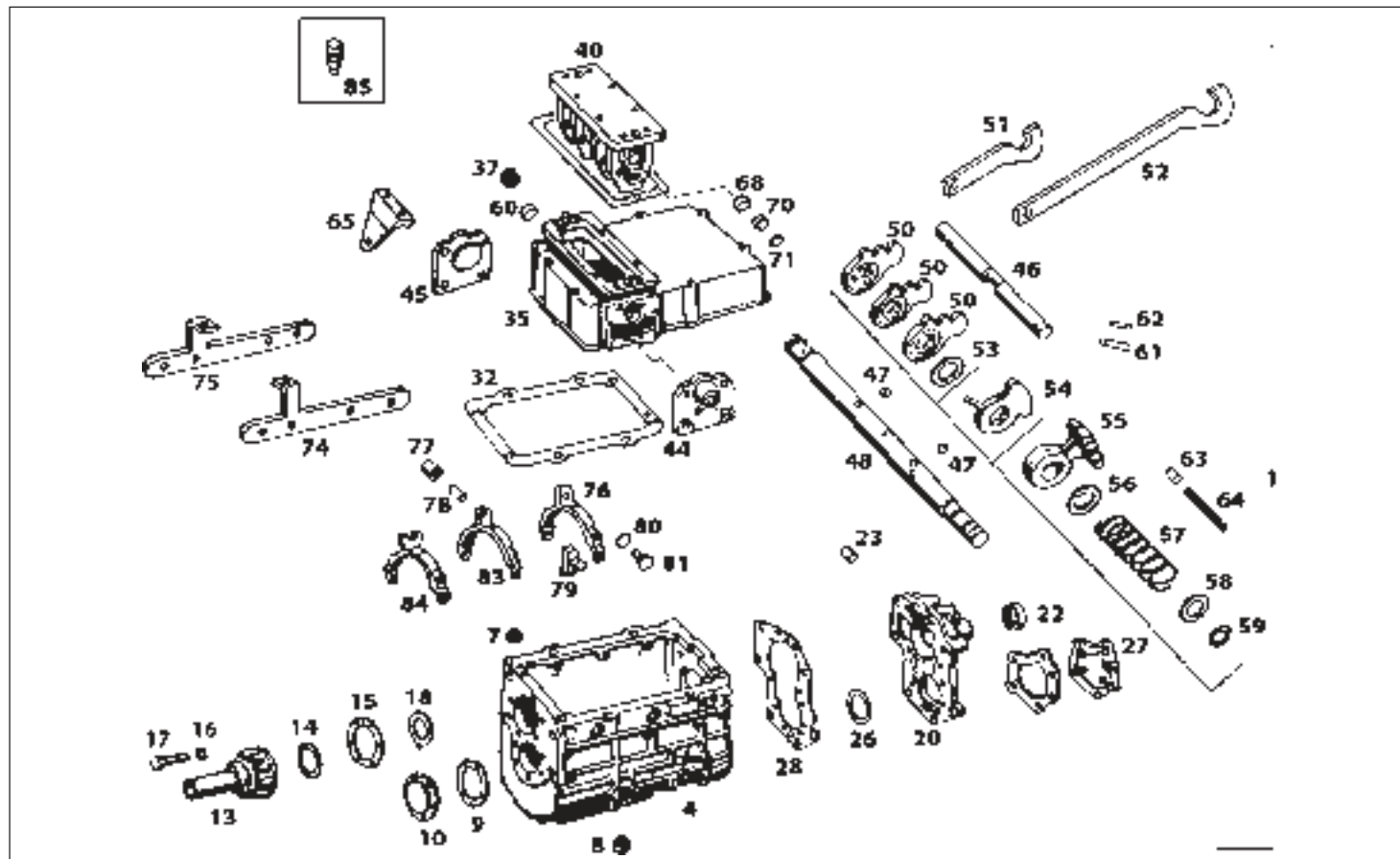
GEAR BOX (GBS 50)
