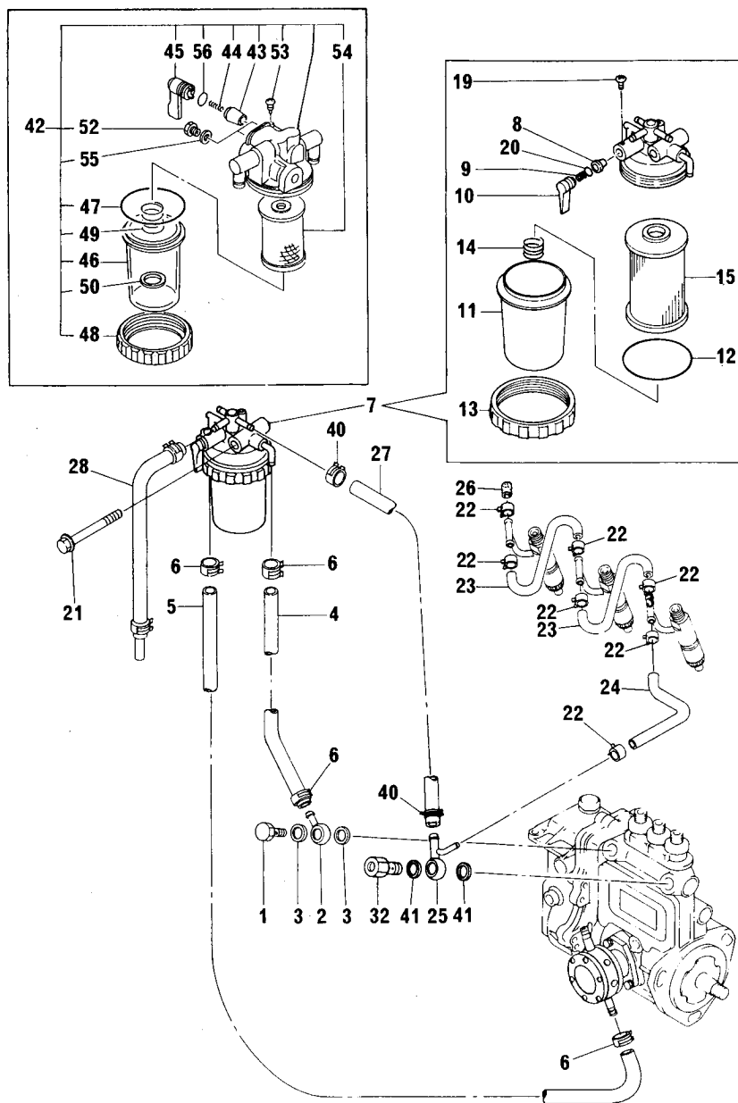
FIG. 0410 IMPIANTO COMBUSTIBILE FUEL LINE
