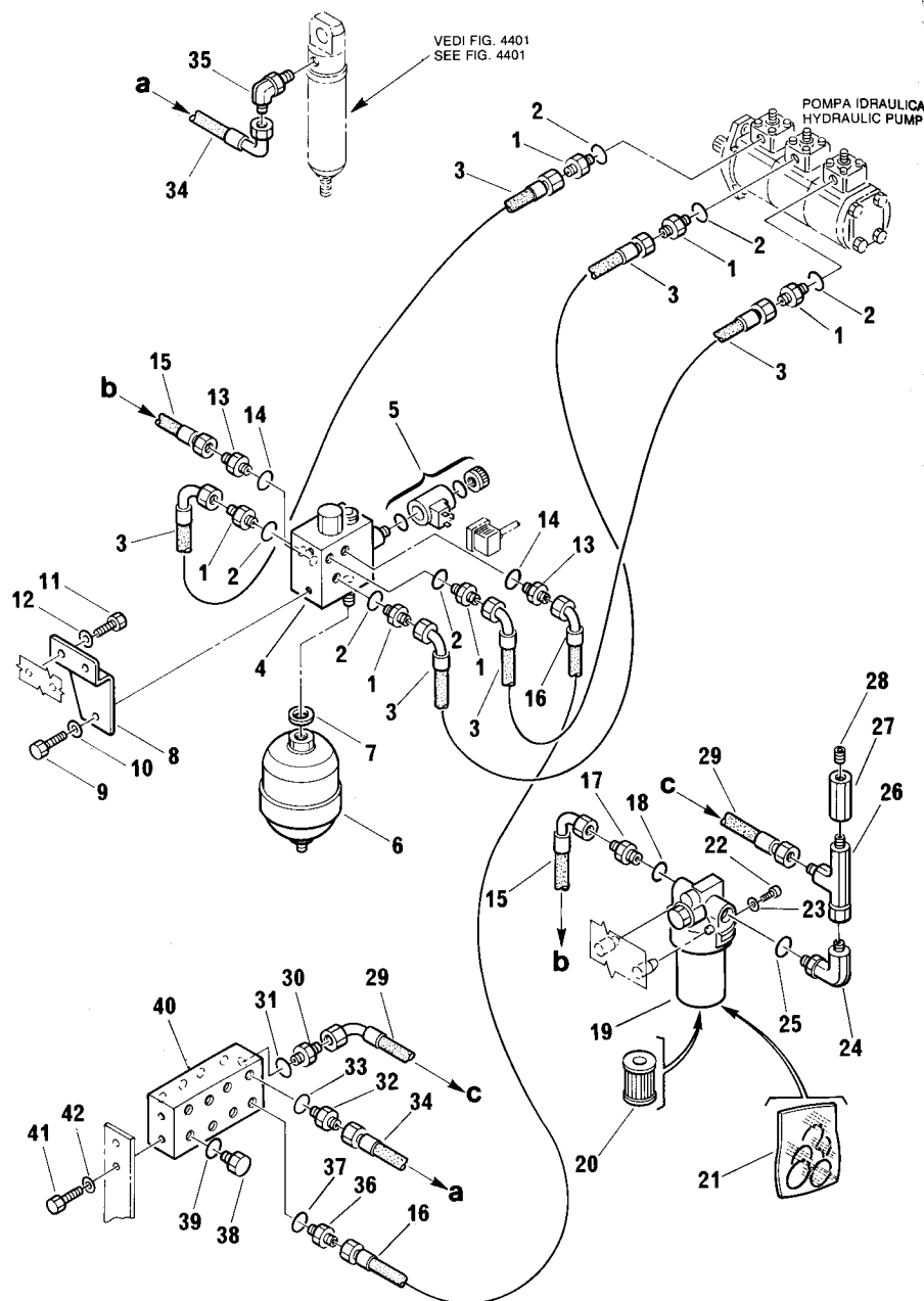
FIG. 6531 IMPIANTO IDRAULICO MANDATA-SCARICO SERVOCOMANDI HYDRAULIC PIPING (SERVOCONTROL LINE)
