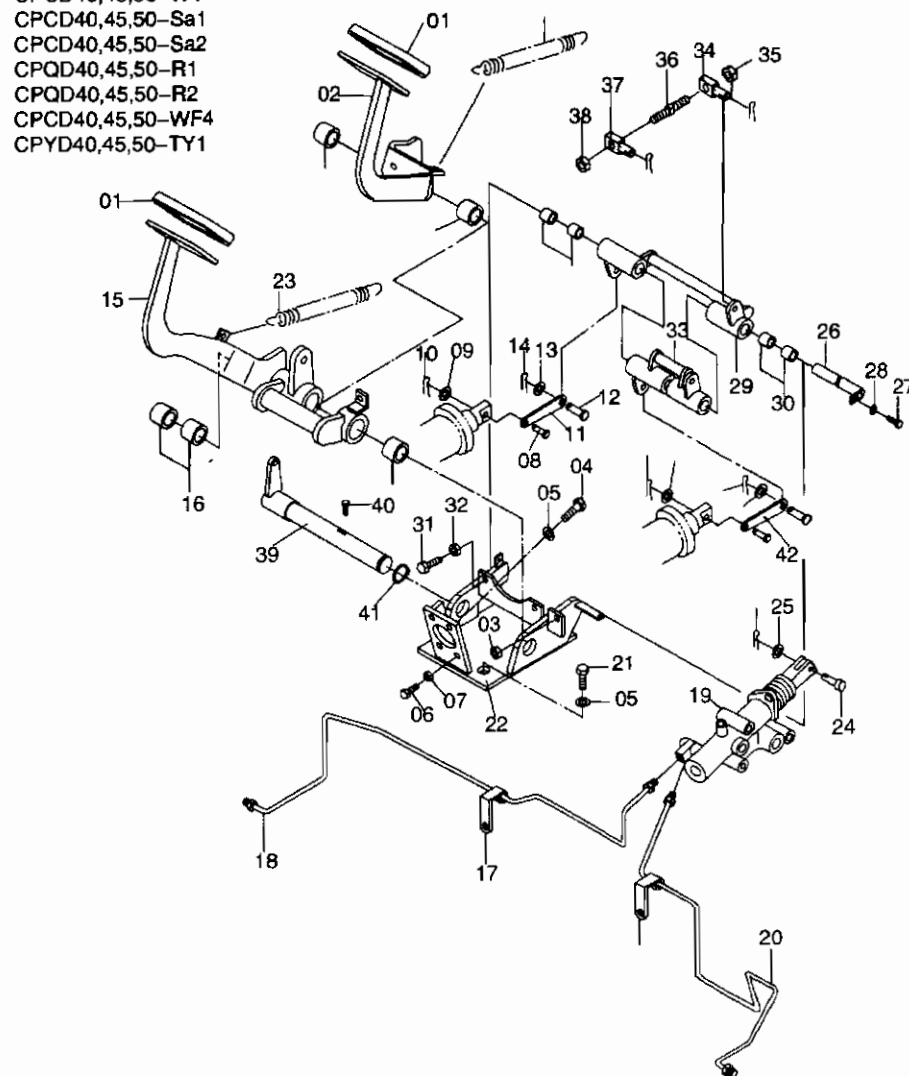
行车制动与微动操纵/BRAKE&amp;INCHING CONTROL
