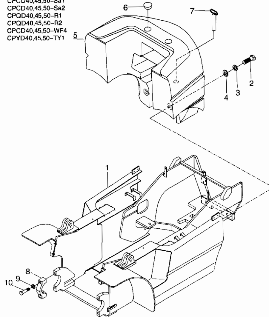
车架与平衡重/FRAME&amp;COUNTER WEIGHT
