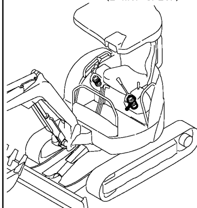
Fig. 82 ロータリバルブ (4ウェイ仕様) ROTARY VALVE (4-WAY SPEC.)
