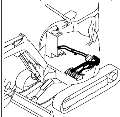
Fig. 84 油圧配管 (タンク〜ポンプ〜バルブ) HYD. OIL PIPING (TANK - PUMP - VALVE)
