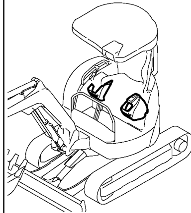
Fig. 48 シート & シートマウント SEAT & SEAT MOUNT (CABIN SPEC.)
