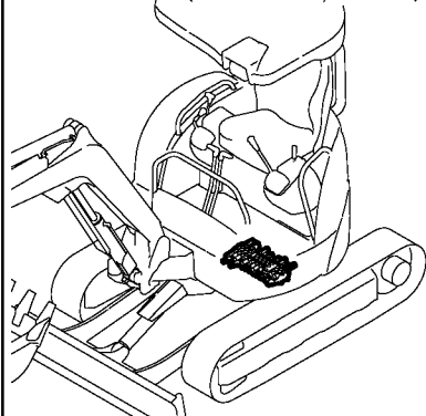
Fig. 79 コントロールバルブ (旋回 & プレート) CONTROL VALVE (TURNING BLADE)
