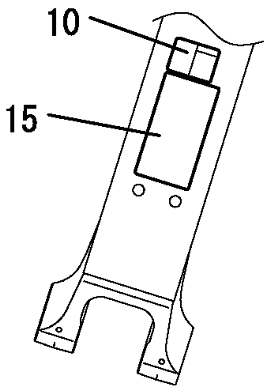
Ⓑ から見る VIEWED FROM Ⓑ
