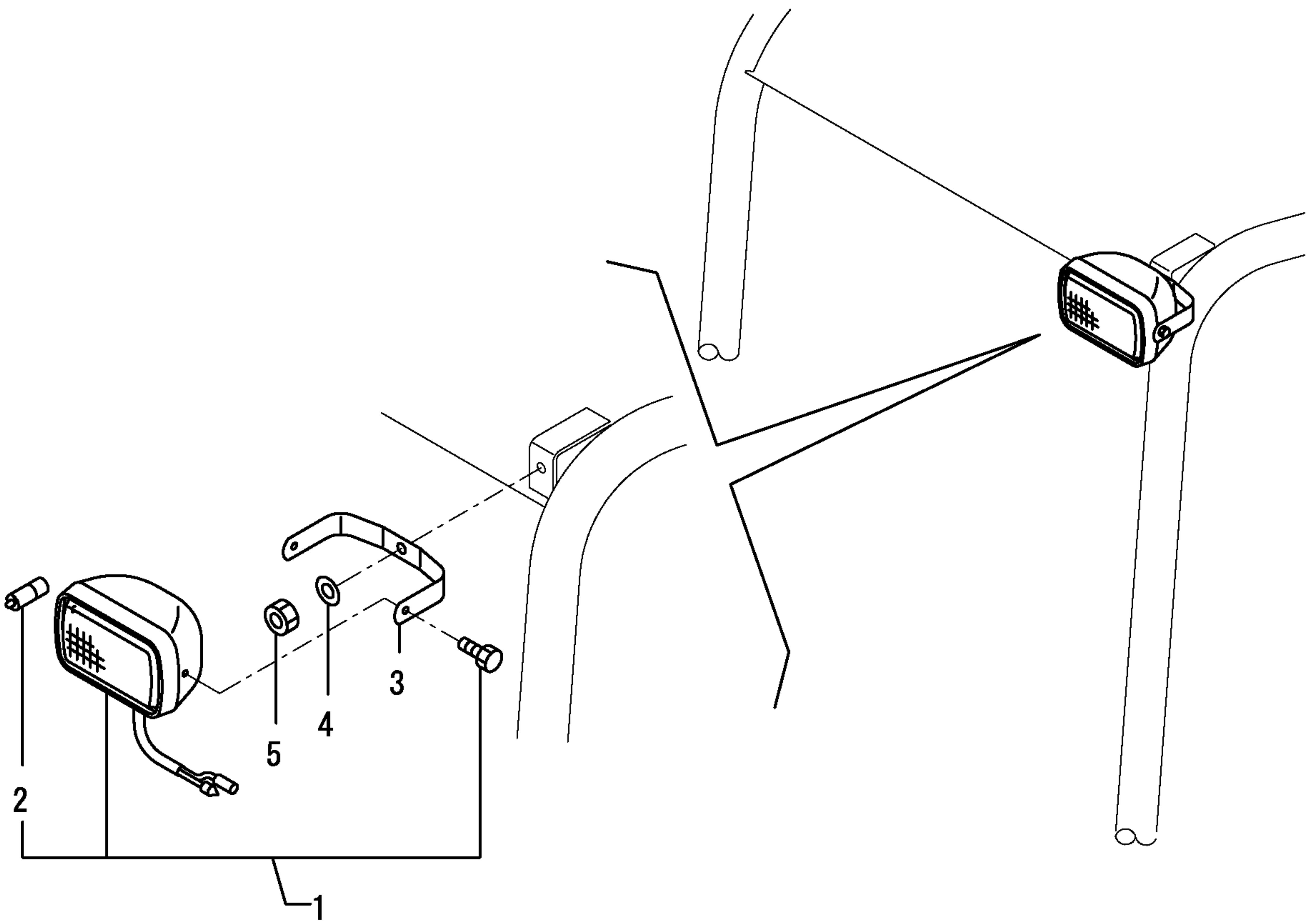
ROPSキャノピ仕様 ROPS CANOPY SPEC.
