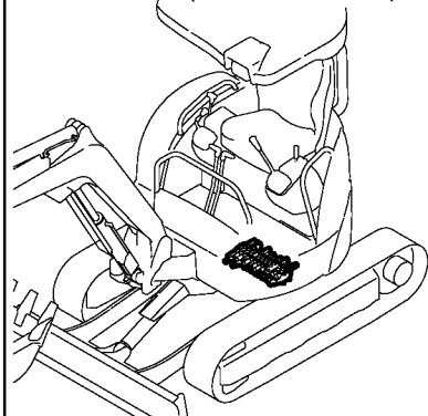
Fig. 75 コントロールバルブ (ブーム2 & 走行:右) CONTROL VALVE (BOOM 2 & TRAVEL:RIGHT)
