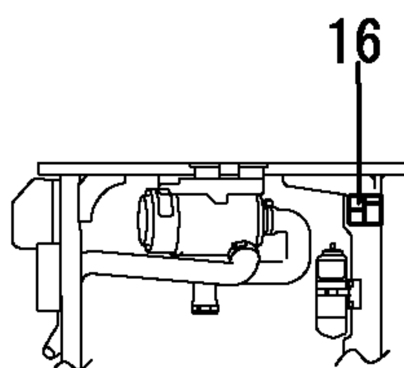
ボンネット内部詳細 DETAILS OF BONNET INSIDE
