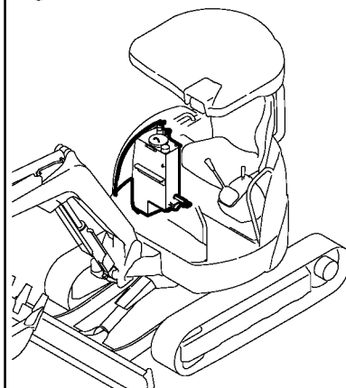
Fig. 84 油圧配管 (タンク〜ポンプ〜バルブ) HYD. OIL PIPING (TANK - PUMP - VALVE)
