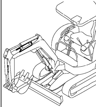
Fig. 44 カバー (ブーム) COVER (BOOM)
