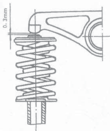
рис.7-8 холодный зев воздухзаборника 0.3mm рис.7-9 холодный зев исхода 0.4mm
