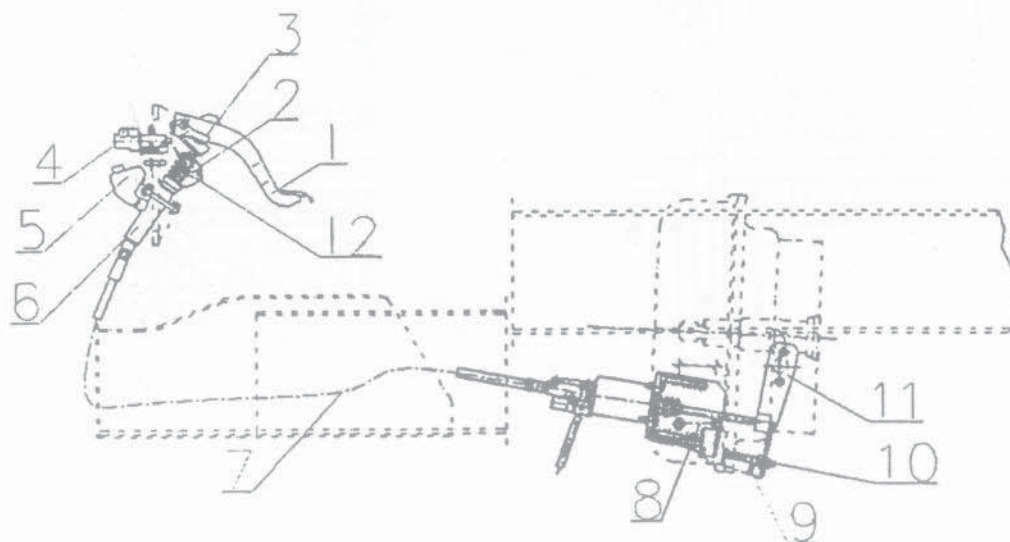
Рис.1 схема установки управления сцеплением
