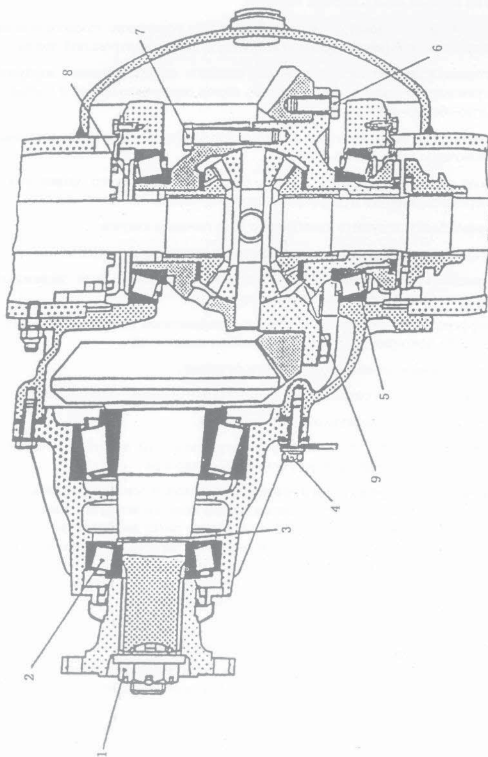
Рис. 6—8 конструктивная диаграмма заднего ося 1. гайка фланца 2. катучий конический подшипник 3. регулирующая шайба для подшипникового предварительного натяжения 4, 6, 7. болт 5. подшипник дифференциала 8. регулирующая гайка 9. регулирующая шайба для зазора между зубчатыми колесами дифференциала
