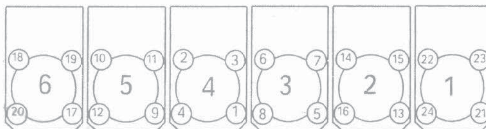
Рис. 6 схема закручивающего порядка вторичной гайки главного болта головки цилиндра.
