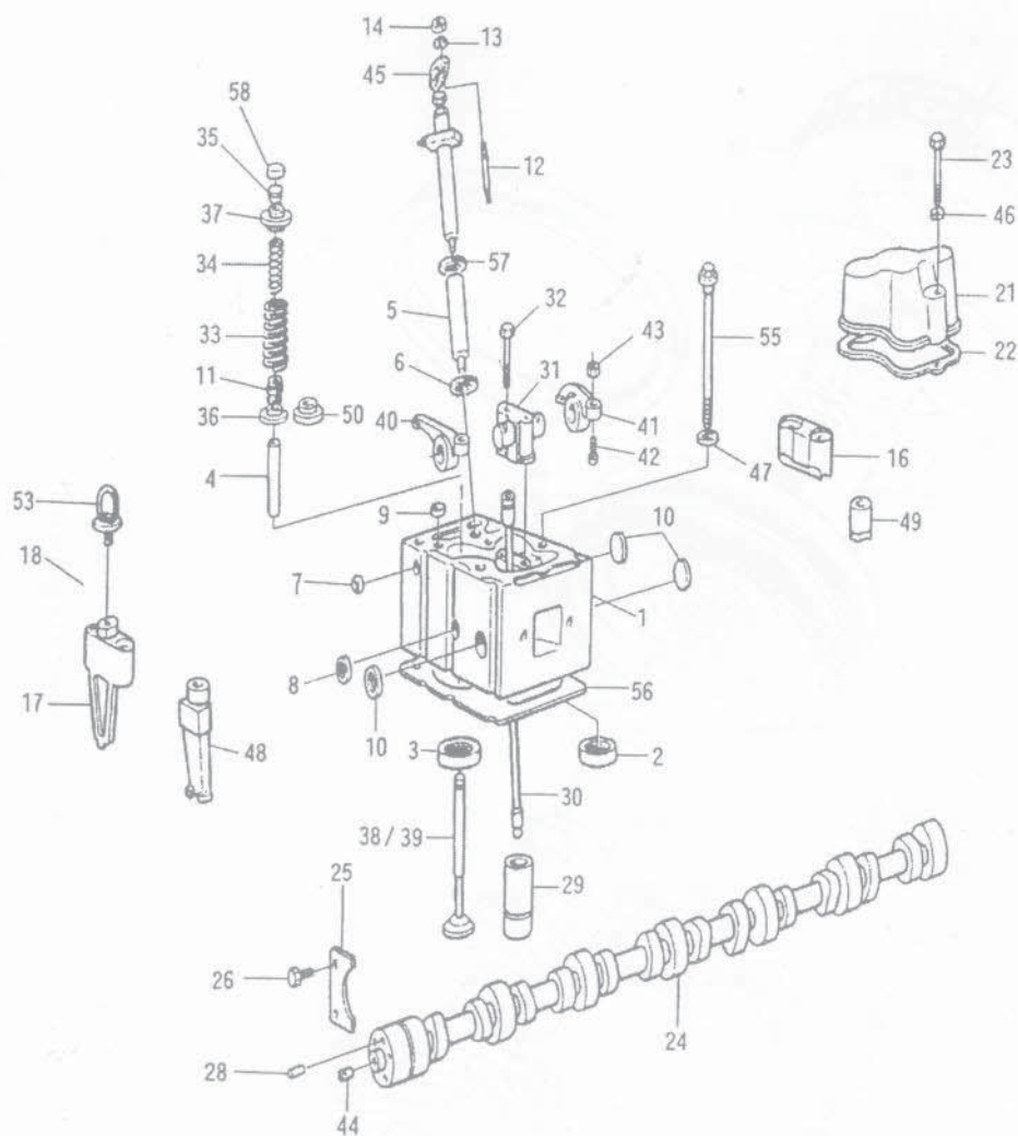
Рис. 7—7 крышка цилиндров и система воздухоораспределения
