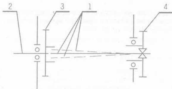
1. шпиндель 2. Вводный валик 3. Зубчатка вводного валика, 4. Приводная зубчатка побояной коробки
