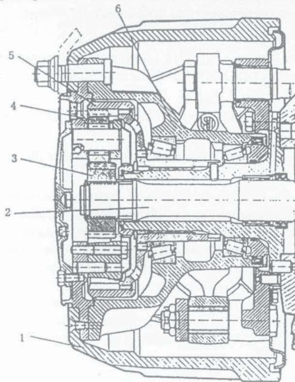
Рис. 6-2 Конструкция ободного редуктора приводной оси
