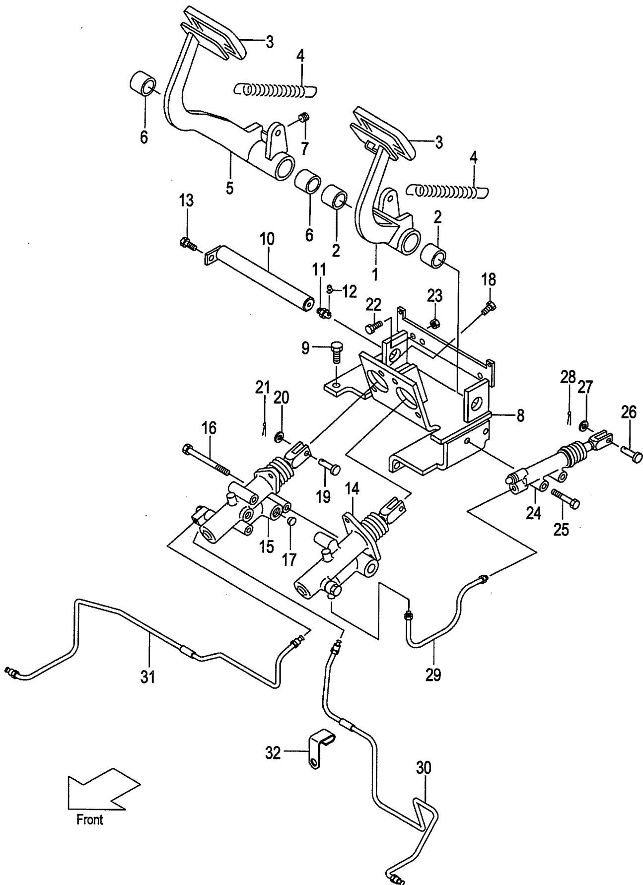
FIG.45 CLUTCH & BRAKE PEDAL (CLUTCH) (F6045410) クラッチ&ブレーキペダル
