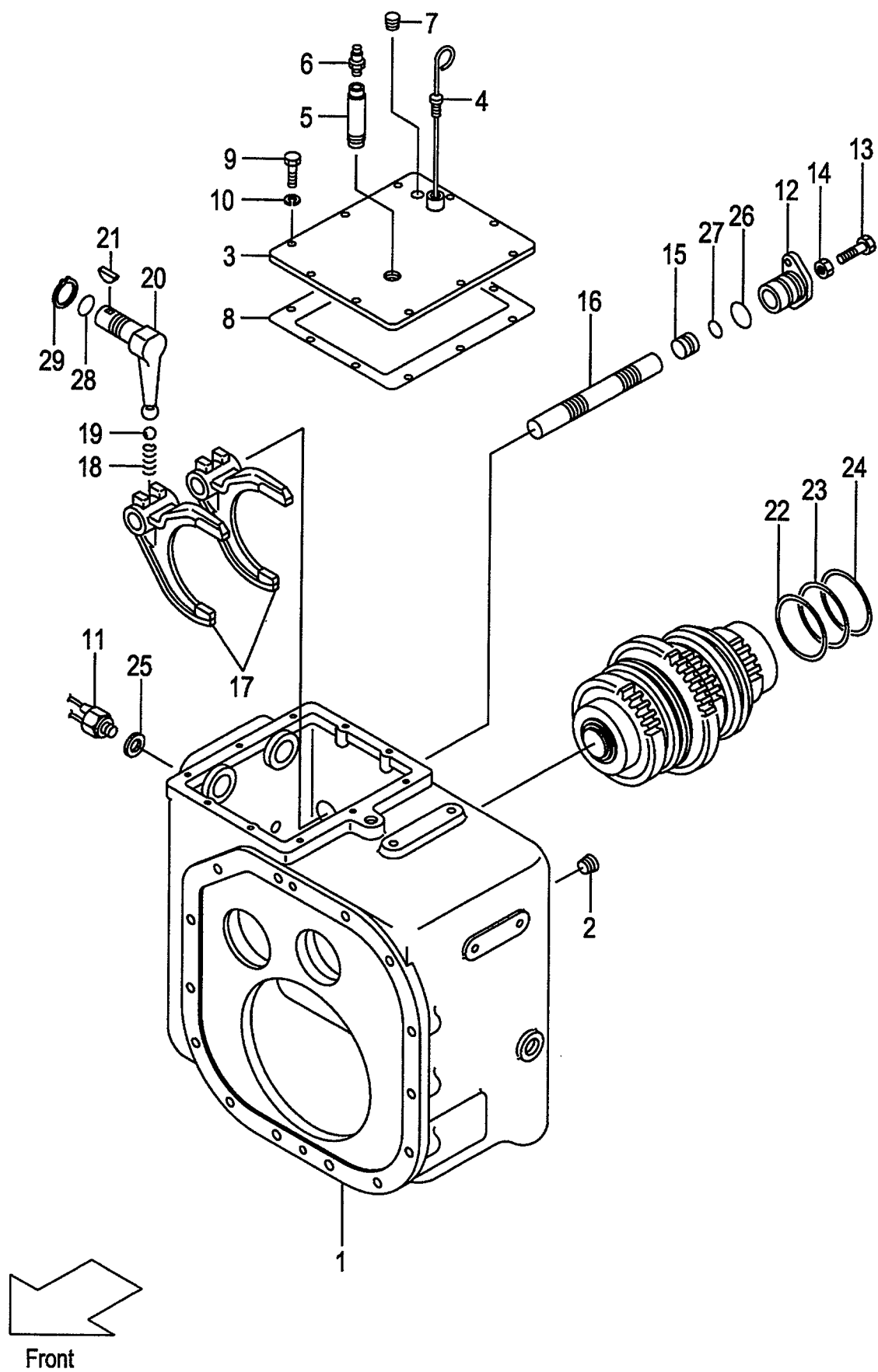
FIG.24 DRIVE UNIT (2/3)(CLUTCH) (F6042540) ドライブユニット
