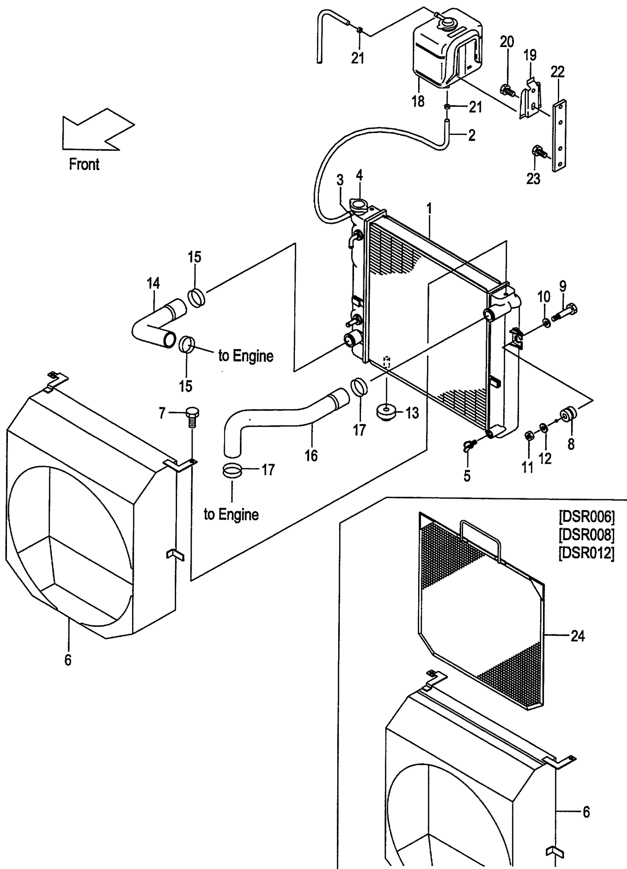
FIG.5 COOLING UNIT (F6042110) クーリングユニット
