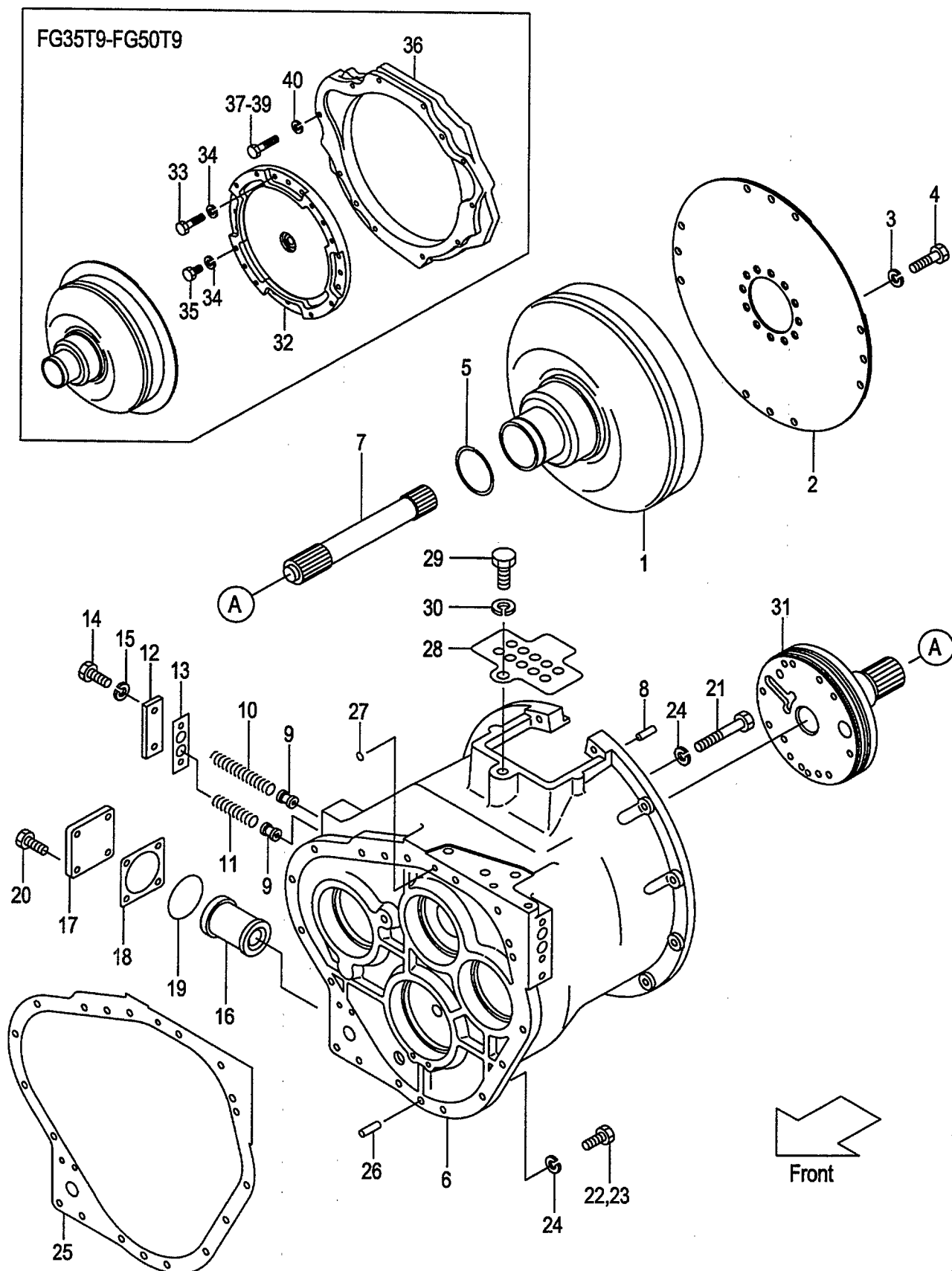
FIG.26 DRIVE UNIT (1/2)(TOR-CON) (F6042560) ドライブユニット
