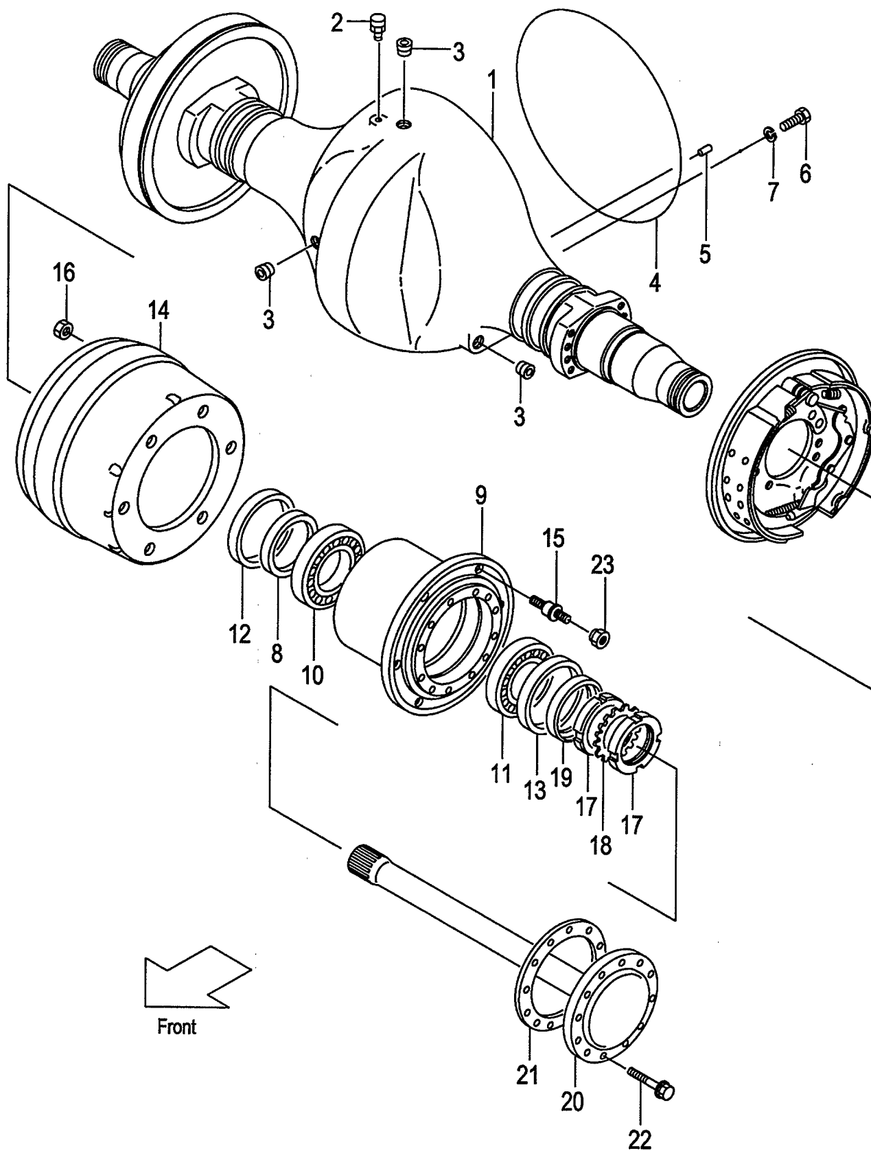
FIG.32 DRIVE AXLE (F6043020) ドライブアクスル
