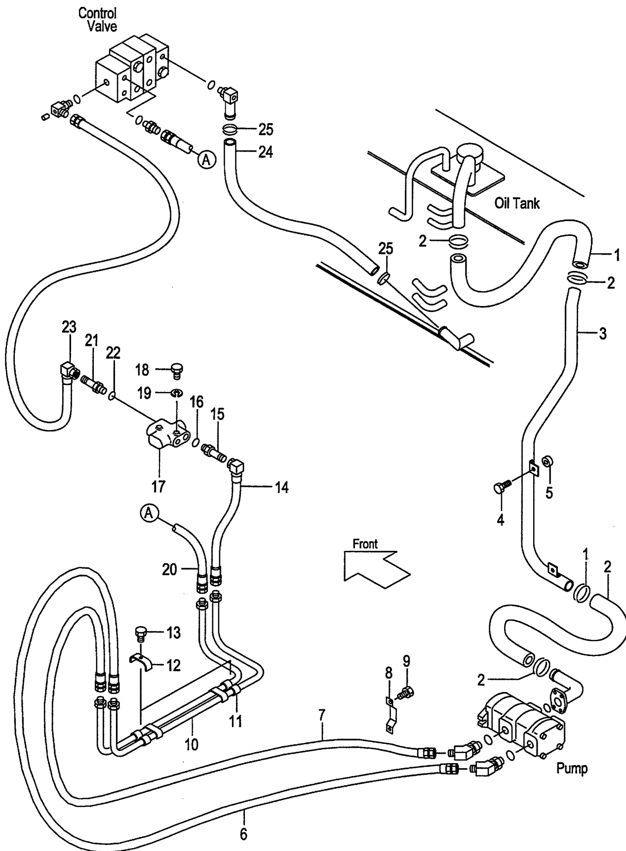
FIG.77 HYDRAULIC LINE(MAIN)(1/4) (F6047610) ハイドロリックライン
