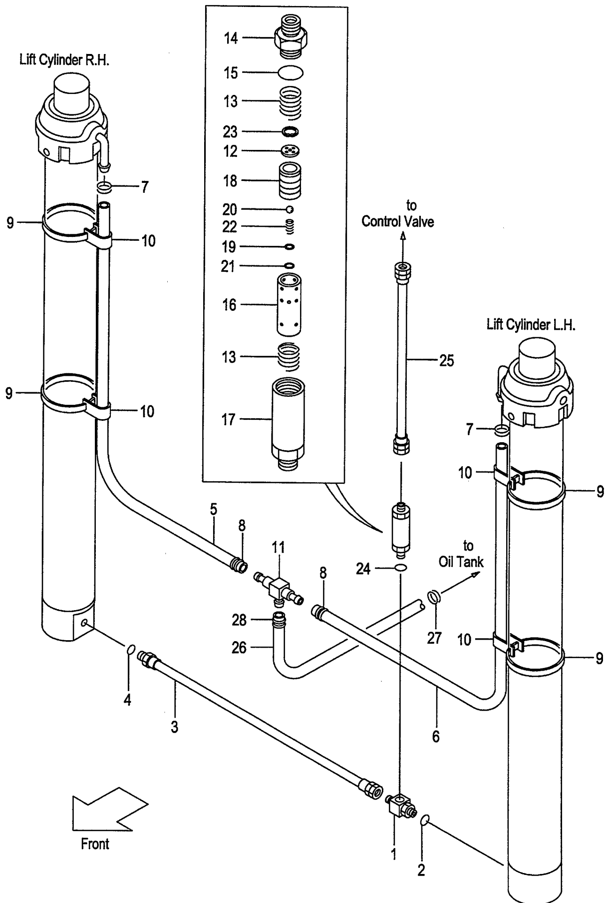
FIG.95 MAST PIPING [VM43A] (M6048420) マストパイピング
