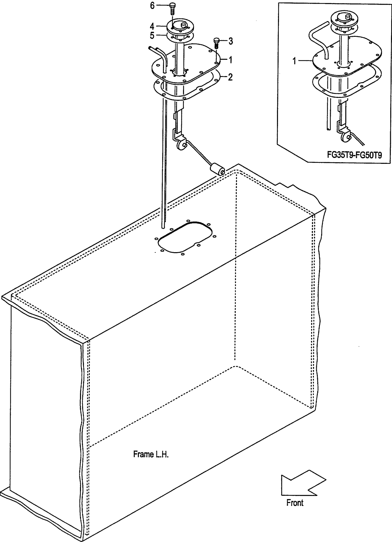
FIG.53 FUEL TANK (F6046130) フューエルタンク
