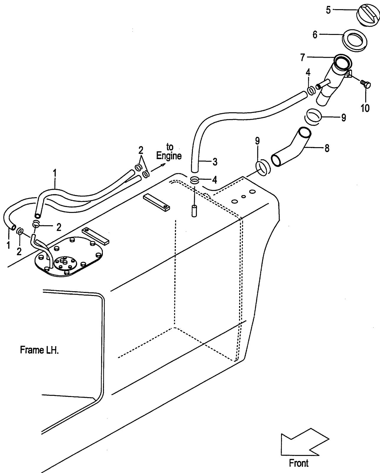
FIG.7 FUEL LINE (F6042210) フューエルライン
