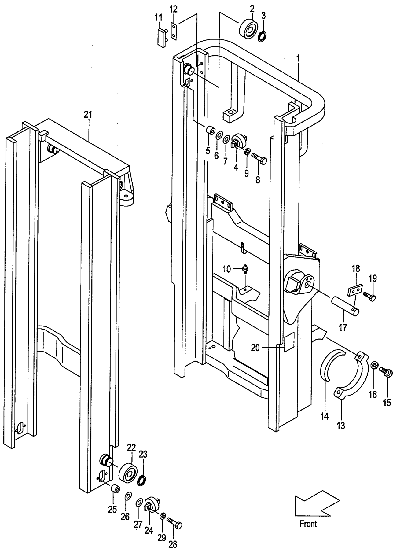
FIG.105 MAST [VM43H] (M6048340) マスト
