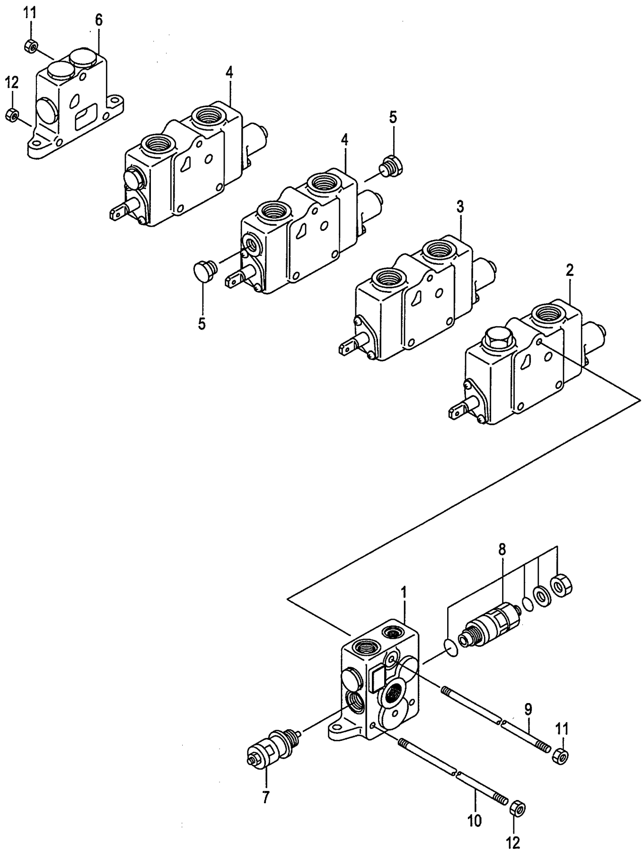
FIG.64 CONTROL VALVE [4SV] (F6047330) コントロールバルブ
