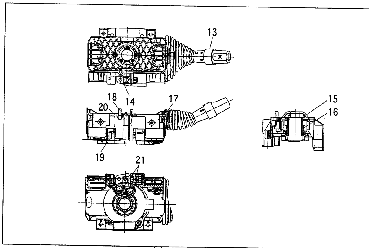
FIG.15 ELECTRIC PARTS (STEERING SHAFT COVER)(CLUTCH) (F6042450) エレクトリックパーツ
