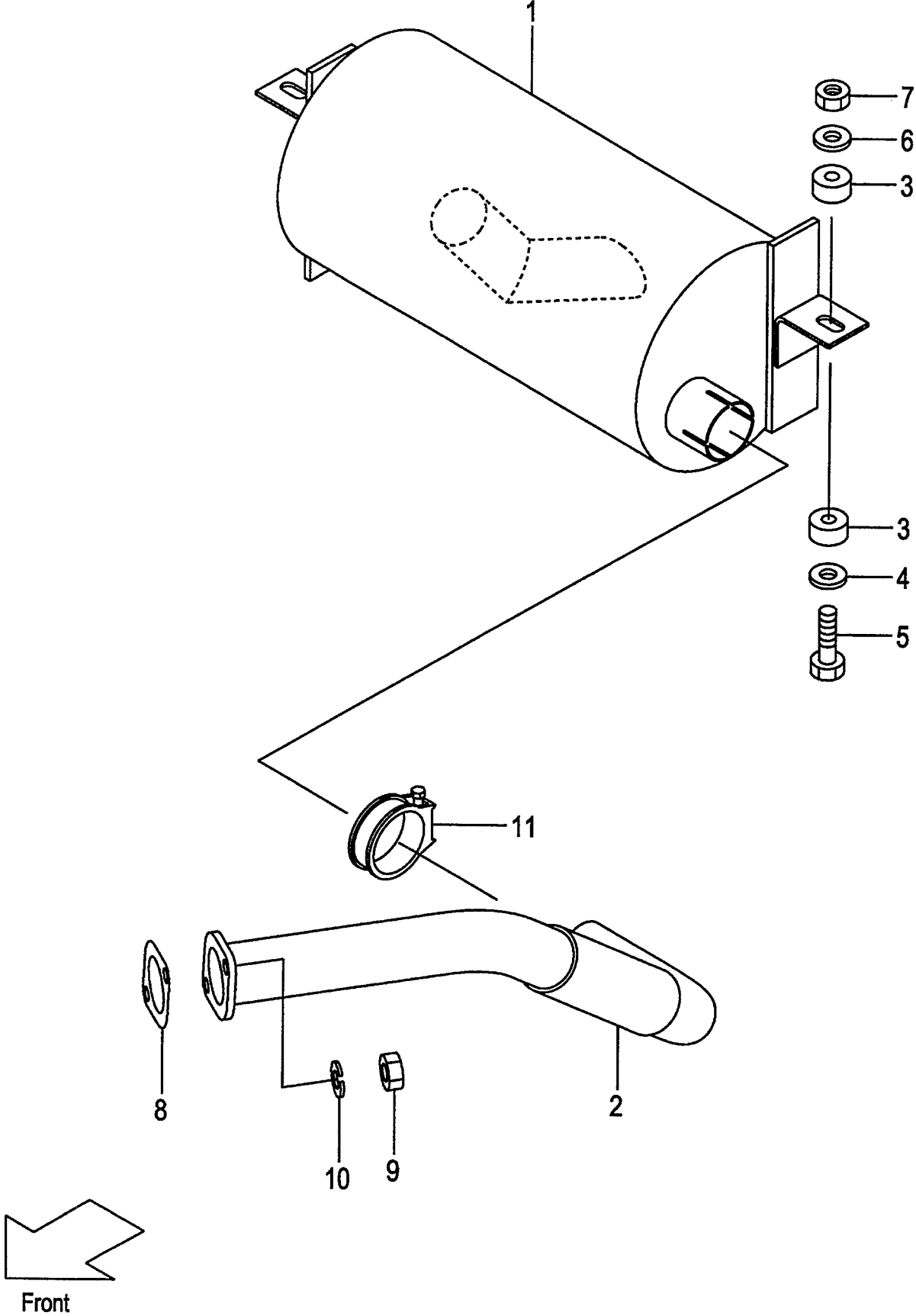
FIG.9 EXHAUST SYSTEM (F6042310) エキゾーストシステム
