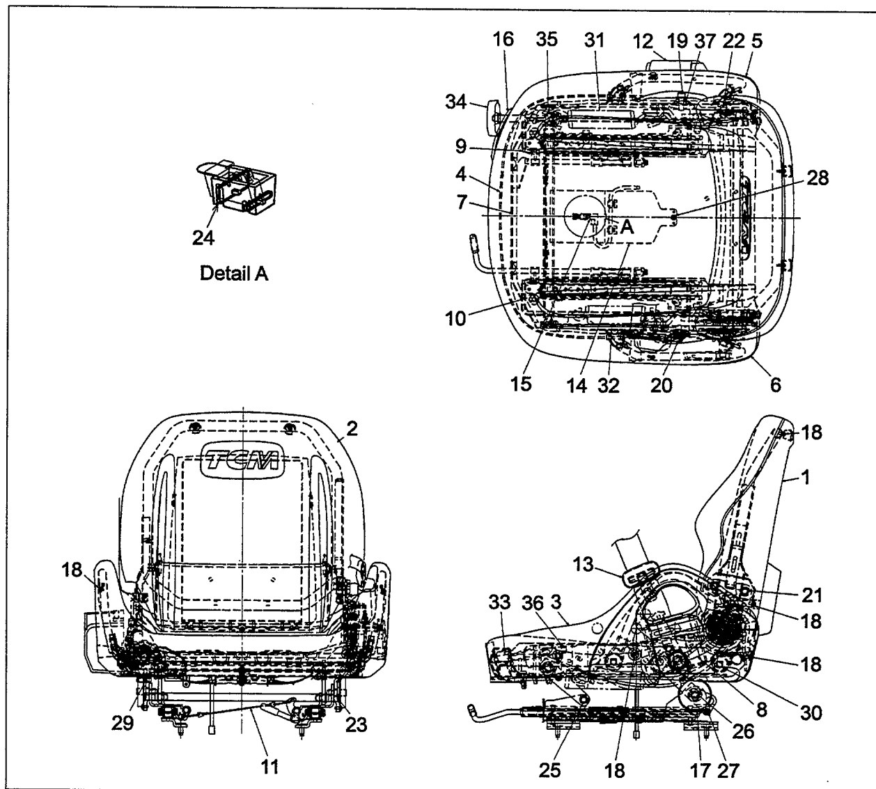
FIG.59 SEAT (F6046810) シート
