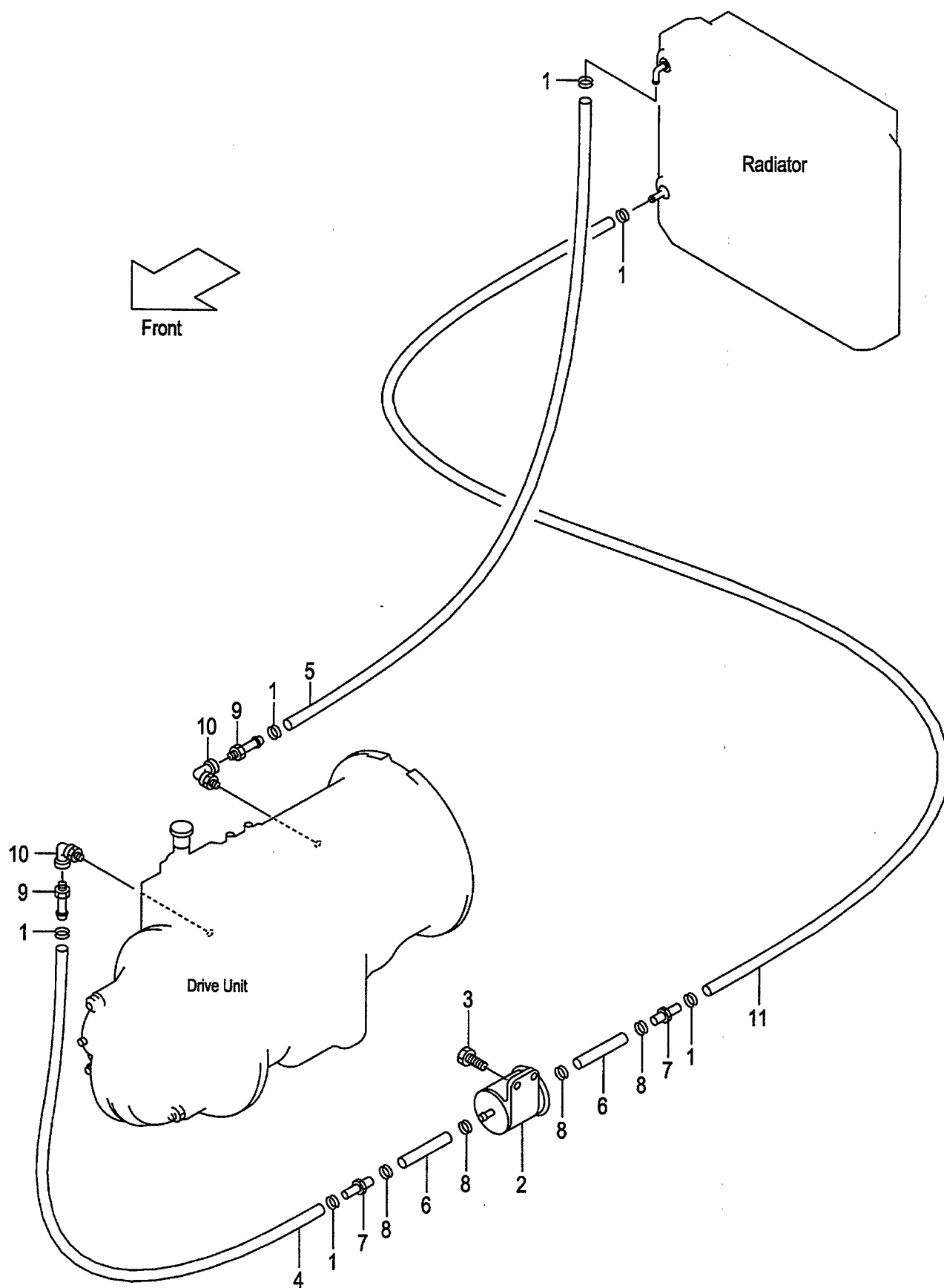
FIG.83 HYDRAULIC LINE(TOR-CON LINE) (F6047670) ハイドロリックライン
