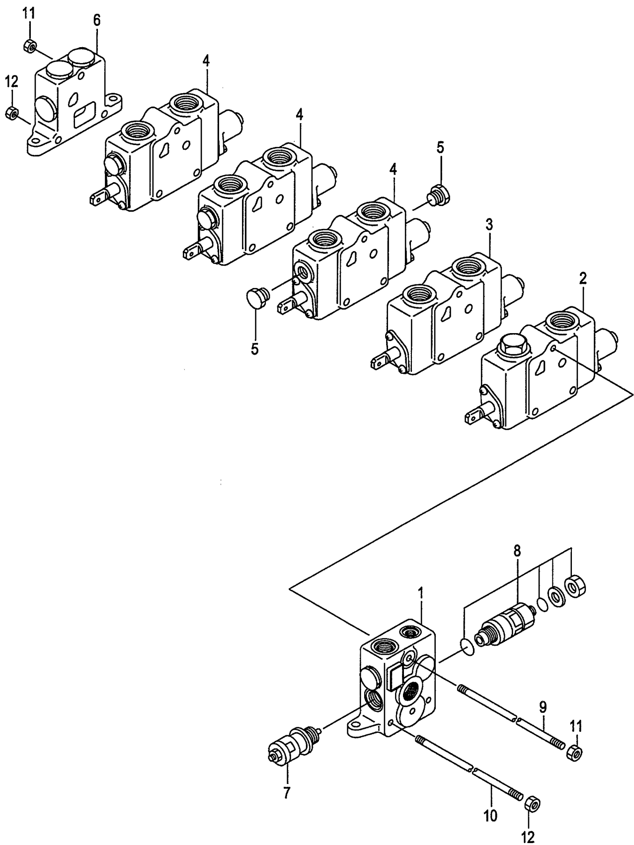
FIG.65 CONTROL VALVE [5SV] (F6047340) コントロールバルブ
