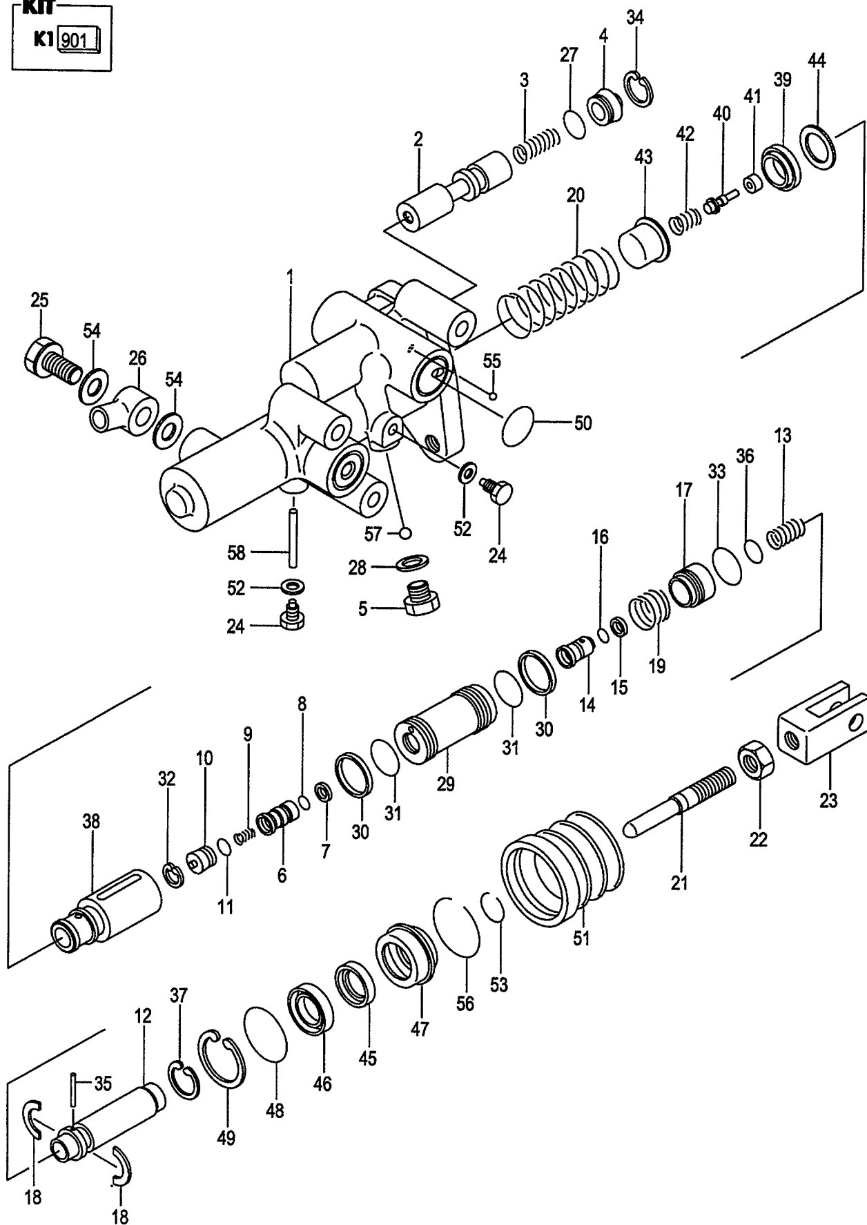
FIG.49 CLUTCH BOOSTER (CLUTCH) (F6045450) クラッチブースタ
