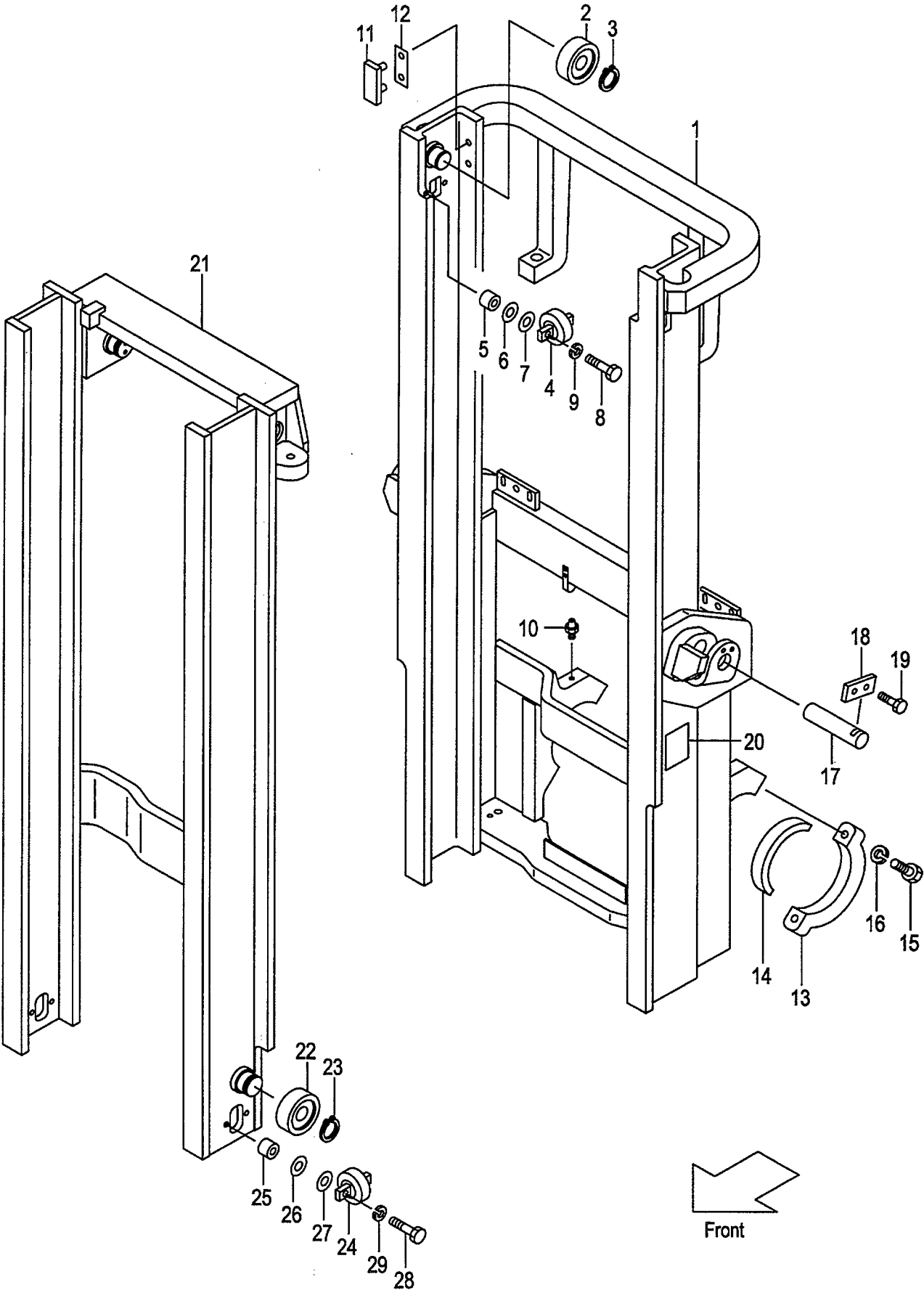
FIG.99 MAST [VM43F] (M6048330) マスト
