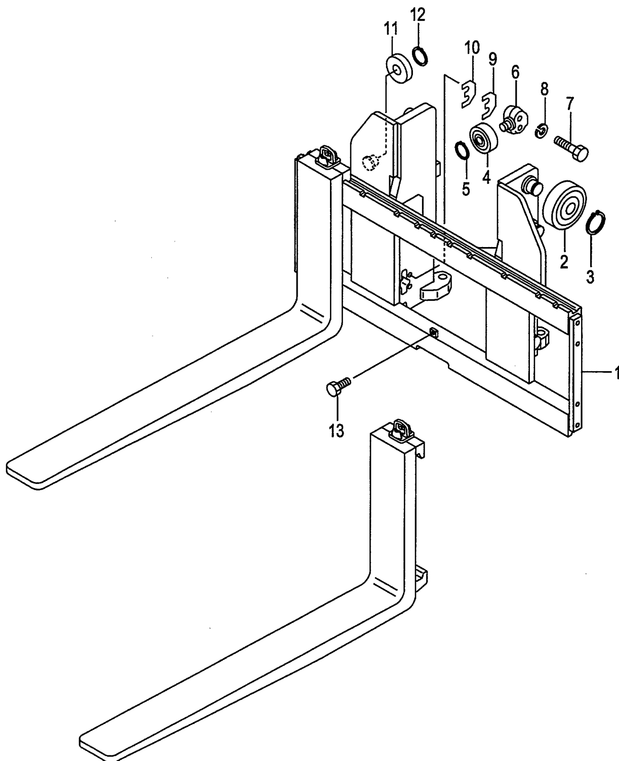
FIG.97 LIFT BRACKET [VM43F] (M6048230) リフトブラケット
