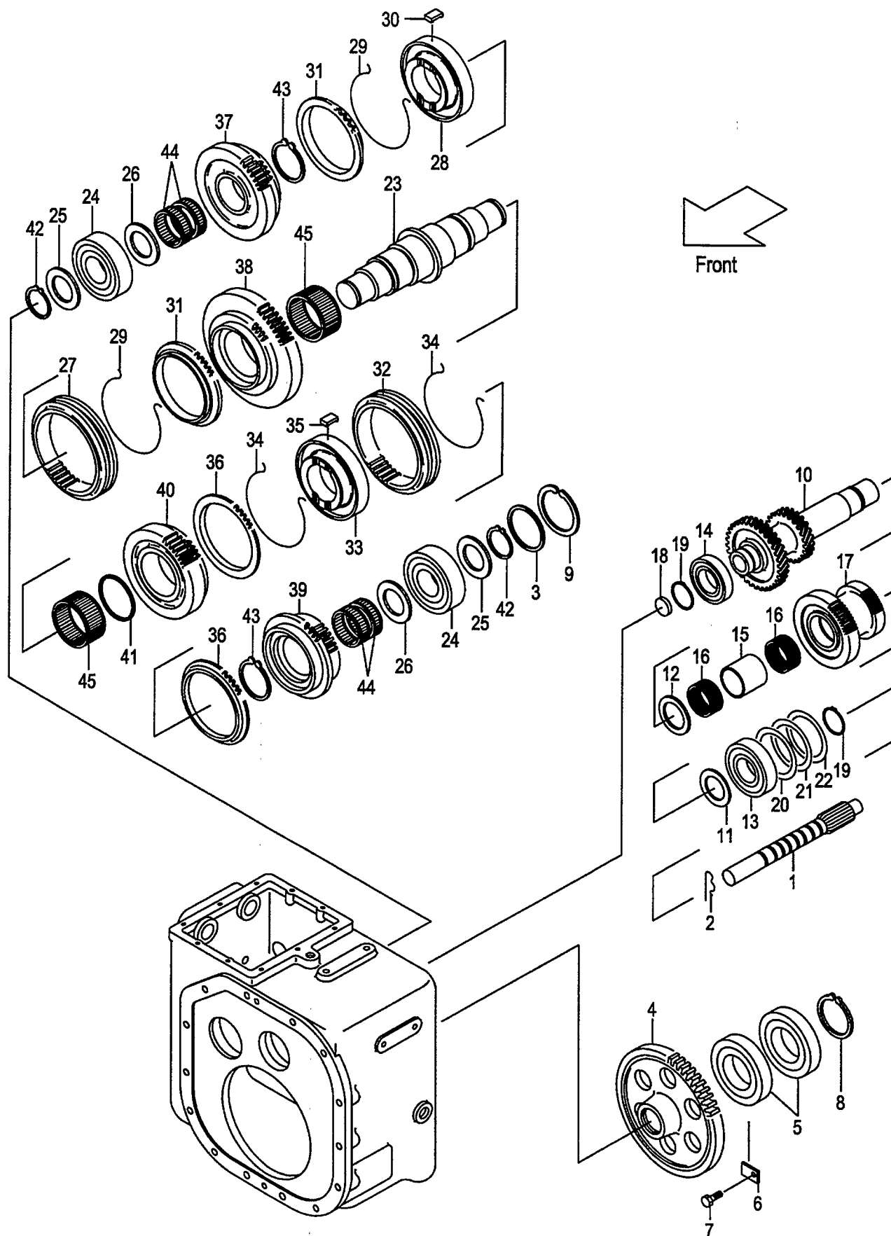
FIG.25 DRIVE UNIT (3/3)(CLUTCH) (F6042550) ドライブユニット
