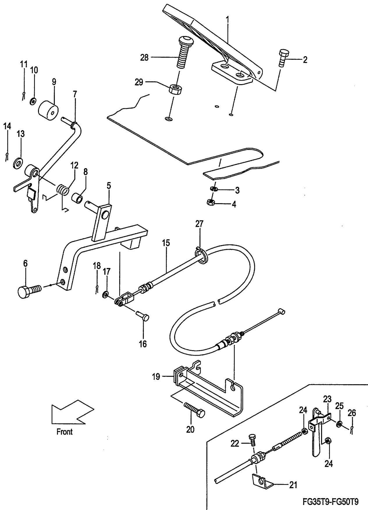
FIG.44 ACCEL PEDAL (F6045210) アクセルペダル
