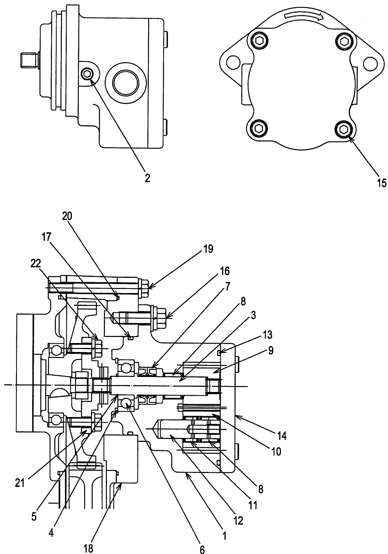
FIG.84 HYDRAULIC PUMP(CLUTCH) (F6047680) ハイ・ロリックポンプ°
