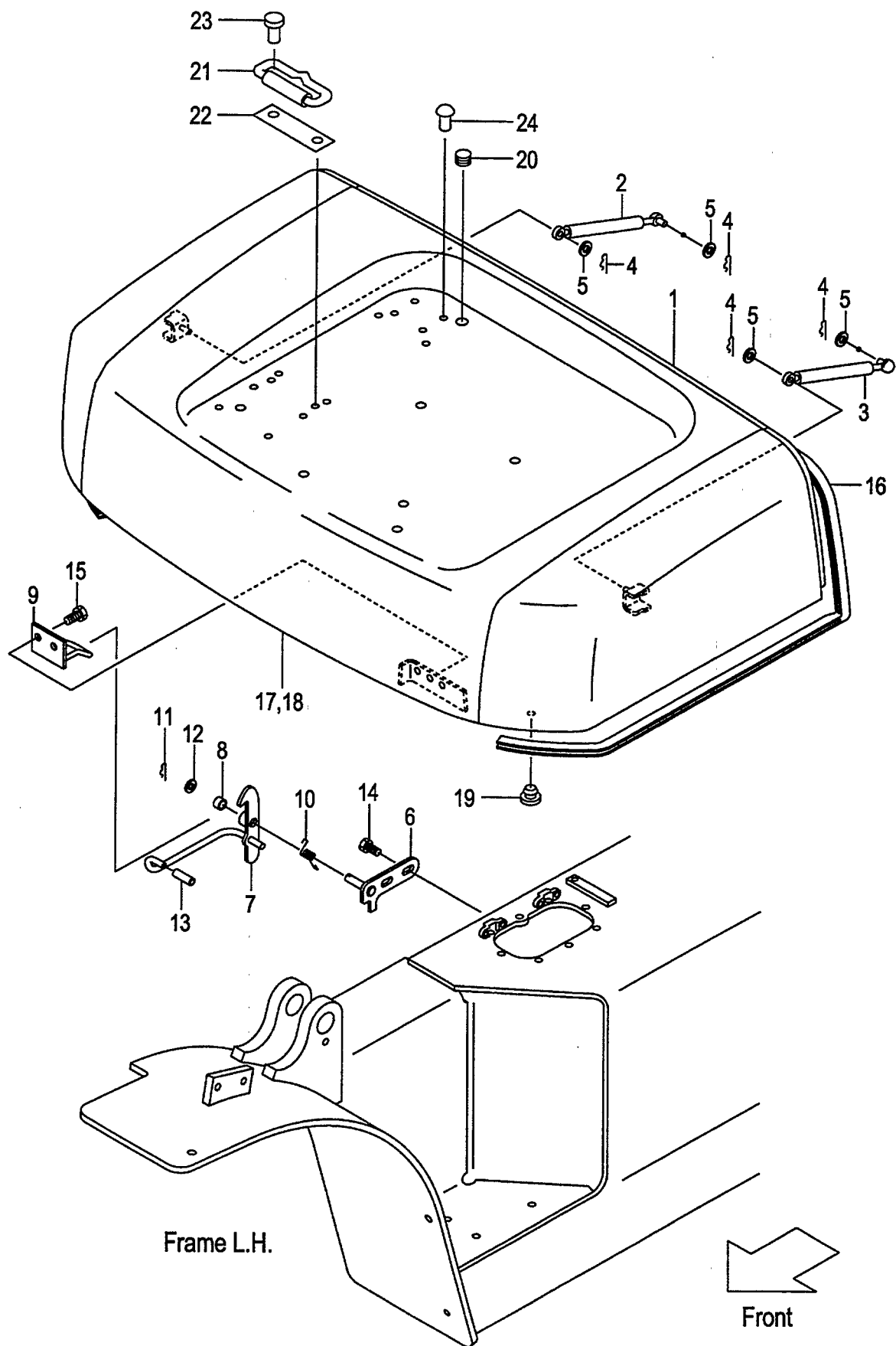
FIG.56 BONNET (F6046420) ホンネット
