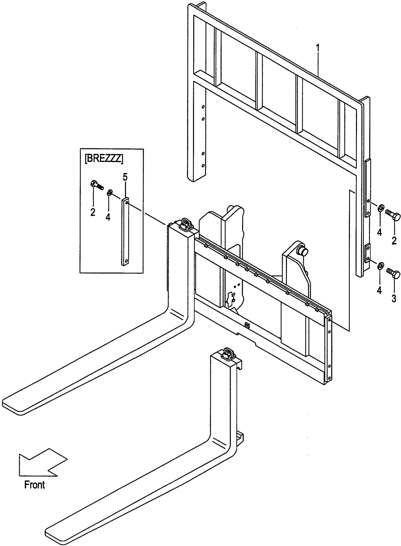
FIG.91 BACKREST [VM43A] (M6048220) バックレスト
