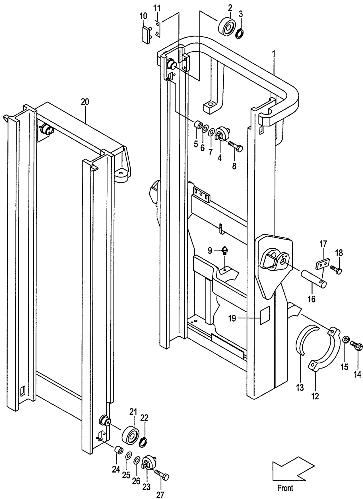
FIG.92 MAST [VM43A] (M6048310) マスト
