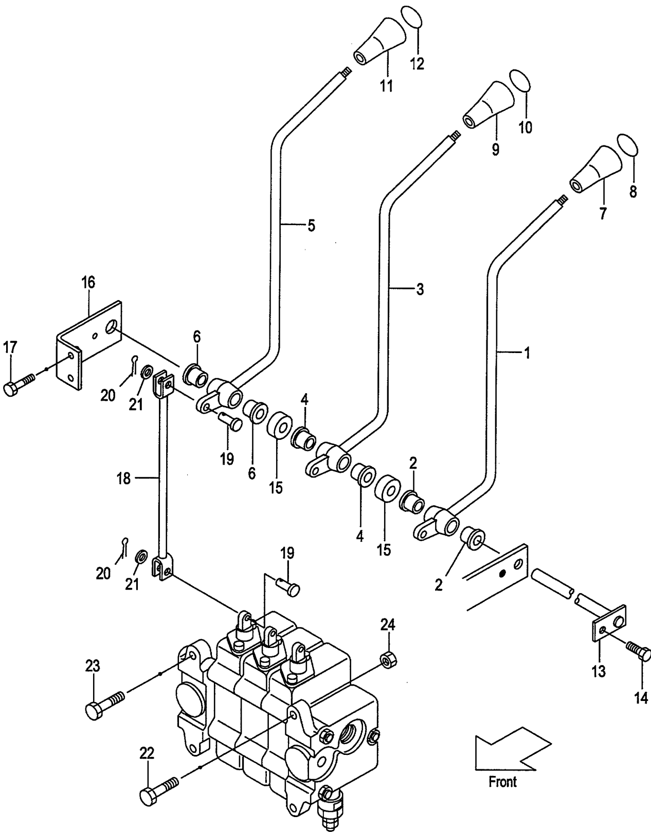
FIG.74 VALVE CONTROL [3SV] (F60473D0) バルブコントロール
