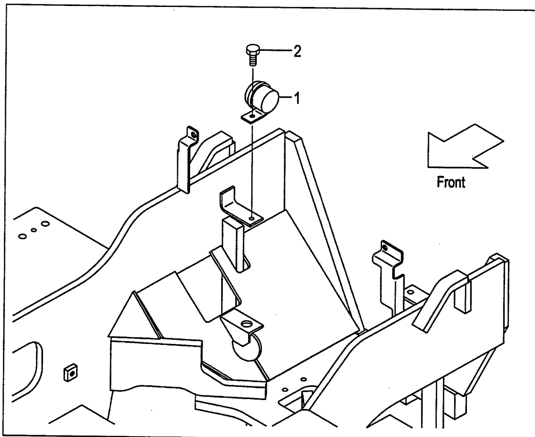
FIG.19 BACK BUZZER (F6042490) バックブザー
