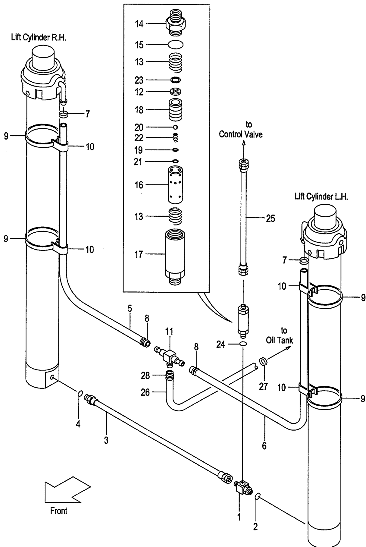
FIG.107 MAST PIPING [VM43H] (M6048460) マストパイピング
