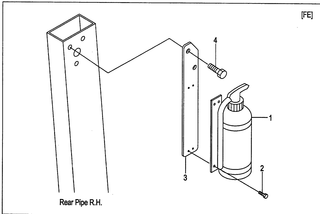
FIG.88 FIRE EXTINGUISHER [FE][FE/CAKB] (F6049320) ファイアクレンジングイッシャ
