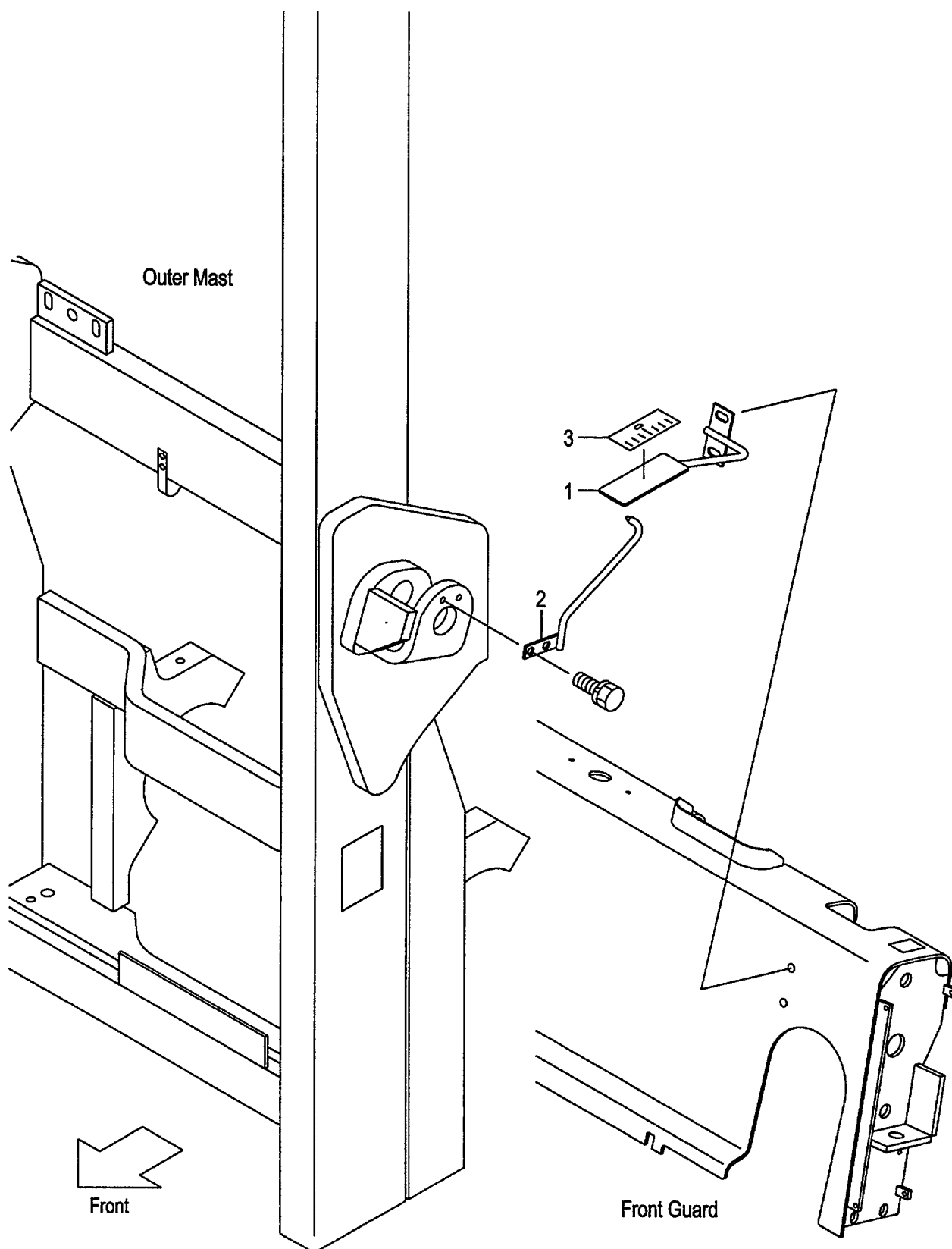
FIG.93 TILT GAUGE [TG/VM43A] (M6048320) ティルトゲージ
