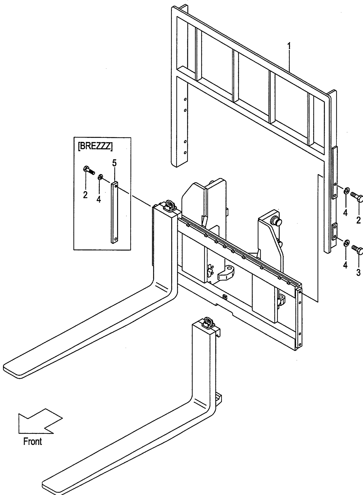
FIG.98 BACKREST [VM43F] (M6048240) バックレスト
