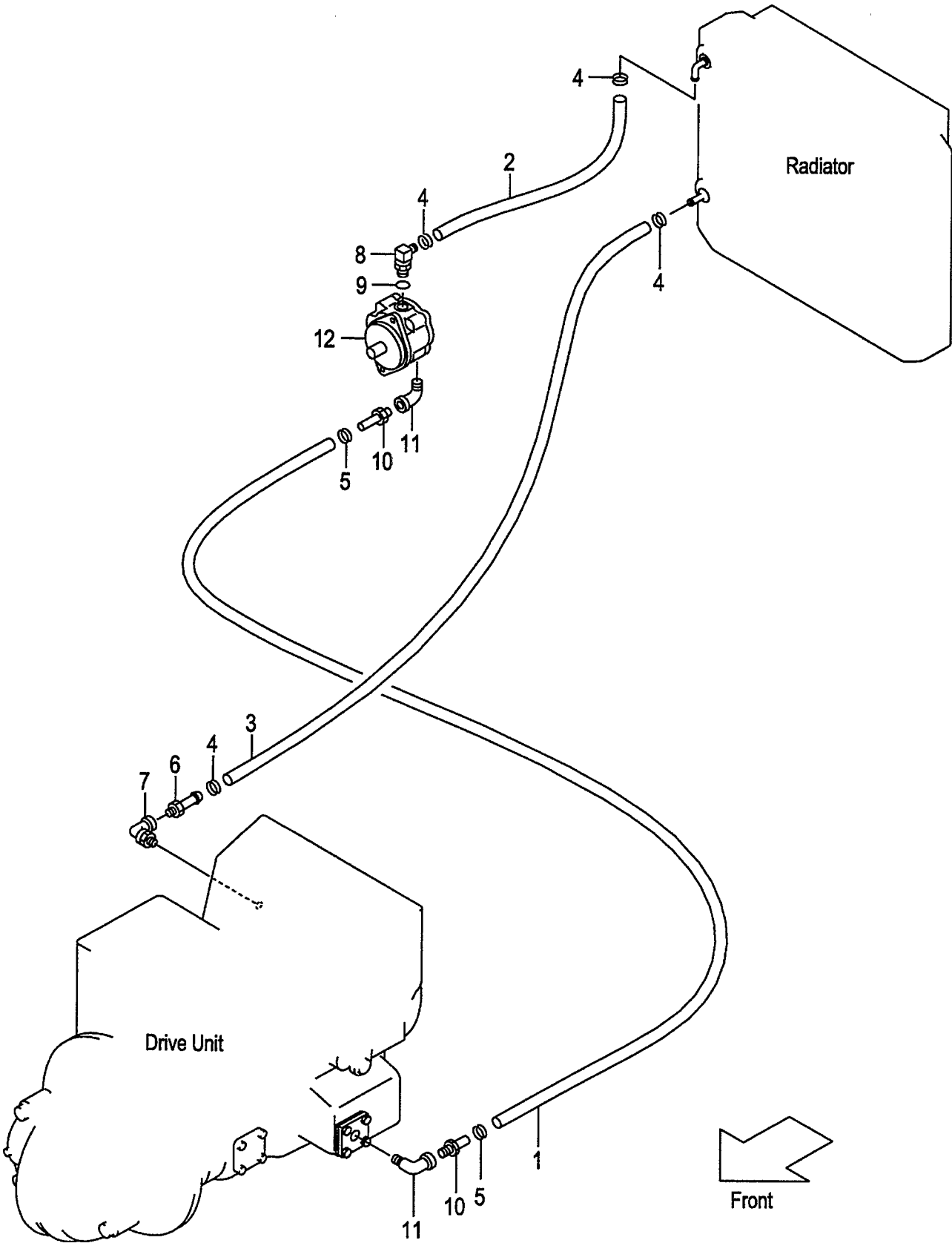
FIG.82 HYDRAULIC LINE(CLUTCH LINE) (F6047660) ハイドロリックライン
