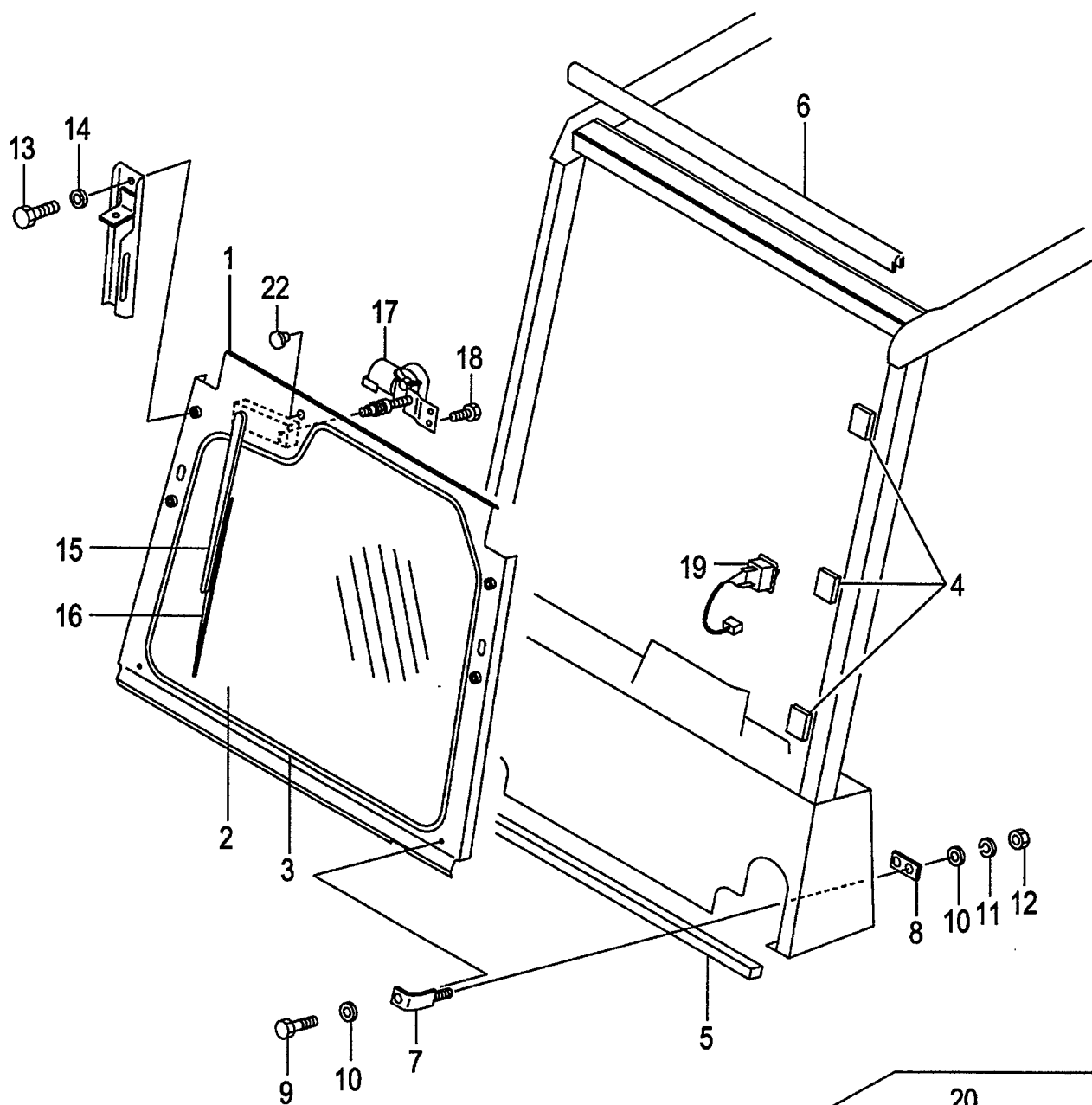
FIG.87 FRONT GLASS [AW071][AW061] (F6049310) フロントガラス
