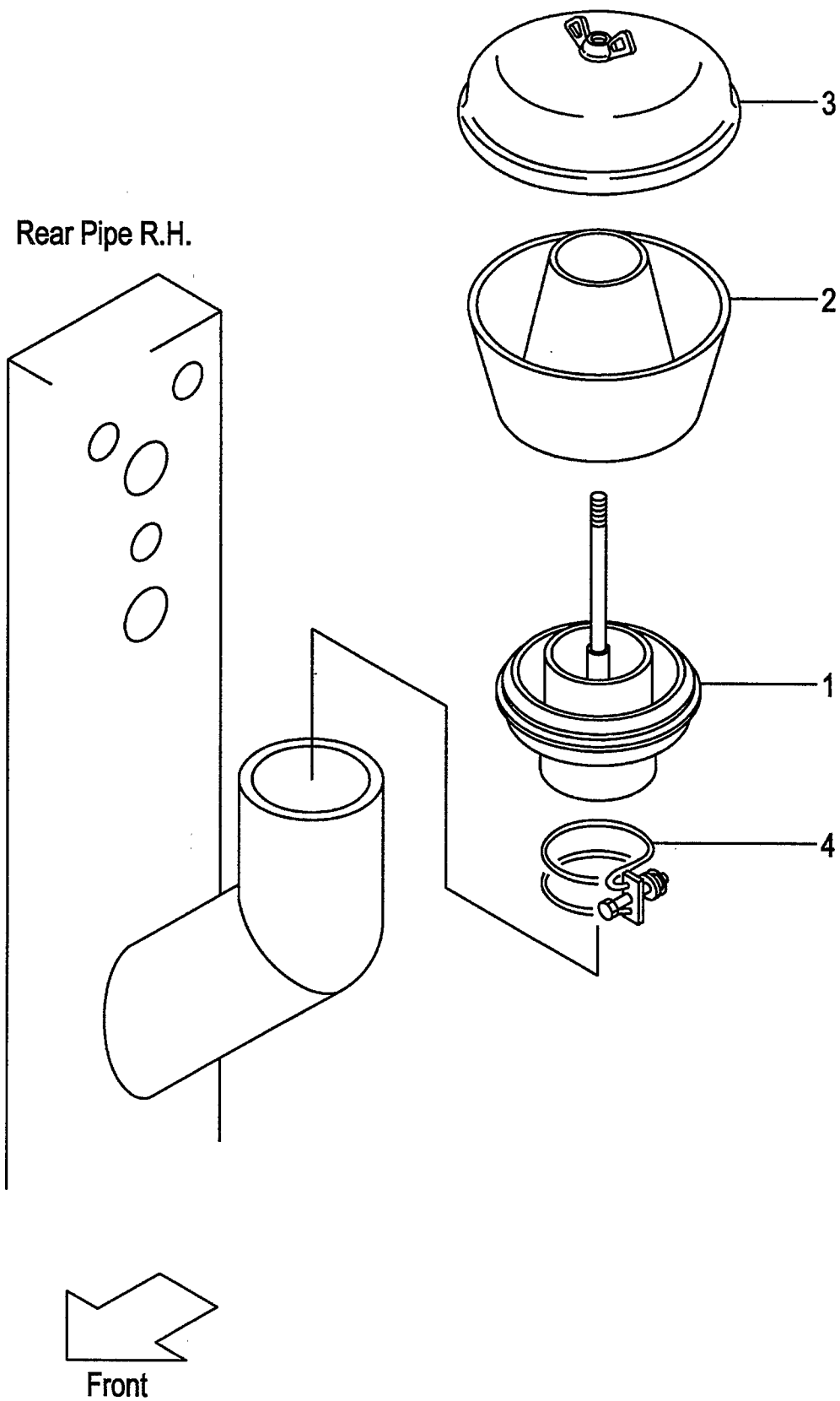
FIG.4 PRE CLEANER [CAKB] (F6041040) プレクリーナ
