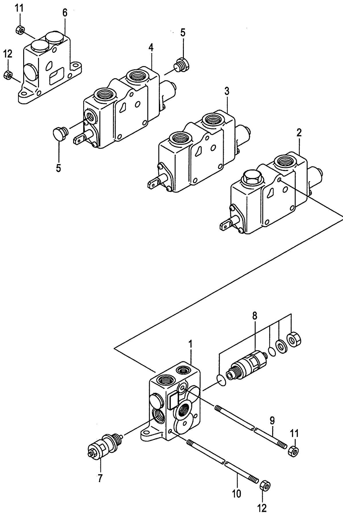
FIG.63 CONTROL VALVE [3SV] (F6047320) コントロールバルブ
