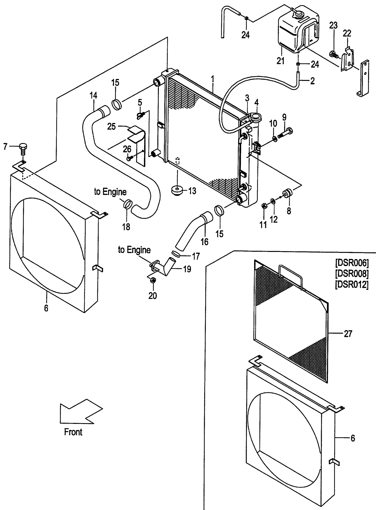
FIG.6 COOLING UNIT (F6042120) クーリングユニット
