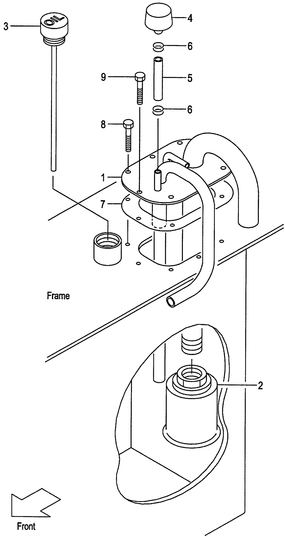
FIG.52 OIL TANK (F6046120) オイルタンク
