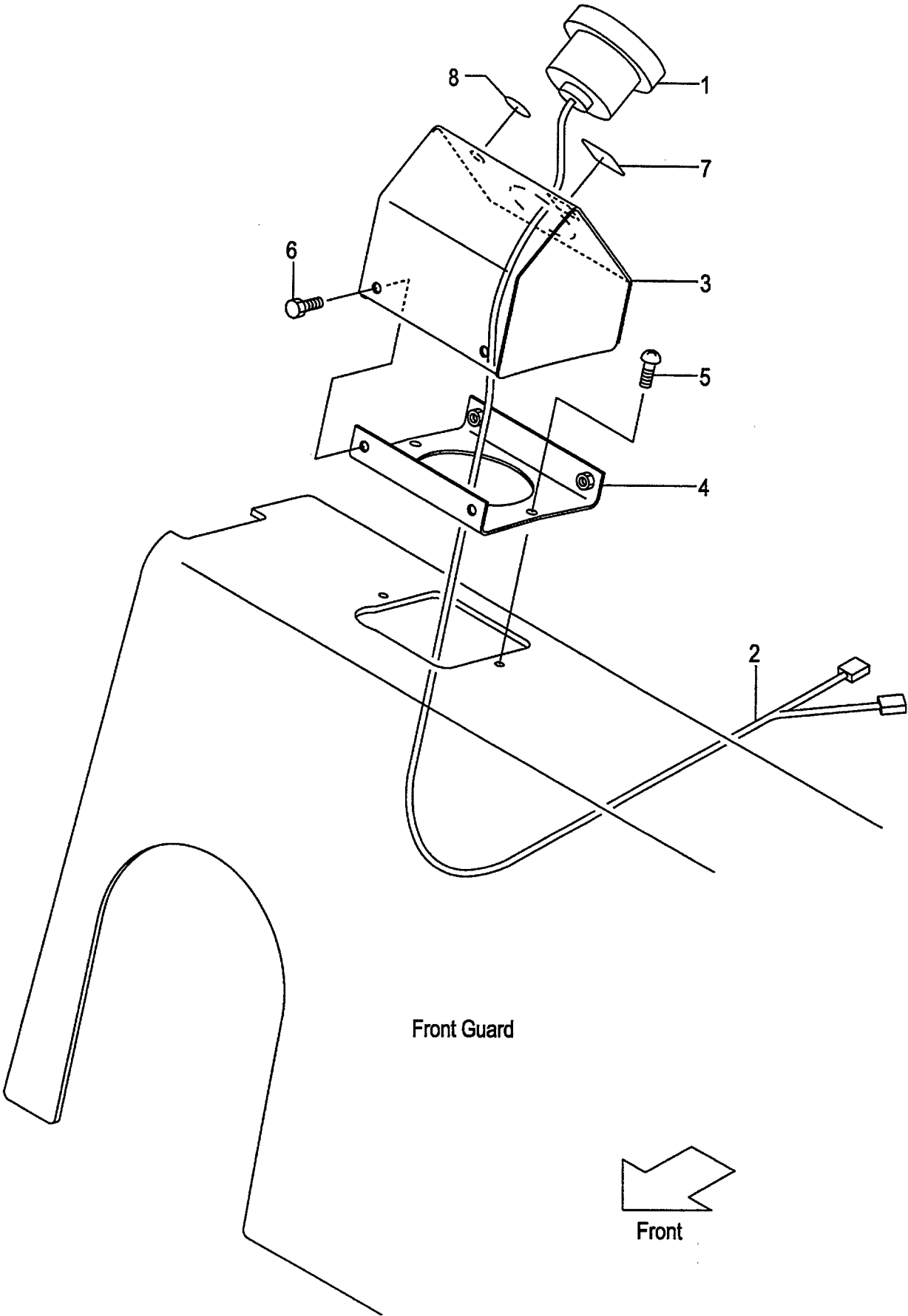
FIG.20 AMMETER [AM] (F60424A0) アンメータ
